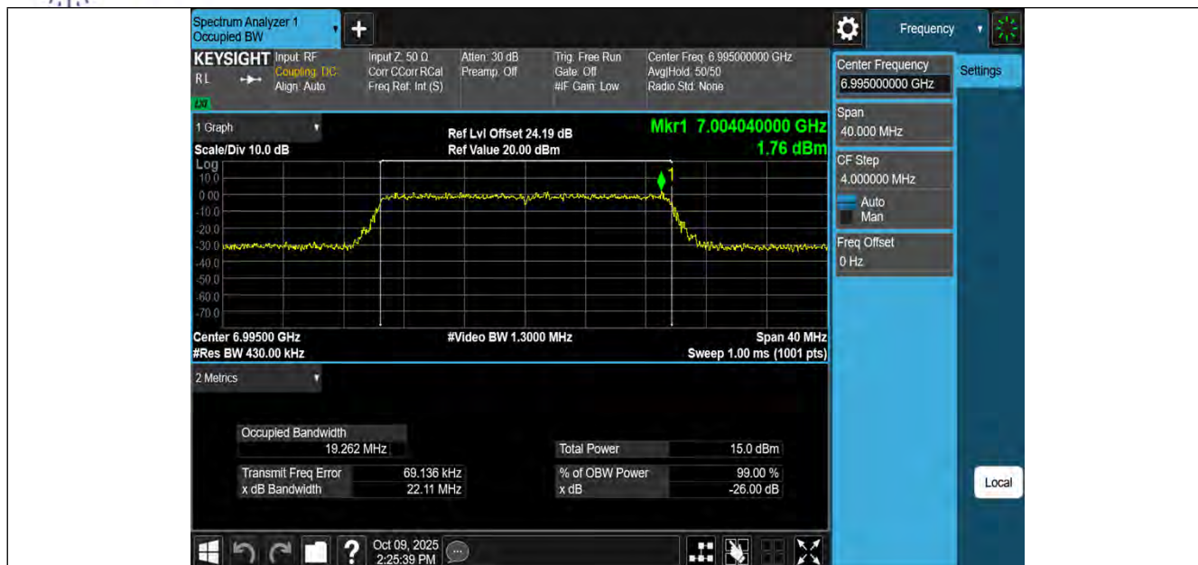
11AX20MIMO-Ant1-6995-PASS
