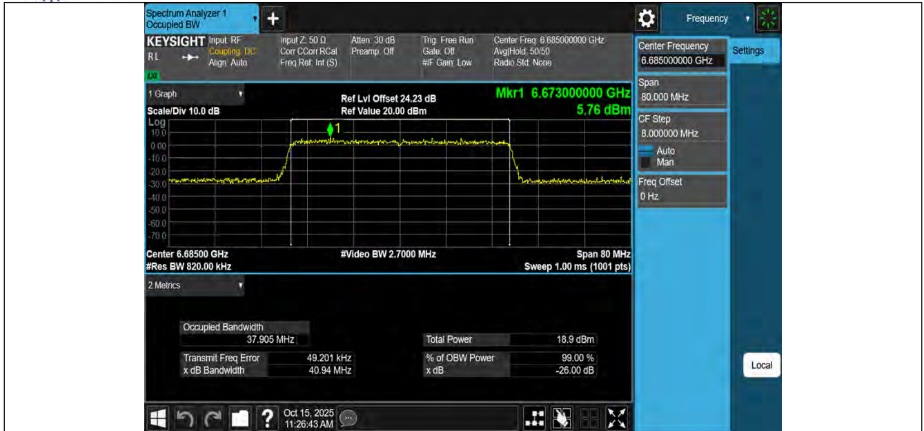
11AX40MIMO-Ant3-6685-PASS
