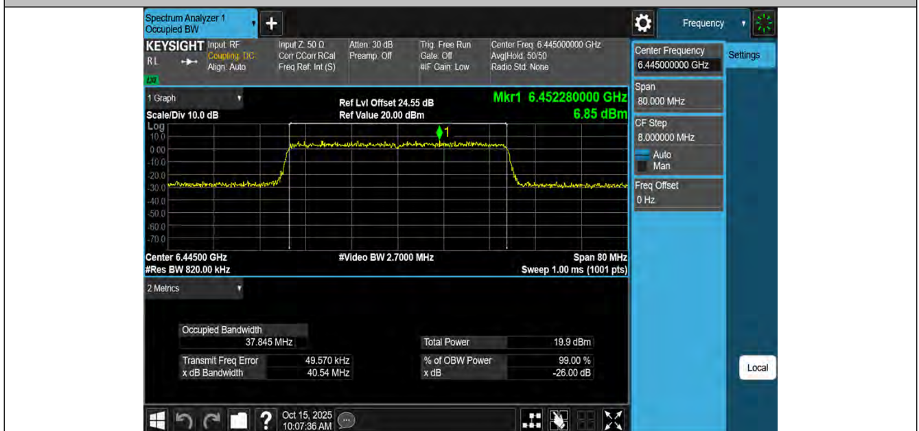
11AX40MIMO-Ant4-6445-PASS
