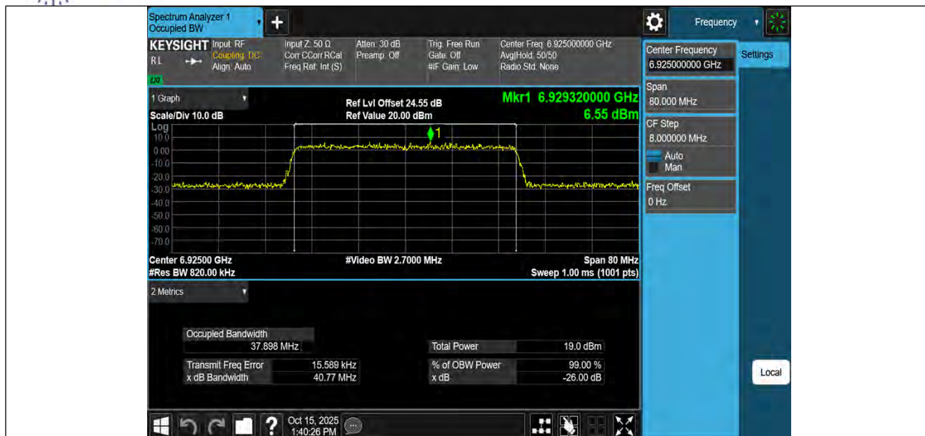
11AX40MIMO-Ant3-6925-PASS
