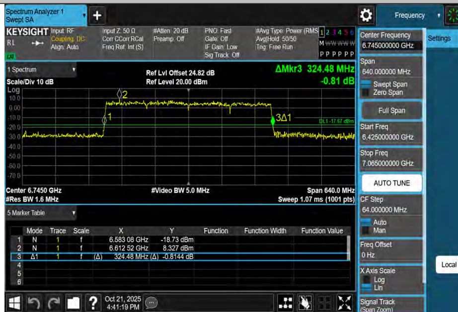
11BE320MIMO-Ant4-6745
