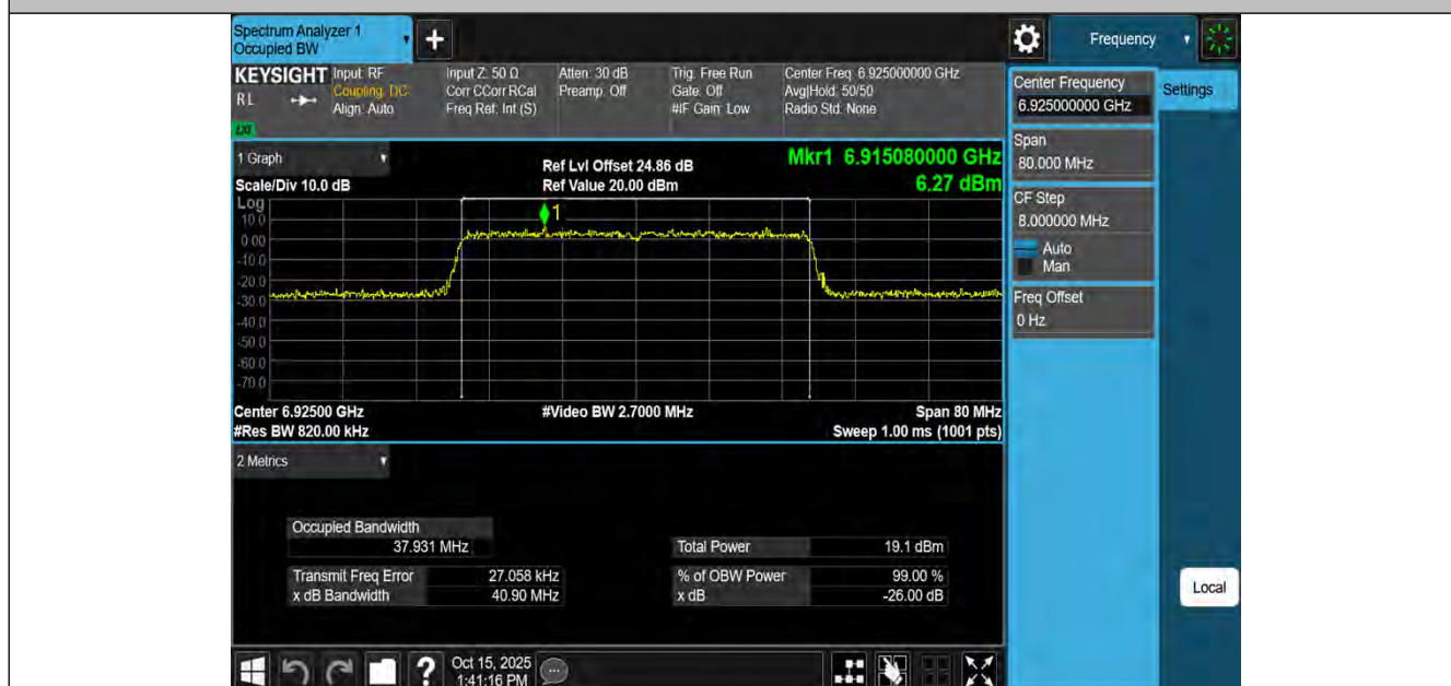
11AX40MIMO-Ant4-6925-PASS
