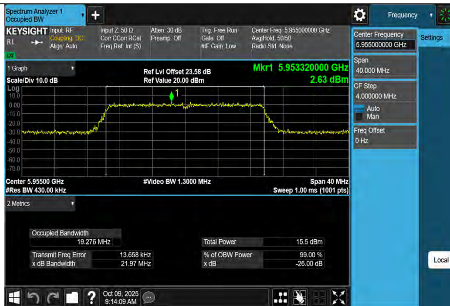
11AX20MIMO-Ant1-5955-PASS
