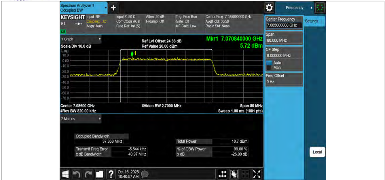
11AX40MIMO-Ant3-7085-PASS
