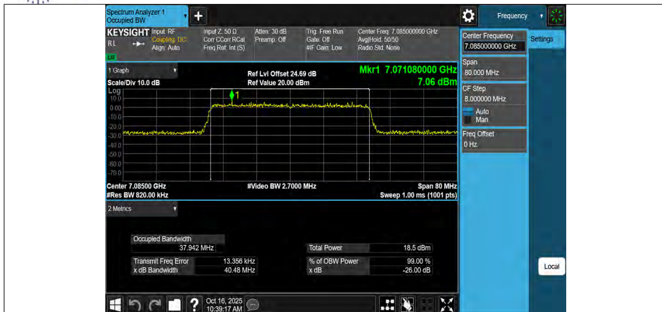
11AX40MIMO-Ant1-7085-PASS
