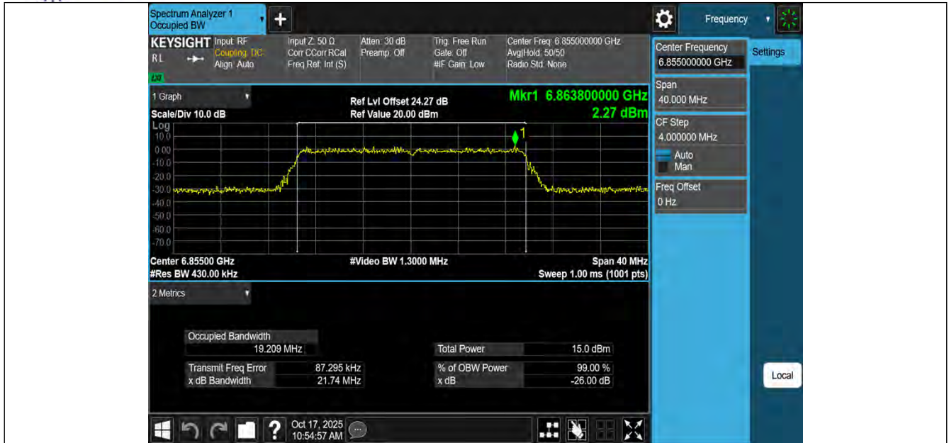
11BE20MIMO-Ant1-6855-PASS
