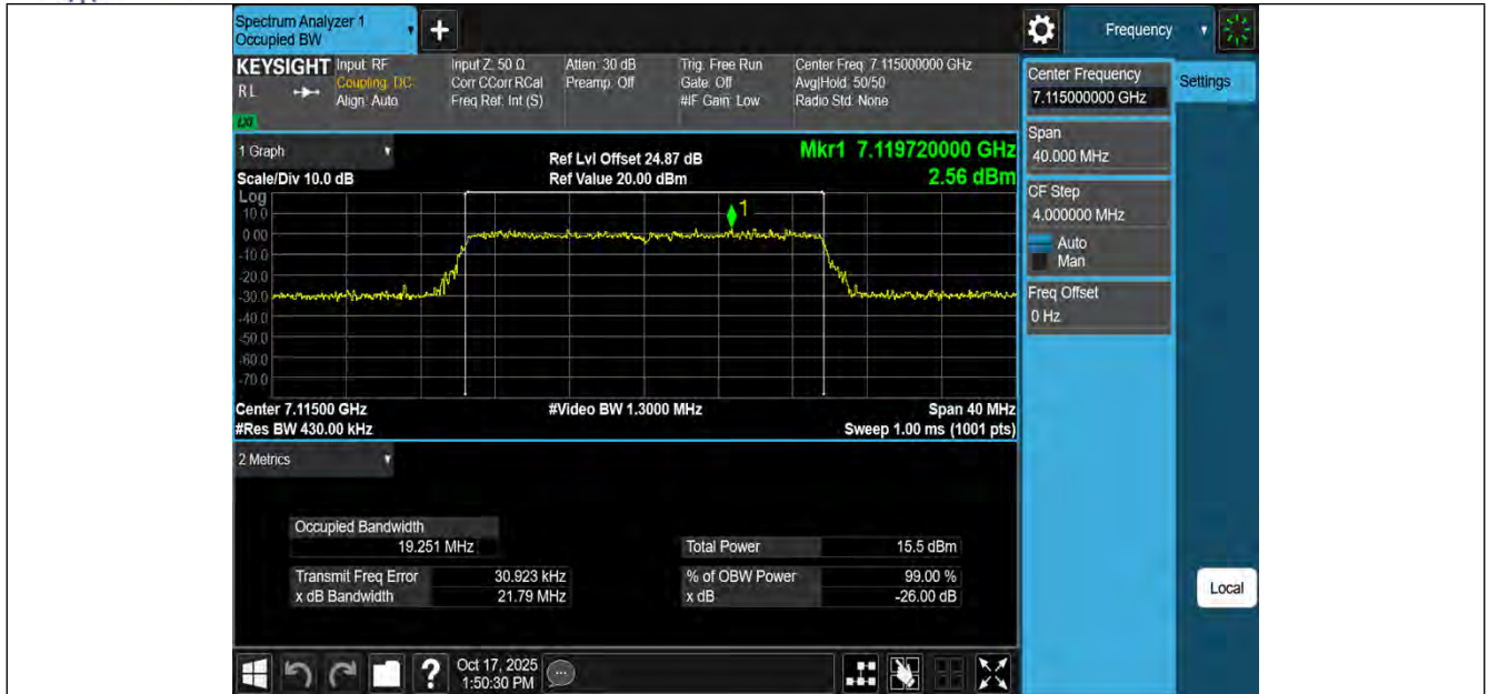
11BE20MIMO-Ant1-7115-PASS
