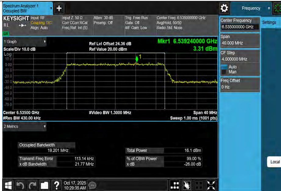
11BE20MIMO-Ant1-6535-PASS
