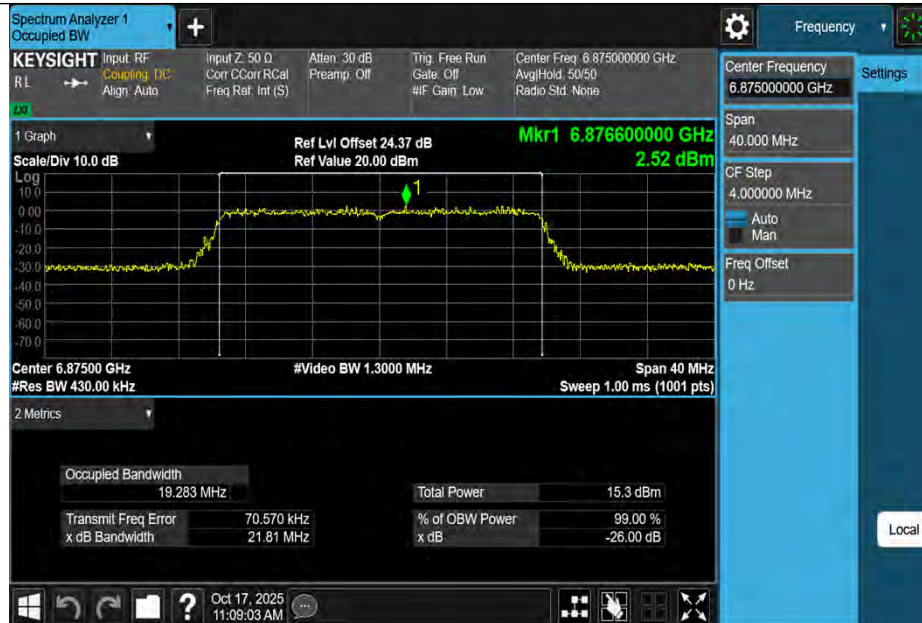
11BE20MIMO-Ant1-6875-PASS
