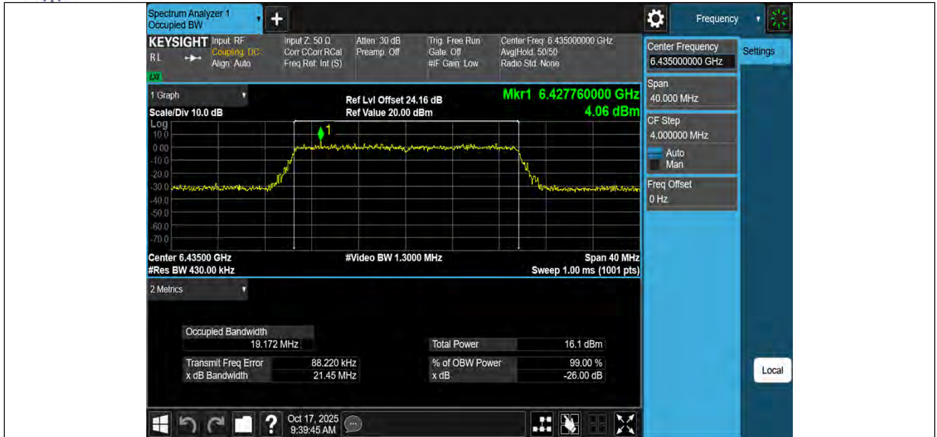
11BE20MIMO-Ant1-6435-PASS
