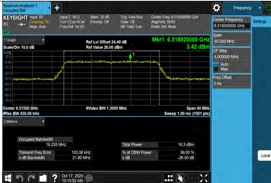
11BE20MIMO-Ant1-6515-PASS
