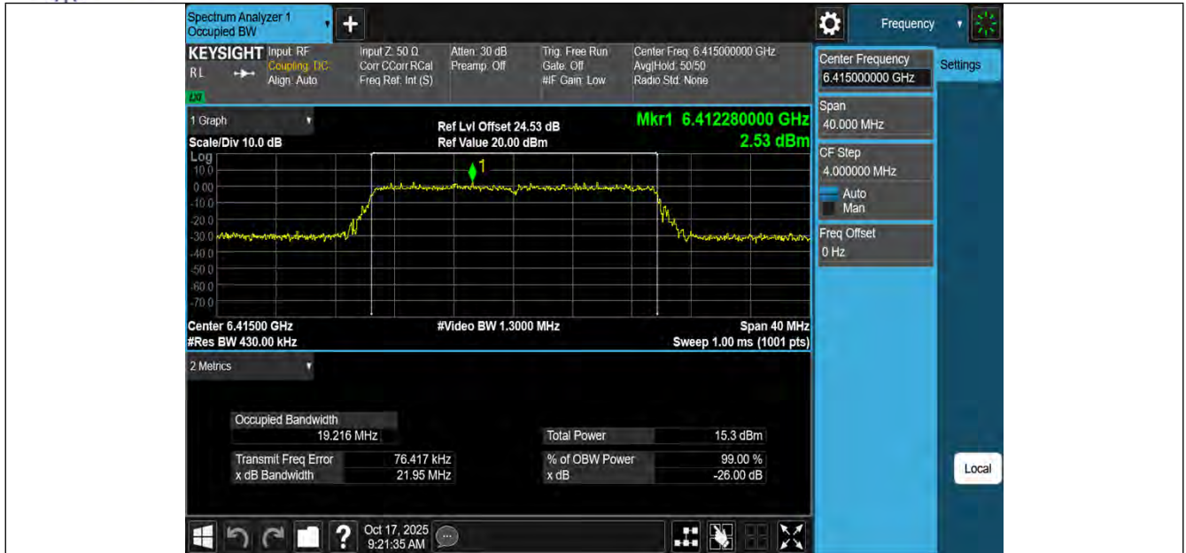
11BE20MIMO-Ant1-6415-PASS
