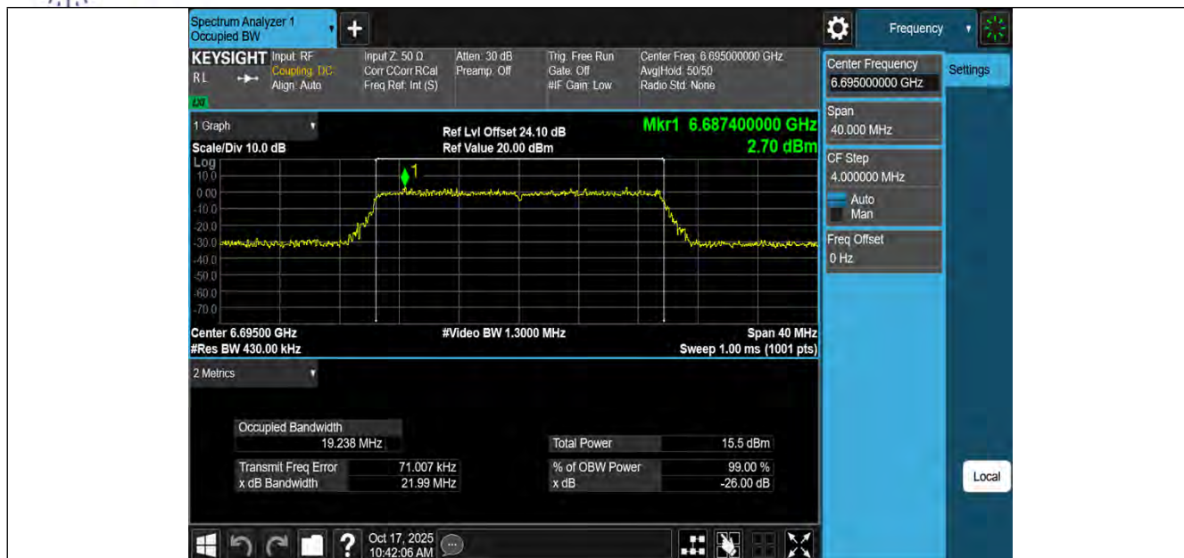
11BE20MIMO-Ant1-6695-PASS
