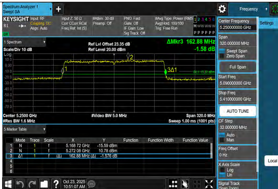
11BE160MIMO-Ant1-5250
