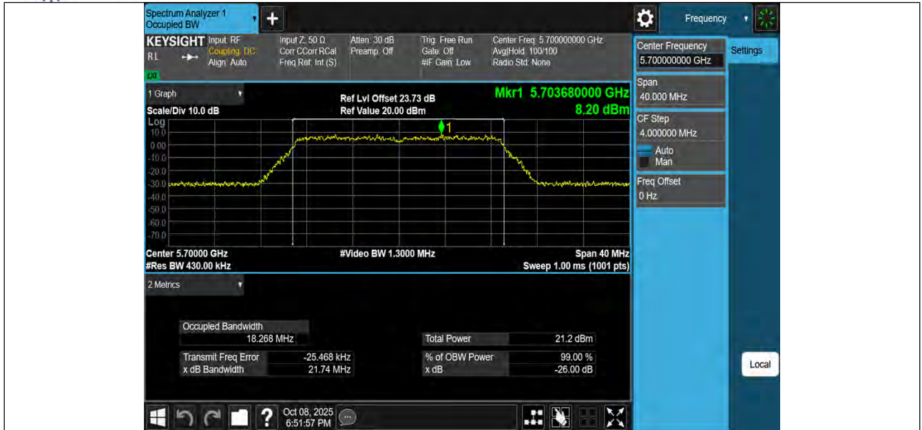
11N20MIMO-Ant3-5700
