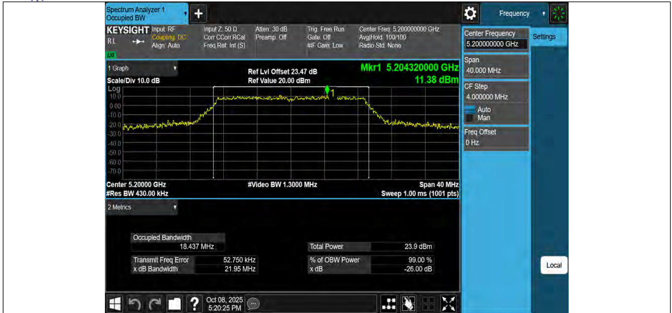
11N20MIMO-Ant3-5200
