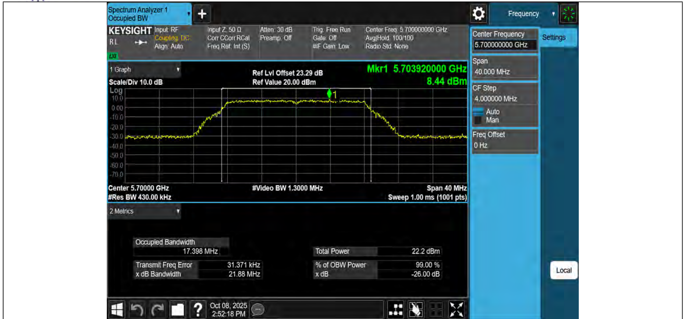
11A-Ant1-5700
