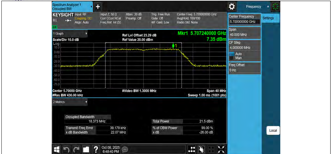
11N20MIMO-Ant1-5700
