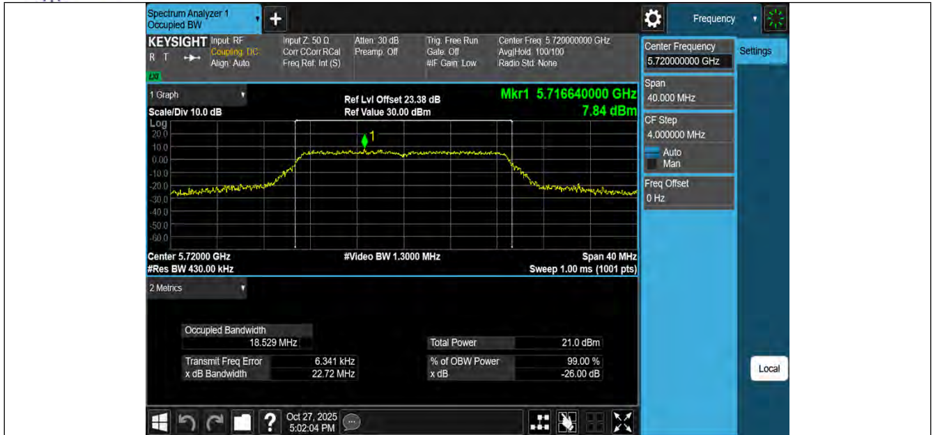
11N20MIMO-Ant1-5720
