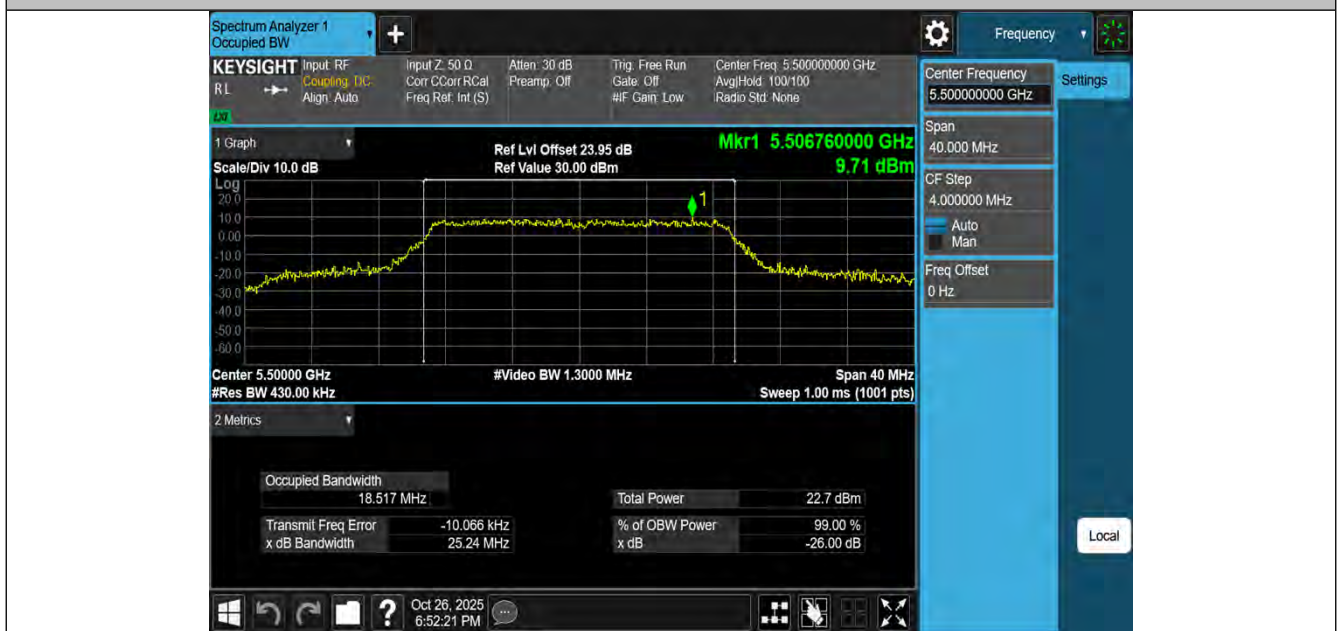
11N20MIMO-Ant4-5500
