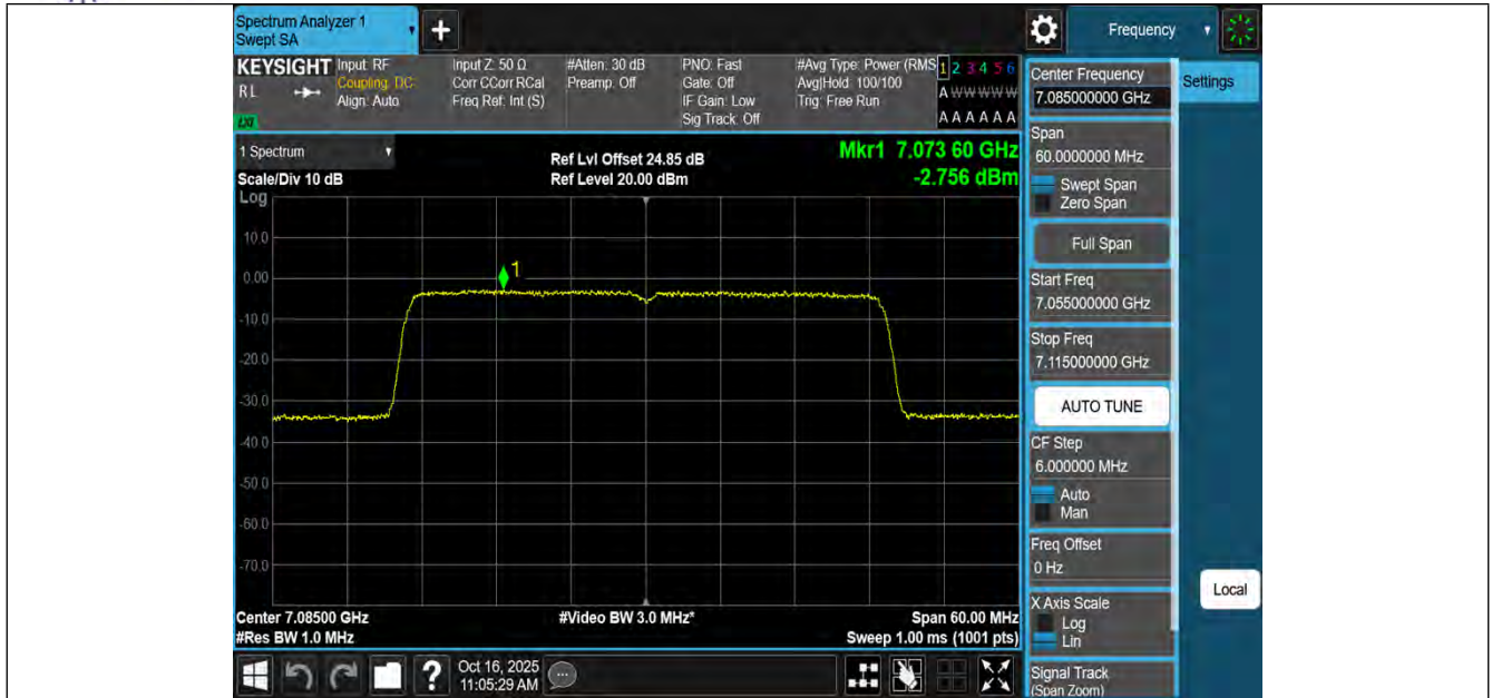
11AX40MIMO-Ant1-7085-PASS
