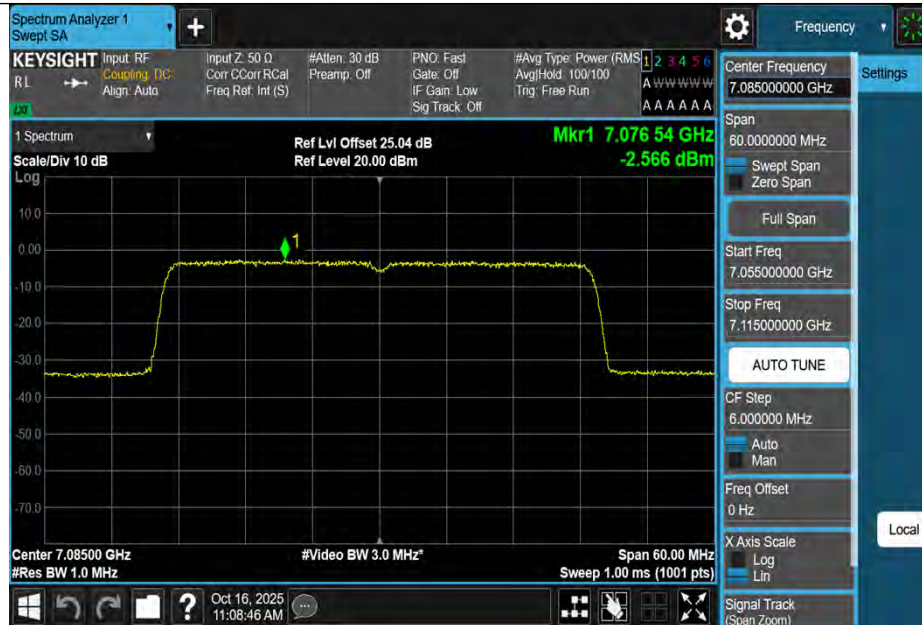
11AX40MIMO-Ant3-7085-PASS
