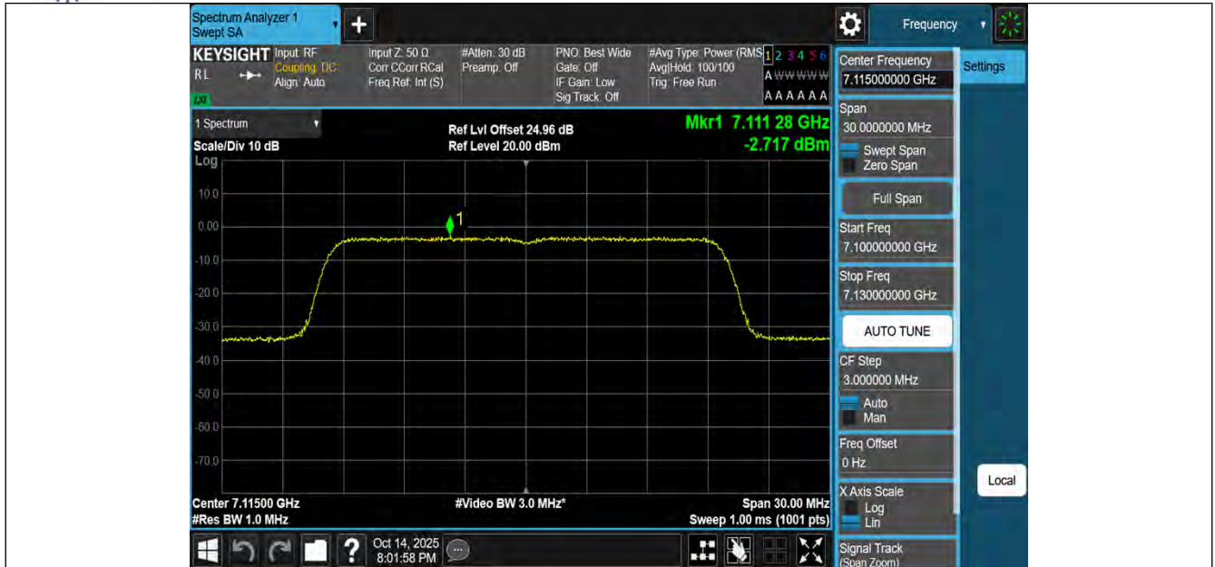
11AX20MIMO-Ant1-7115-PASS
