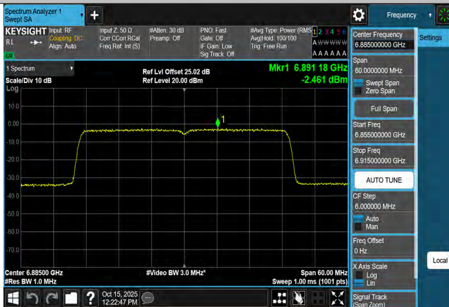
11AX40MIMO-Ant4-6885-PASS
