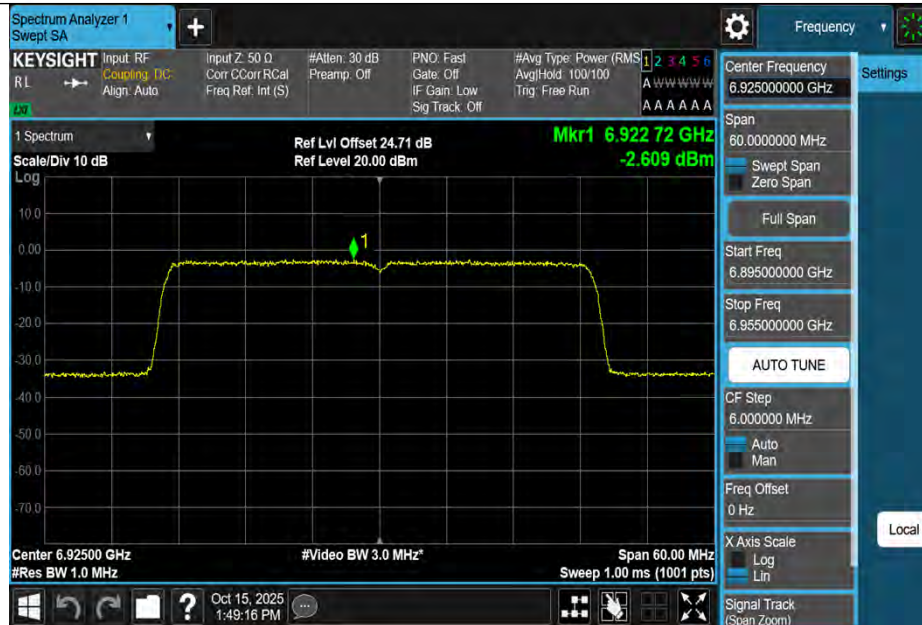
11AX40MIMO-Ant3-6925-PASS
