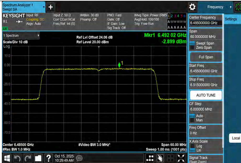
11AX40MIMO-Ant1-6485-PASS
