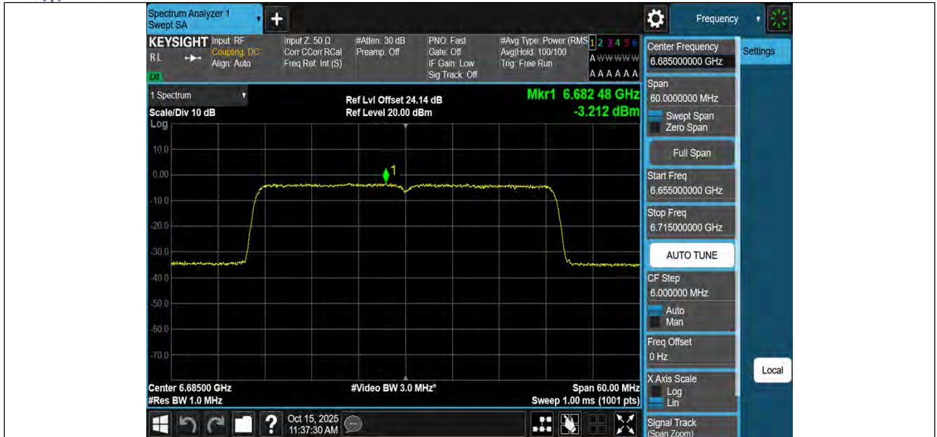
11AX40MIMO-Ant1-6685-PASS
