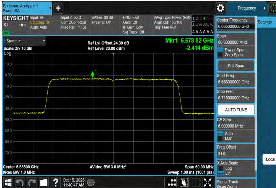
11AX40MIMO-Ant3-6685-PASS
