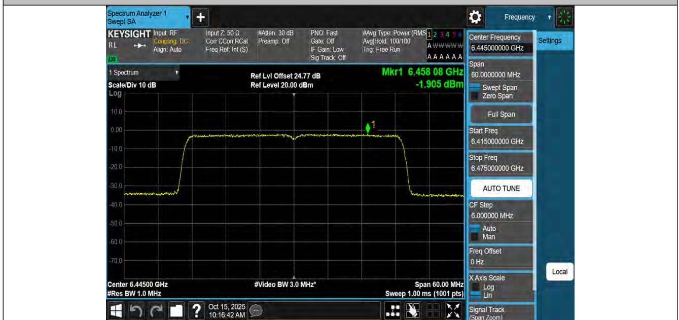
11AX40MIMO-Ant4-6445-PASS
