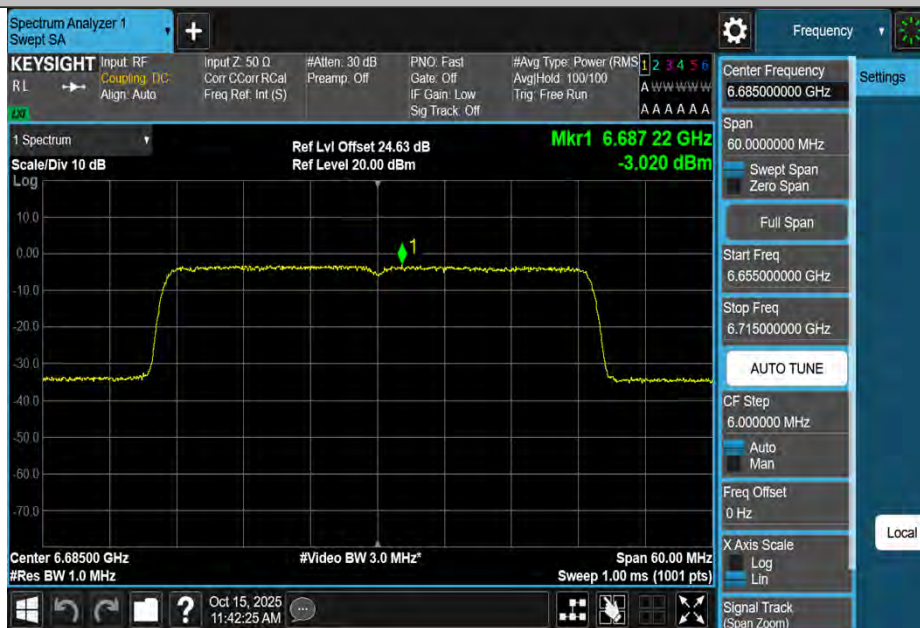
11AX40MIMO-Ant4-6685-PASS
