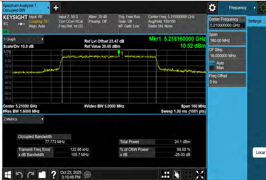
11AX80MIMO-Ant3-5210
