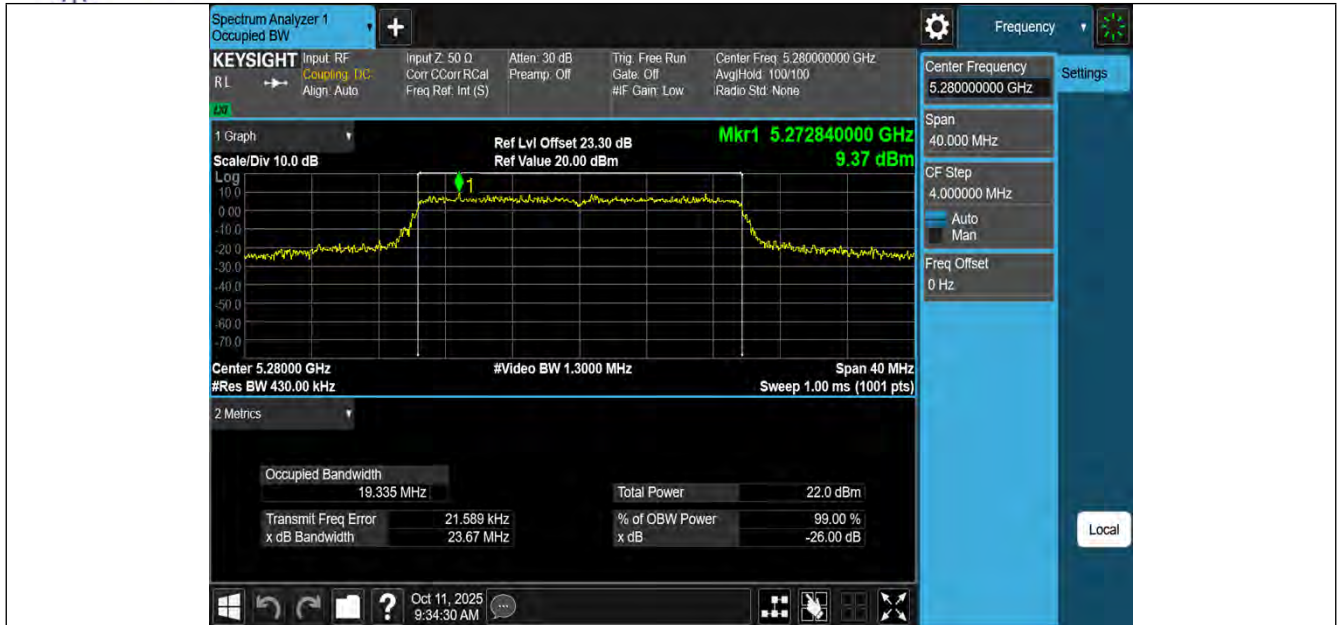
11AX20MIMO-Ant1-5280
