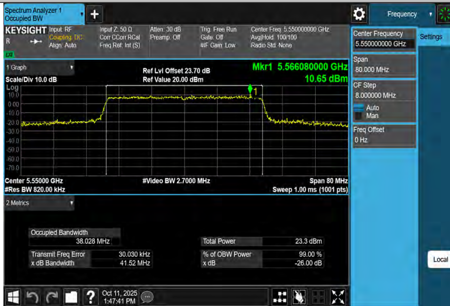
11AX40MIMO-Ant4-5550
