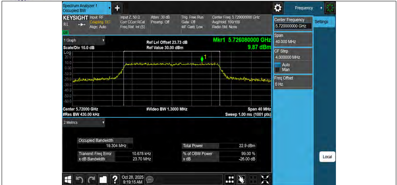
11AX20MIMO-Ant3-5720
