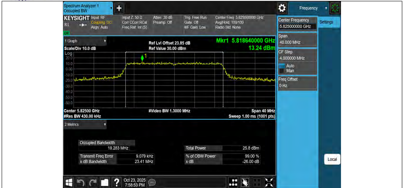
11AX20MIMO-Ant3-5825
