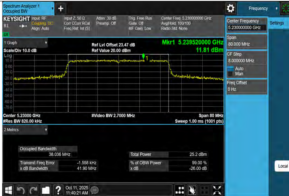
11AX40MIMO-Ant3-5230
