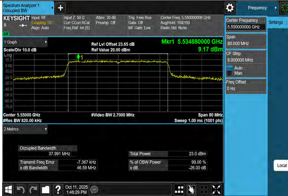
11AX40MIMO-Ant3-5550
