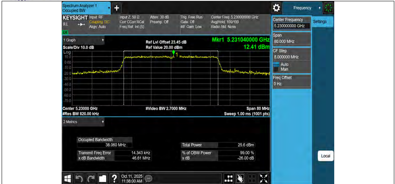
11AX40MIMO-Ant1-5230
