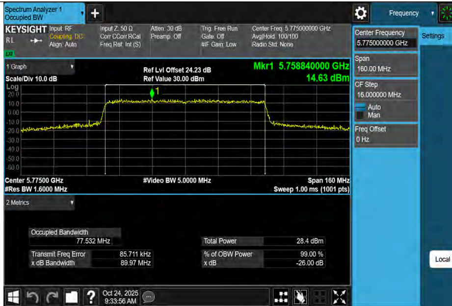
11AX80MIMO-Ant3-5775
