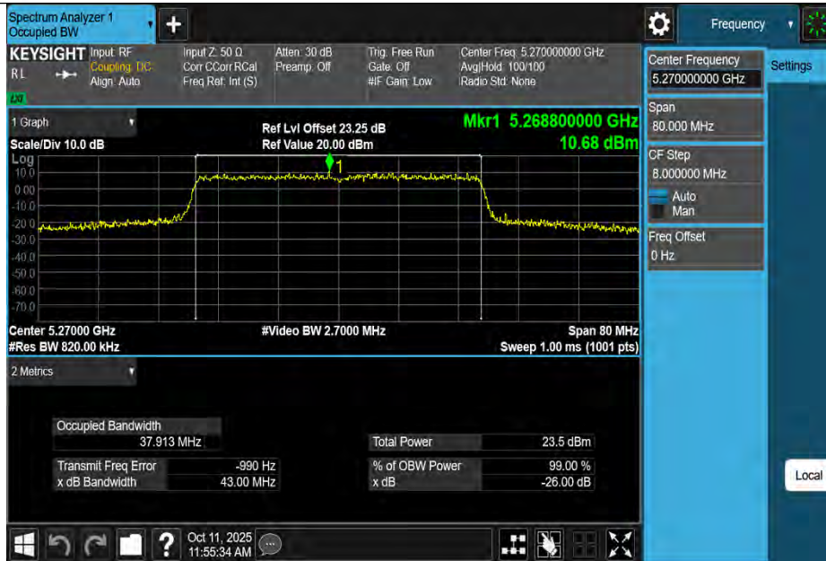
11AX40MIMO-Ant3-5270
