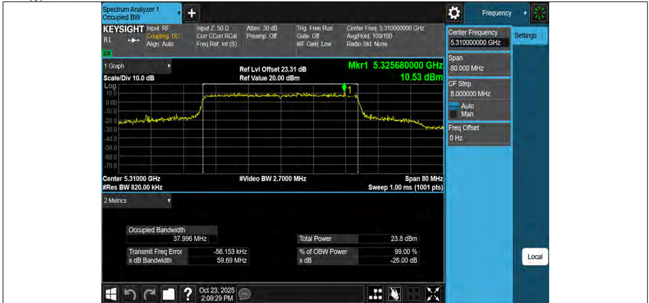
11AX40MIMO-Ant1-5310
