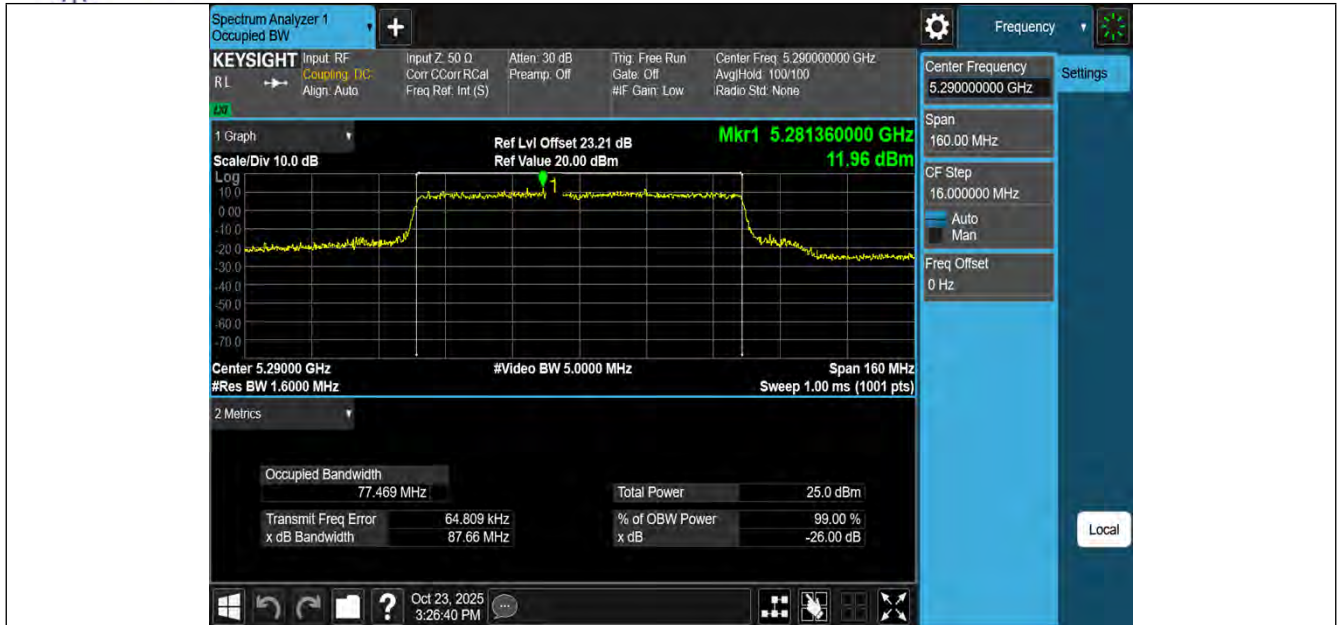
11AX80MIMO-Ant1-5290
