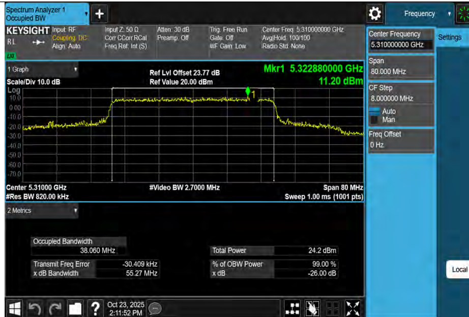
11AX40MIMO-Ant3-5310
