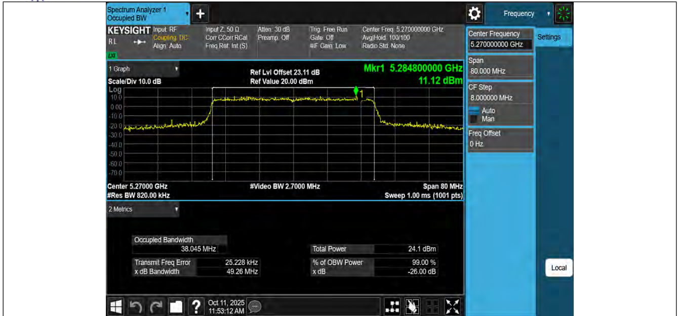
11AX40MIMO-Ant1-5270
