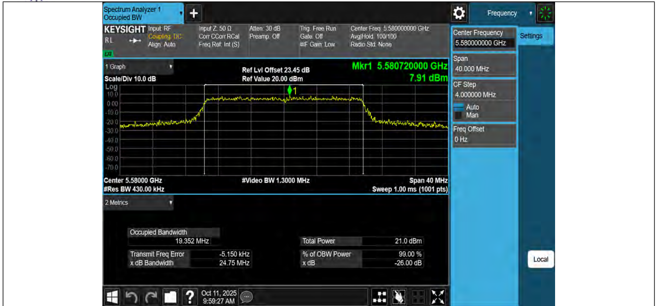
11AX20MIMO-Ant1-5580
