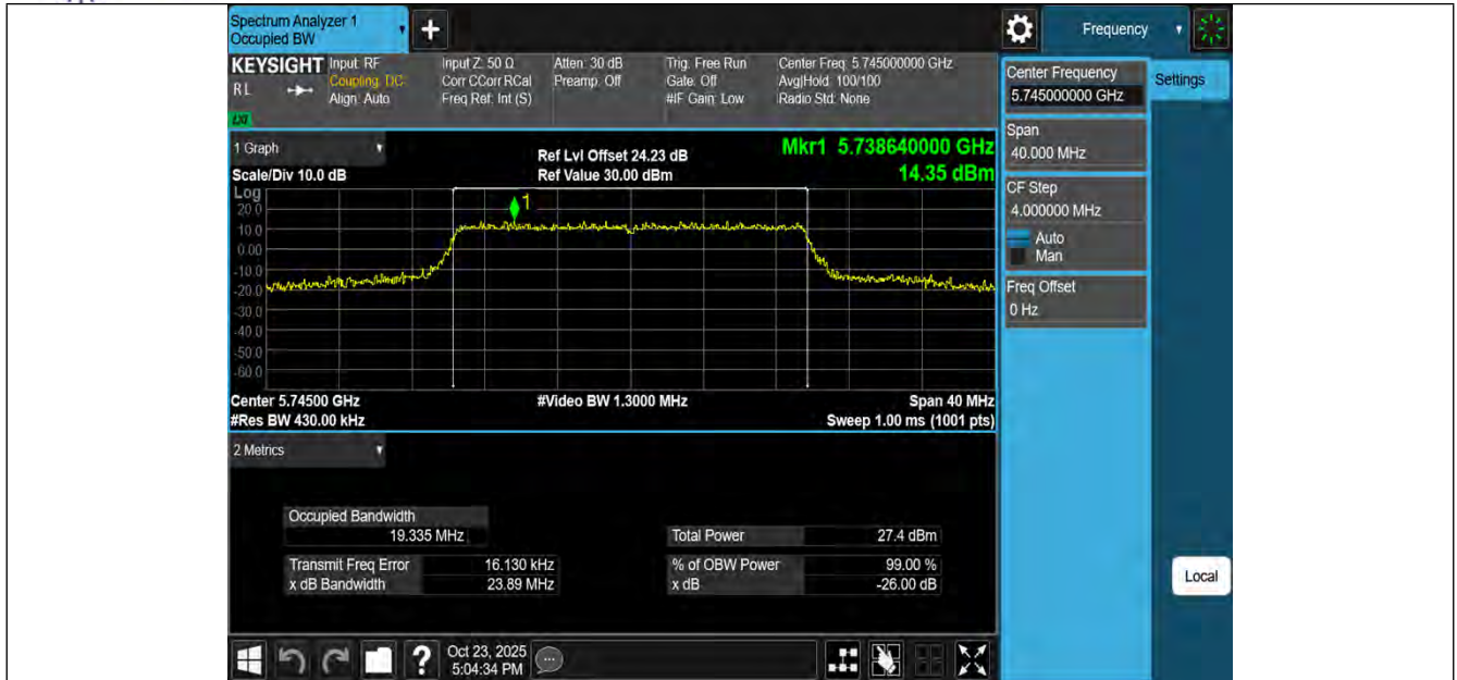
11AX20MIMO-Ant3-5745
