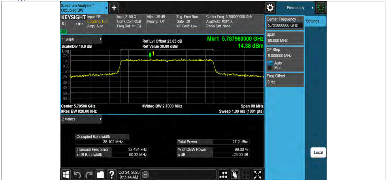
11AX40MIMO-Ant3-5795
