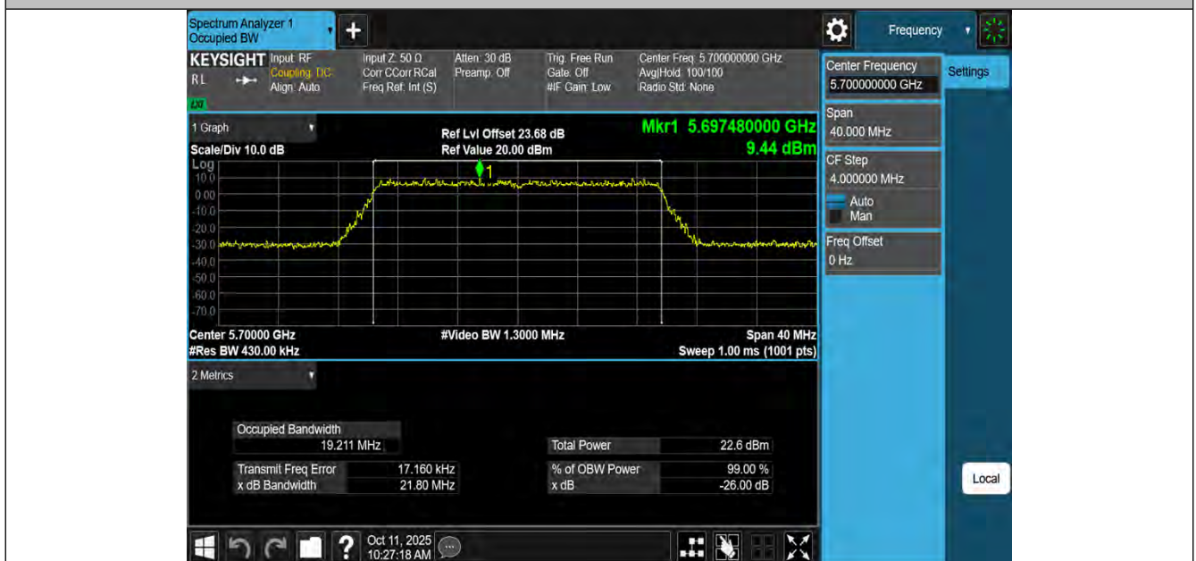
11AX20MIMO-Ant2-5700
