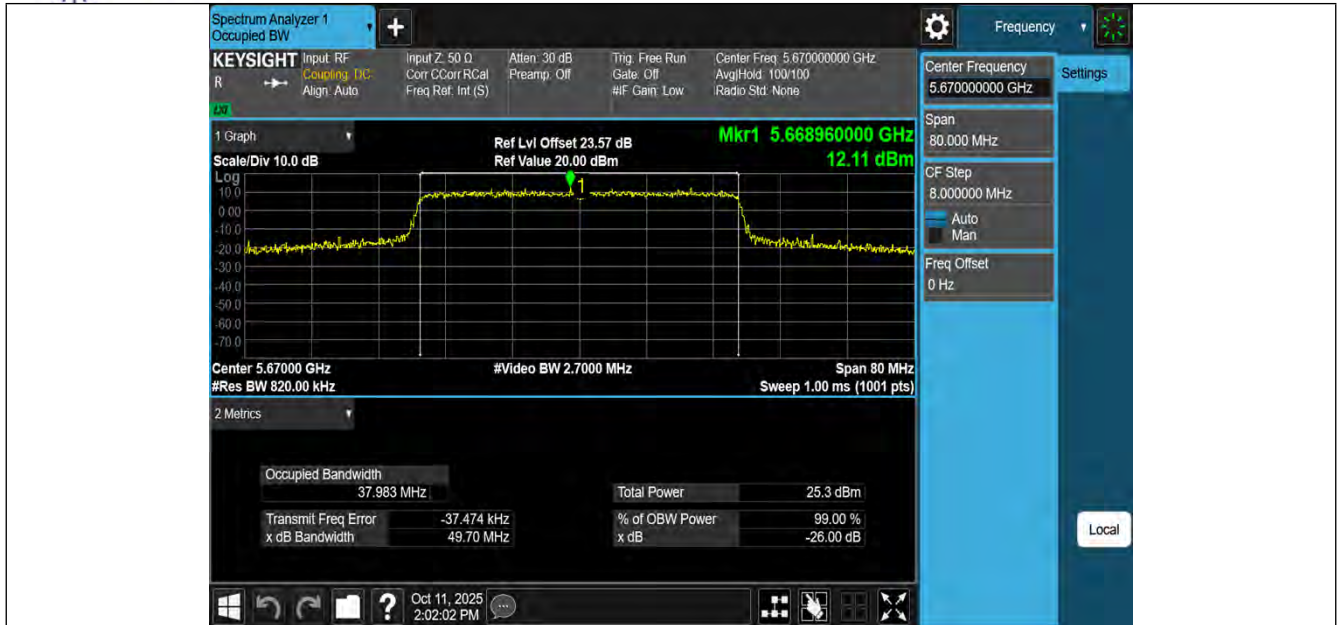
11AX40MIMO-Ant3-5670
