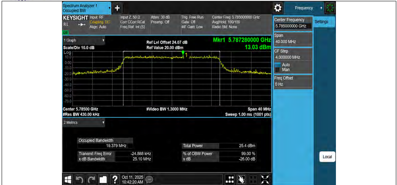
11AX20MIMO-Ant1-5785
