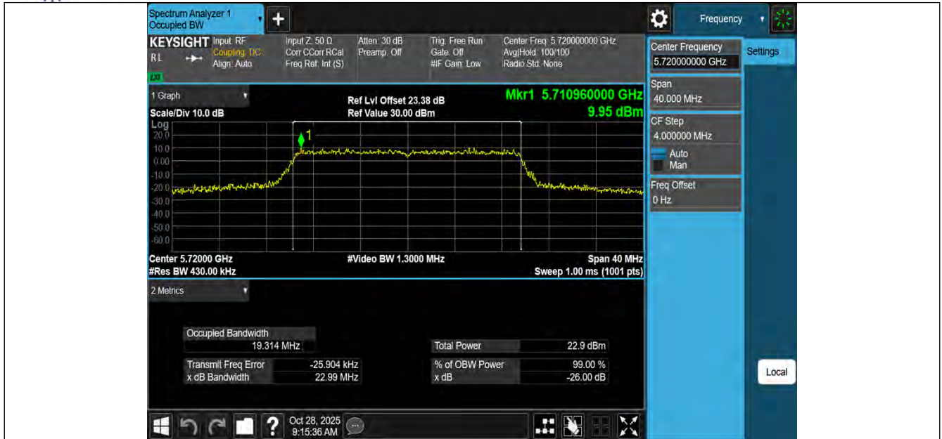
11AX20MIMO-Ant1-5720
