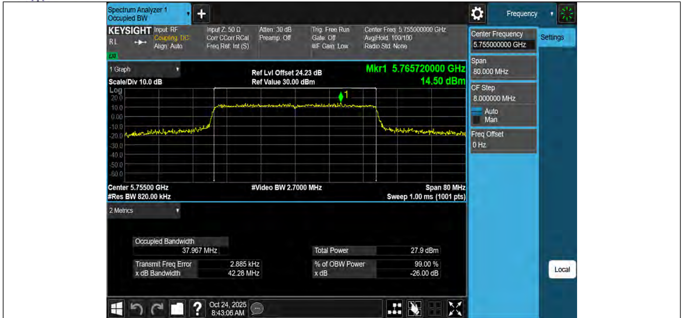
11AX40MIMO-Ant3-5755
