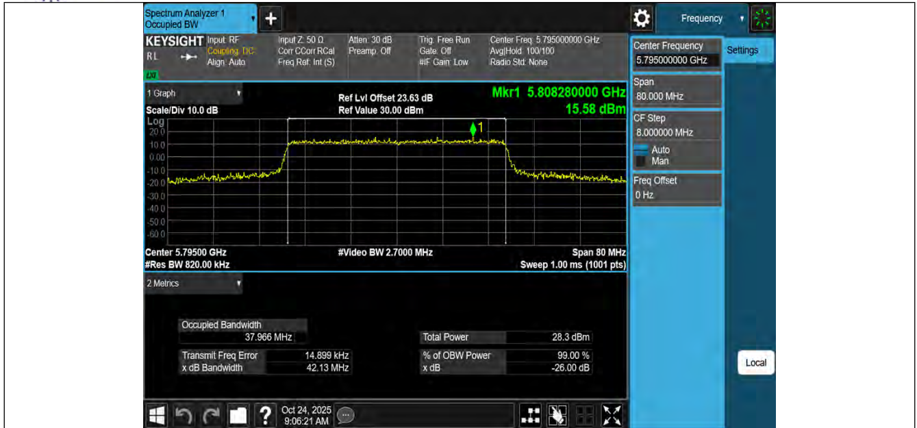
11AX40MIMO-Ant1-5795
