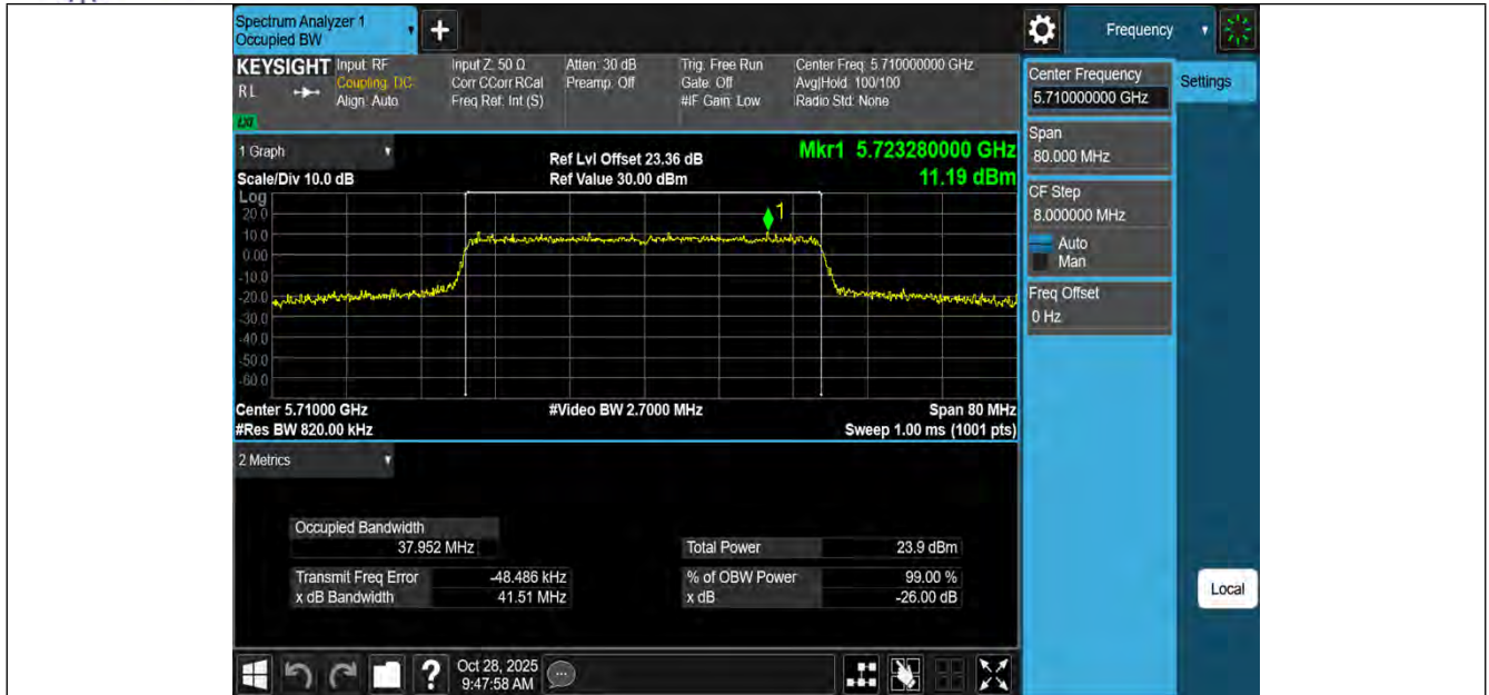
11AX40MIMO-Ant1-5710
