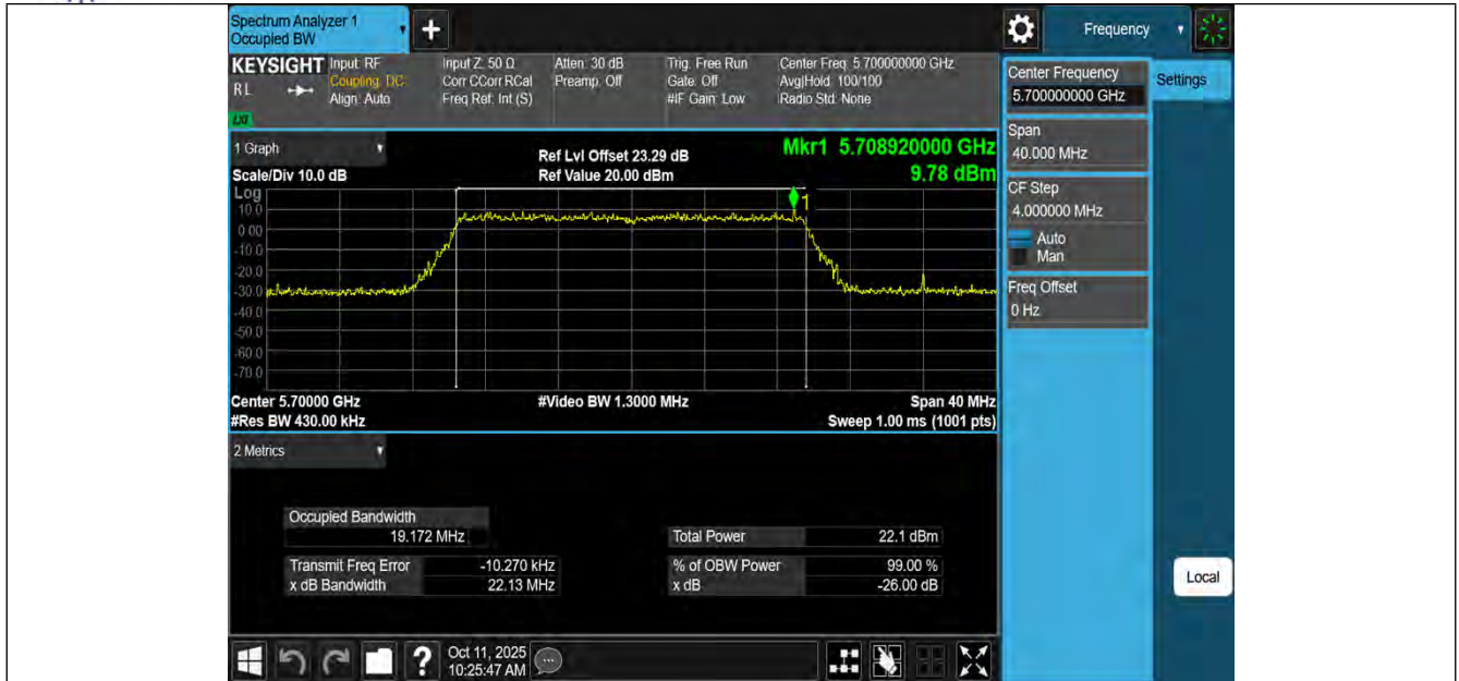
11AX20MIMO-Ant1-5700
