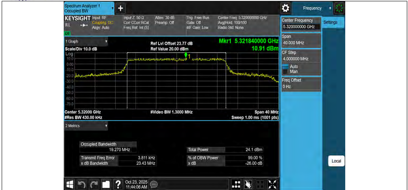
11AX20MIMO-Ant3-5320
