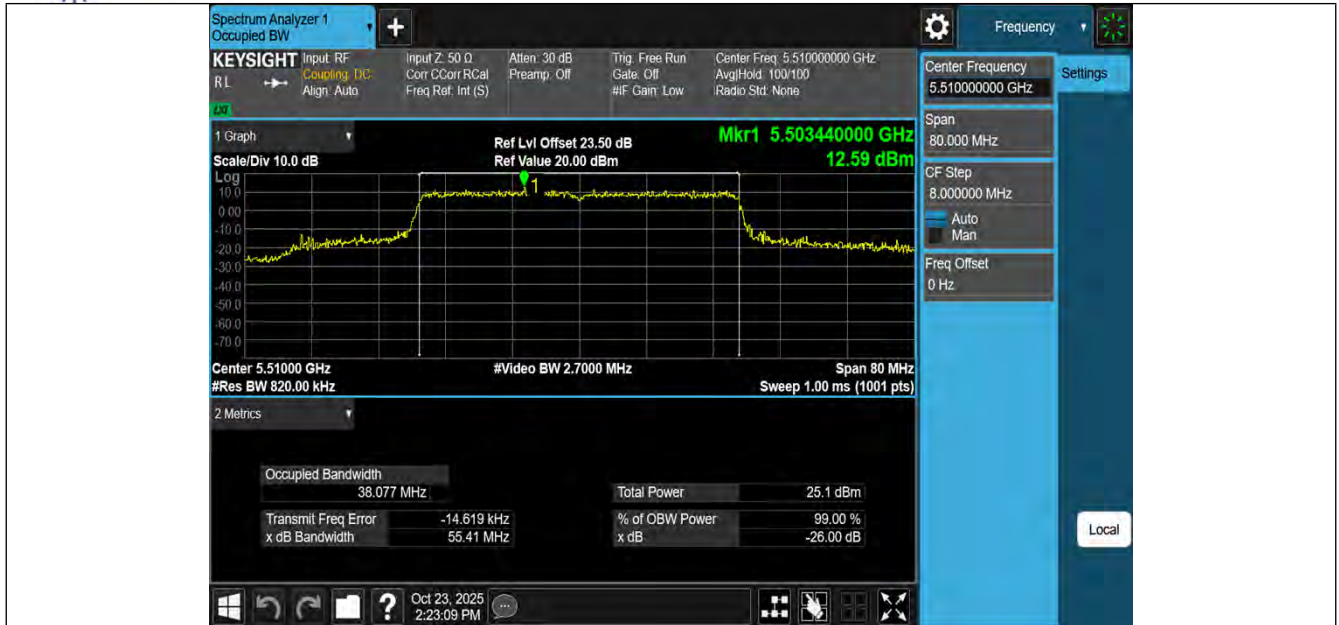
11AX40MIMO-Ant1-5510
