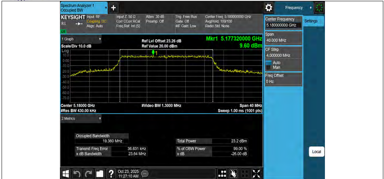
11AX20MIMO-Ant1-5180
