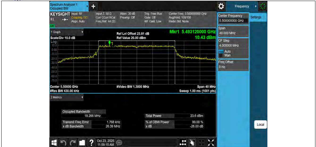
11AX20MIMO-Ant3-5500
