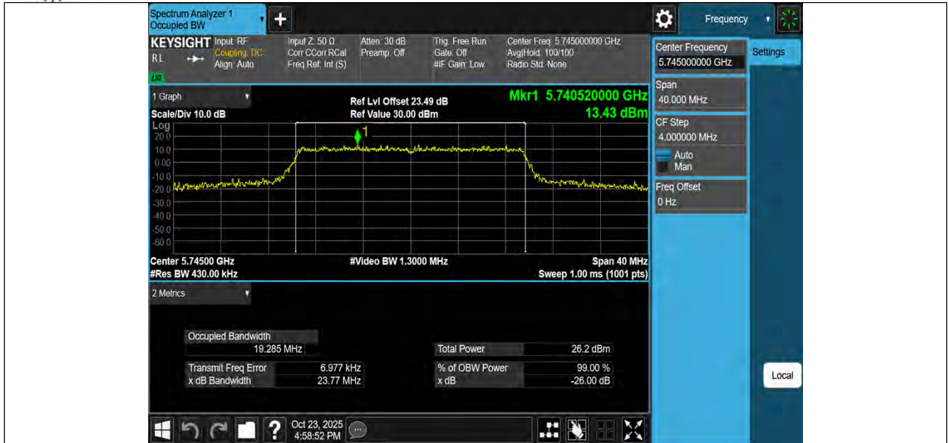
11AX20MIMO-Ant1-5745
