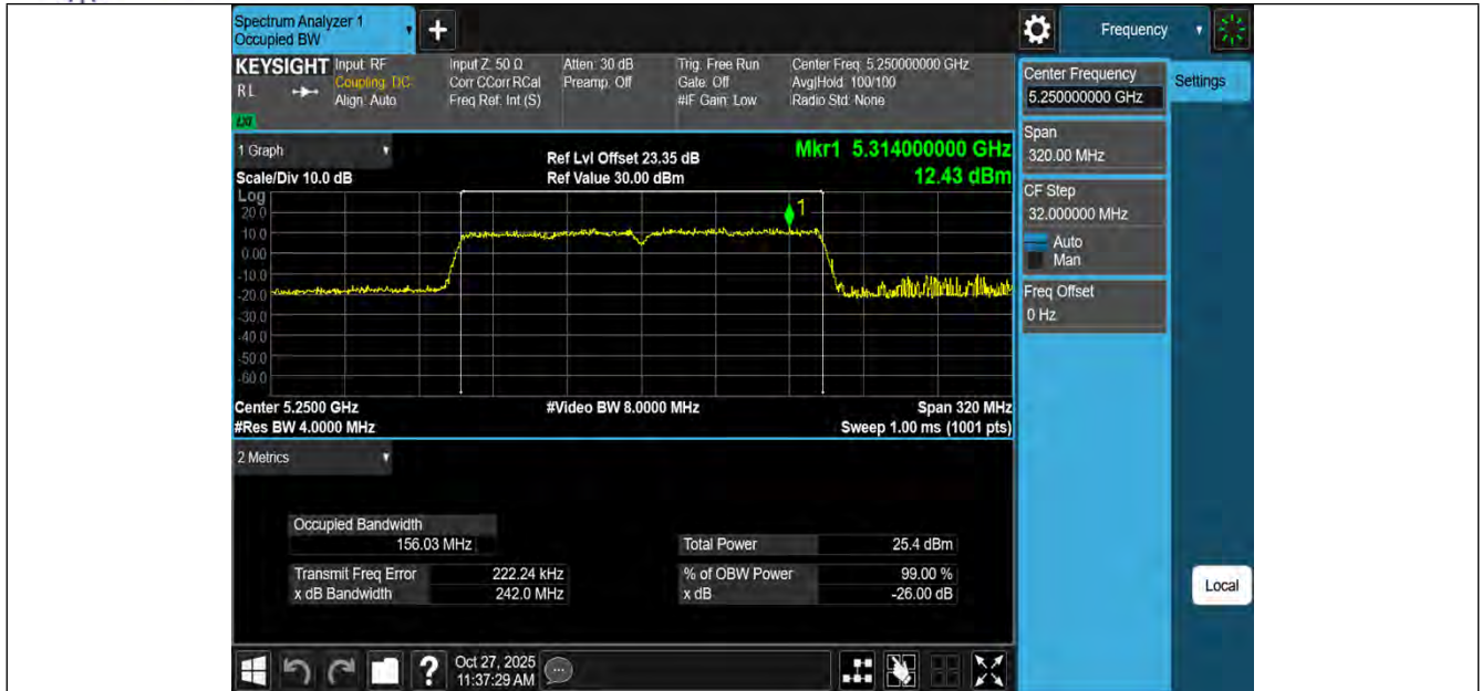
11AC160MIMO-Ant1-5250
