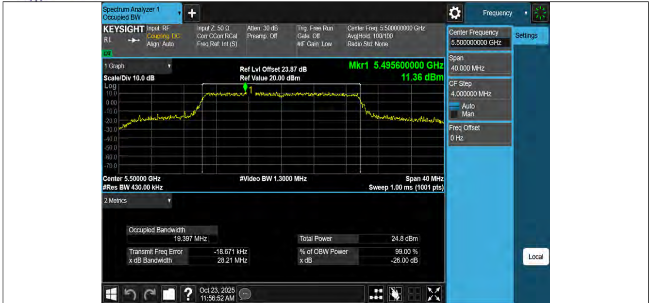
11AX20MIMO-Ant1-5500
