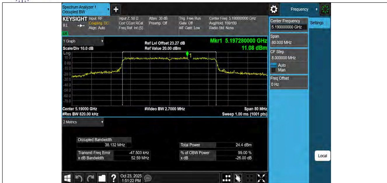
11AX40MIMO-Ant1-5190
