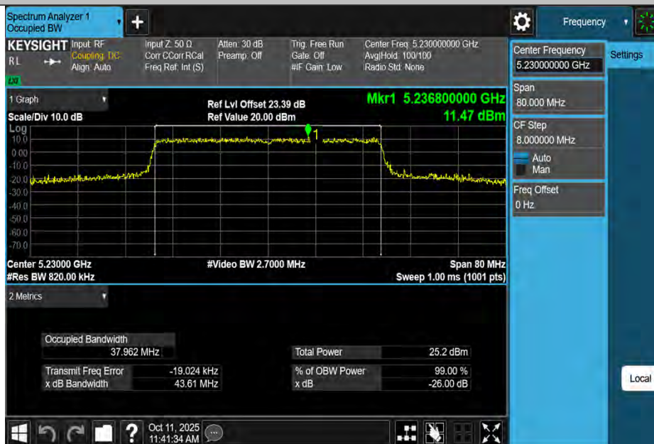
11AX40MIMO-Ant4-5230
