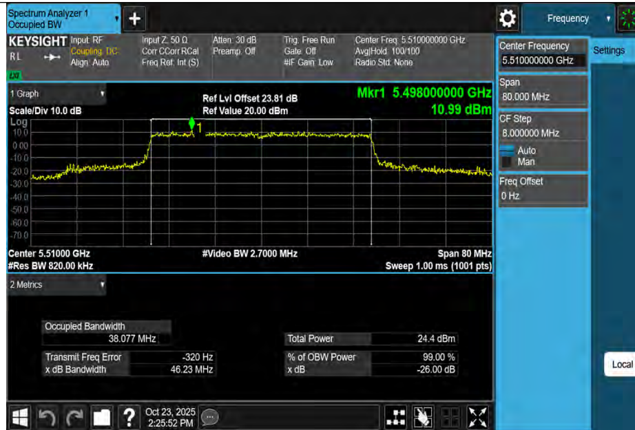
11AX40MIMO-Ant3-5510
