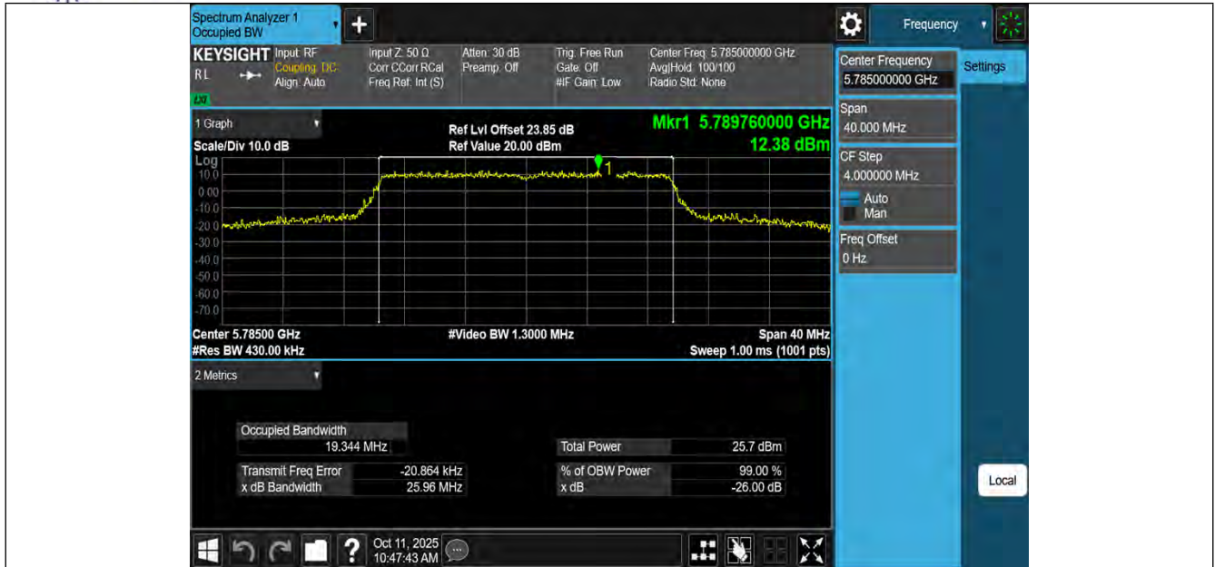
11AX20MIMO-Ant3-5785
