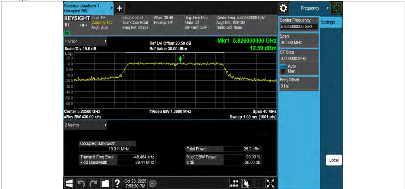
11AX20MIMO-Ant1-5825
