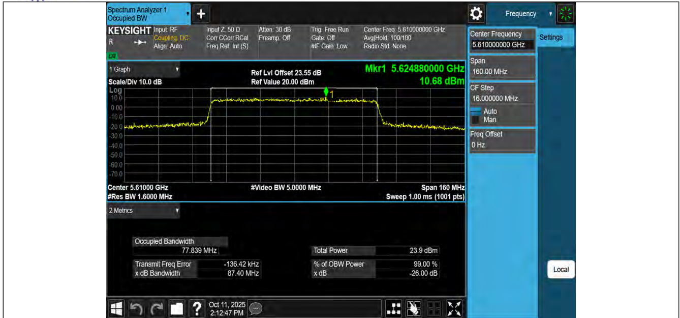
11AX80MIMO-Ant1-5610
