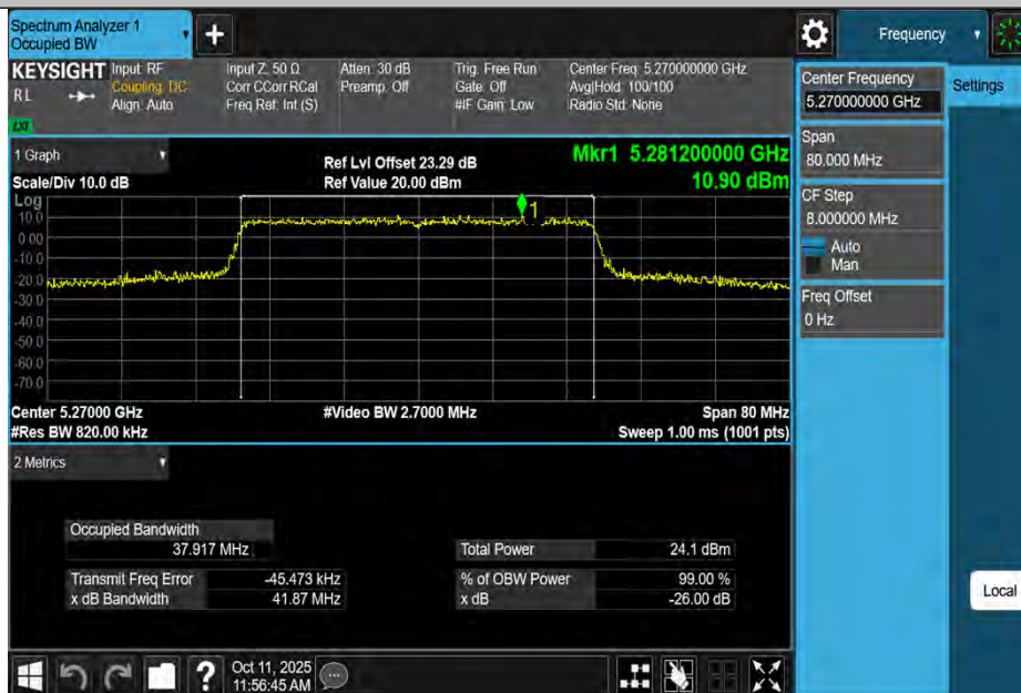
11AX40MIMO-Ant4-5270
