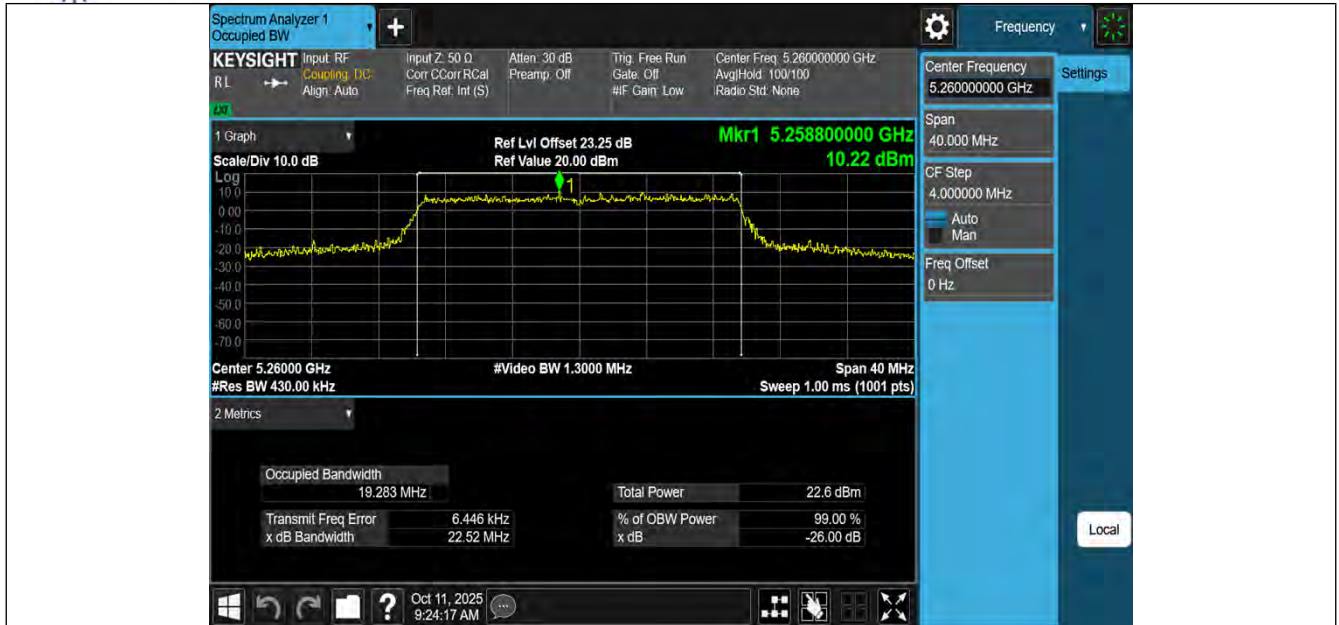
11AX20MIMO-Ant3-5260
