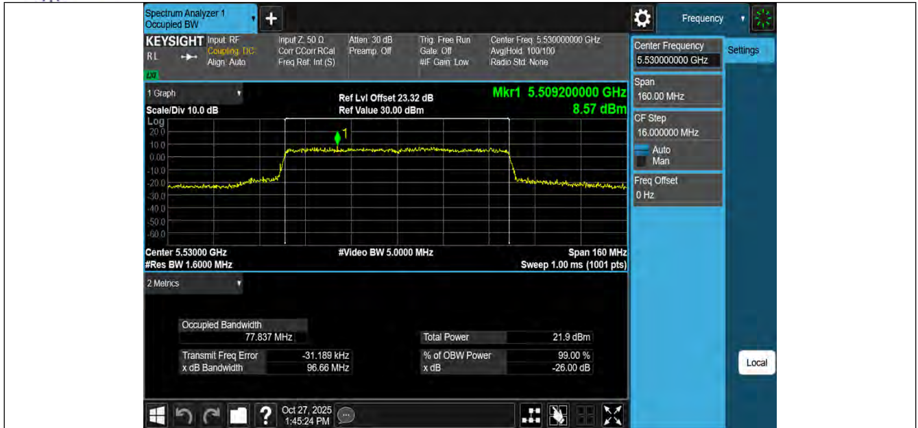
11AX80MIMO-Ant1-5530
