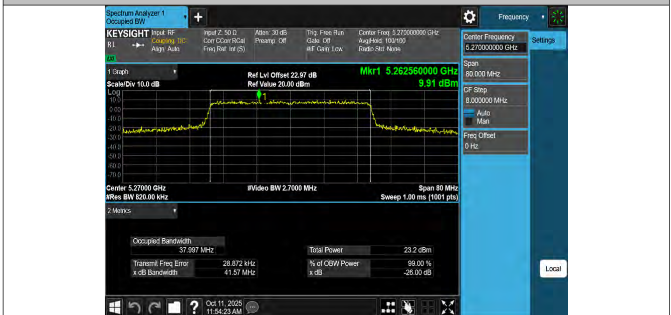
11AX40MIMO-Ant2-5270
