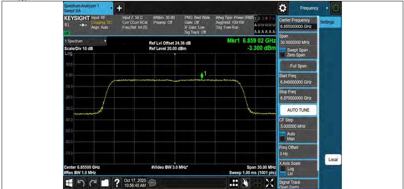
11BE20MIMO-Ant1-6855-PASS
