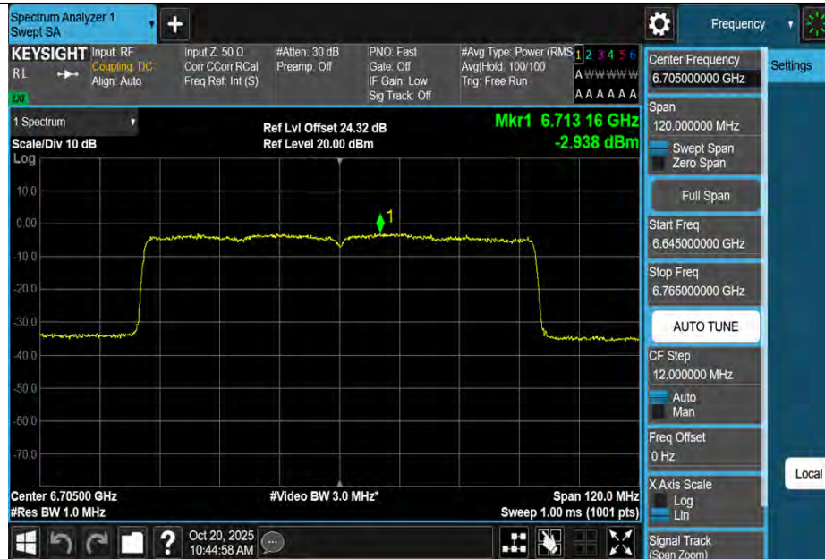
11BE80MIMO-Ant1-6705-PASS
