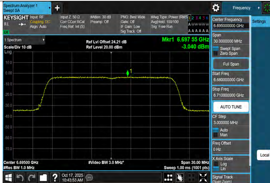
11BE20MIMO-Ant1-6695-PASS
