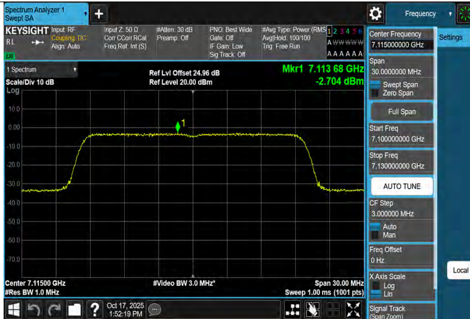
11BE20MIMO-Ant1-7115-PASS
