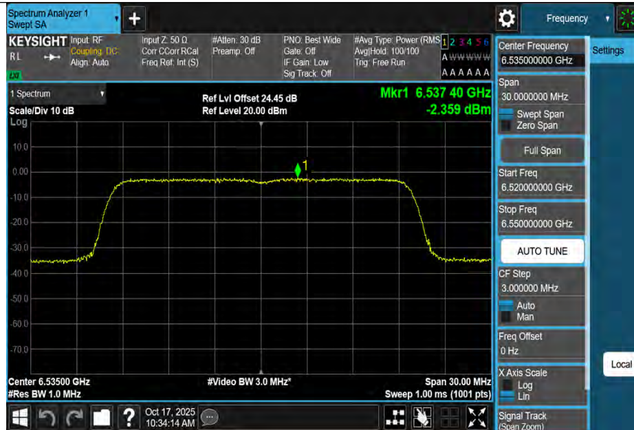
11BE20MIMO-Ant1-6535-PASS
