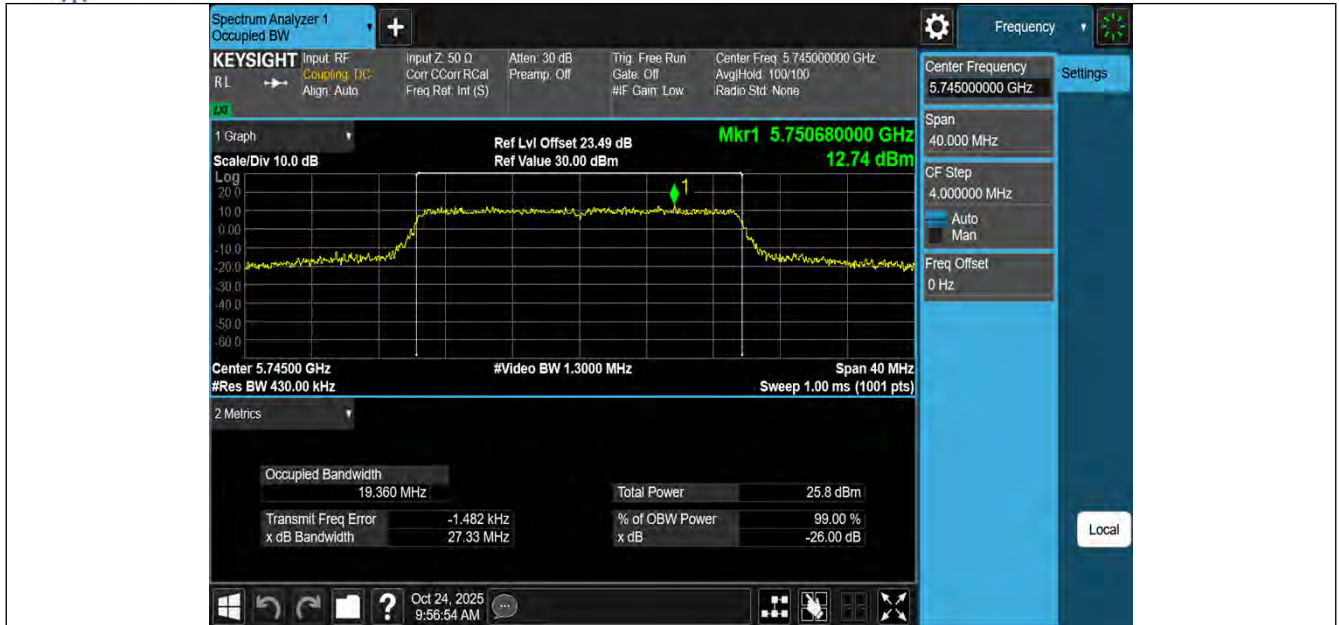
11BE20MIMO-Ant1-5745
