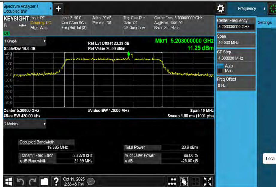
11BE20MIMO-Ant4-5200
