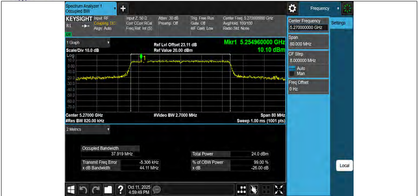
11BE40MIMO-Ant1-5270
