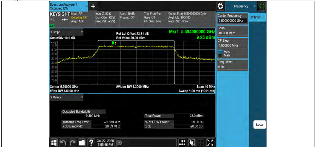
11BE20MIMO-Ant3-5500
