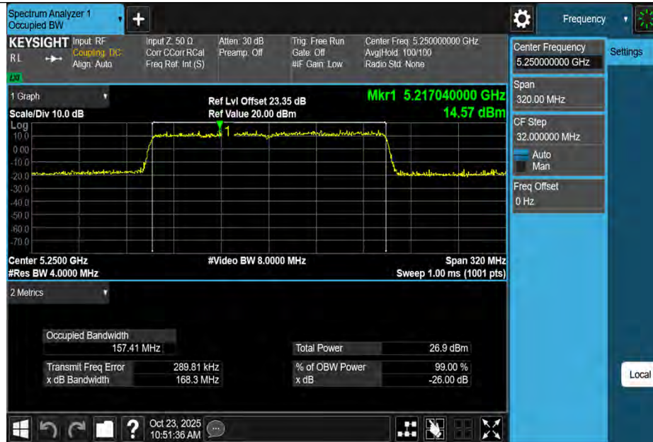
11BE160MIMO-Ant1-5250
