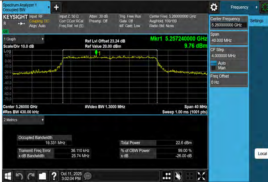
11BE20MIMO-Ant1-5260
