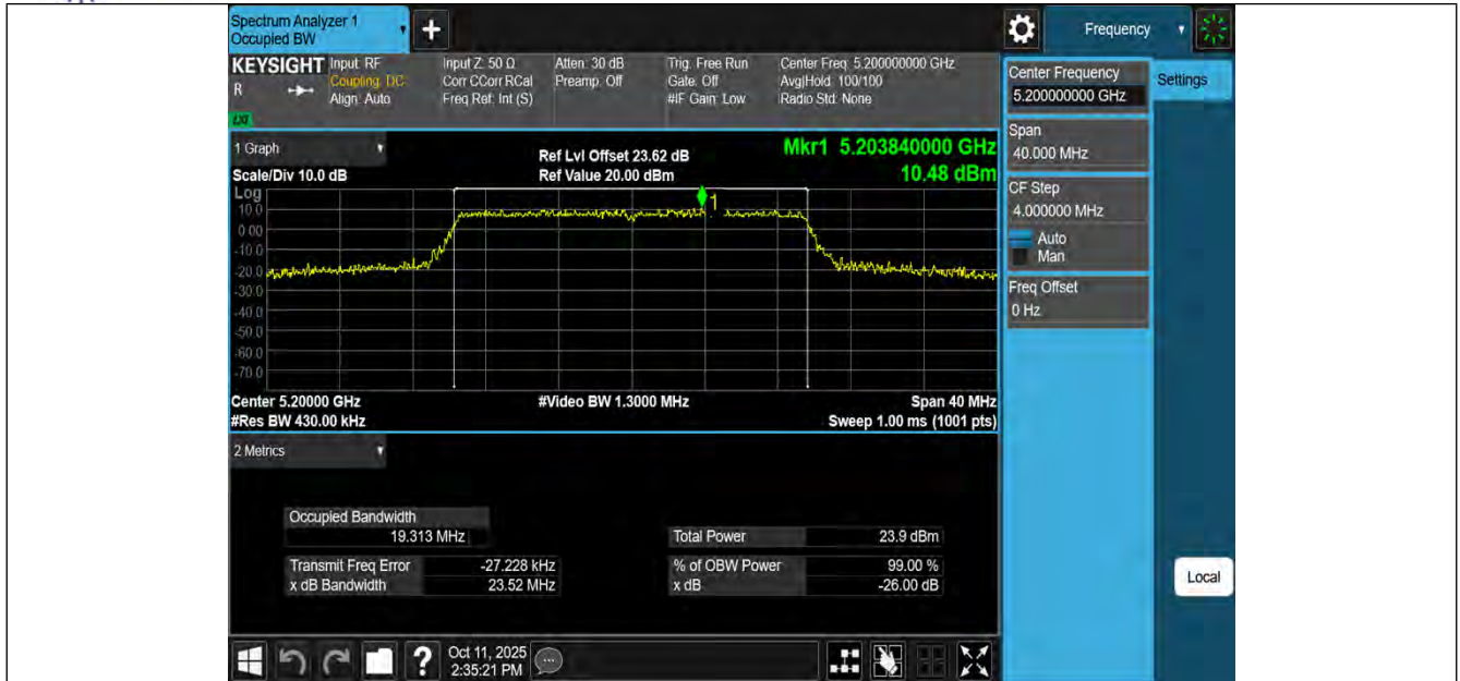
11BE20MIMO-Ant1-5200
