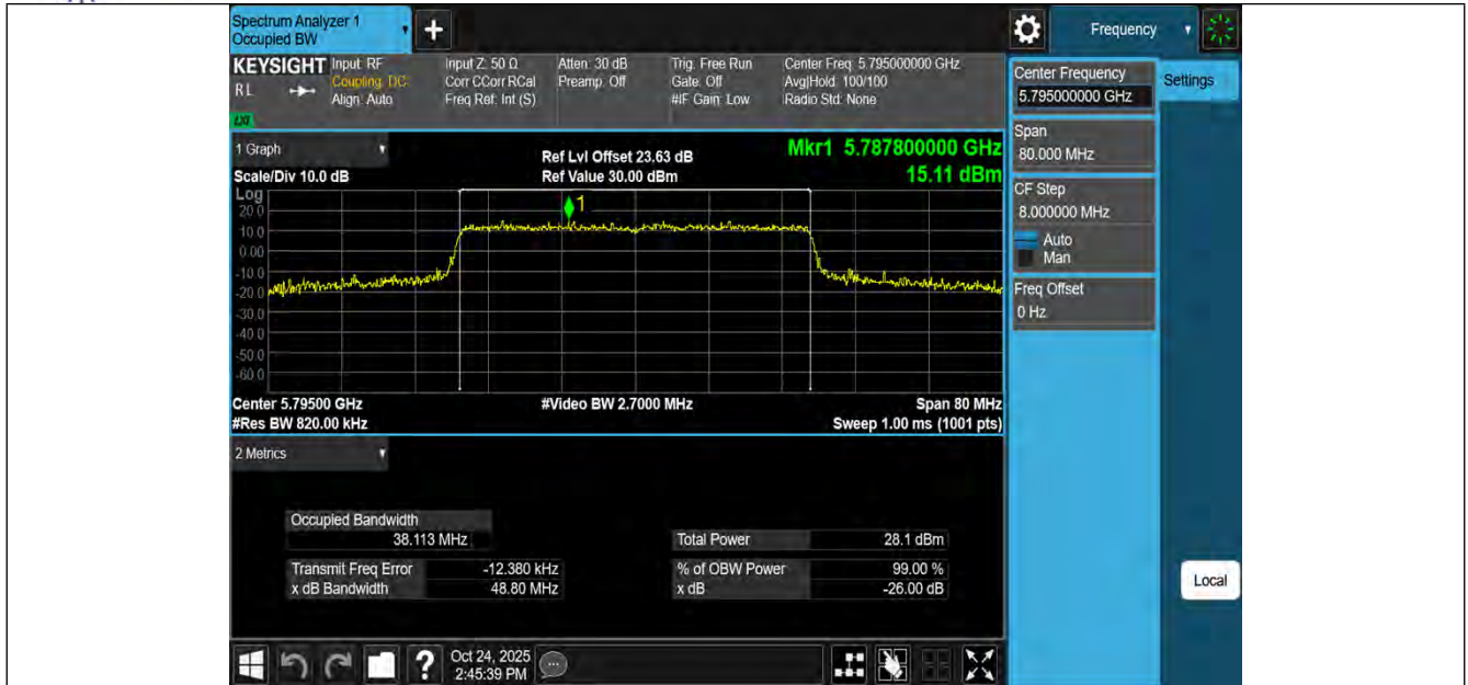
11BE40MIMO-Ant1-5795
