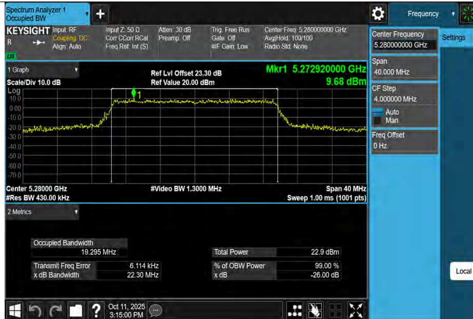
11BE20MIMO-Ant1-5280
