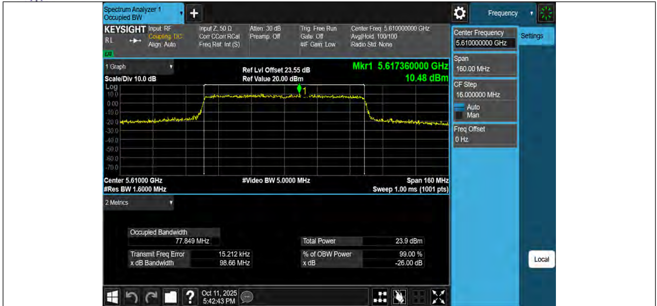
11BE80MIMO-Ant1-5610
