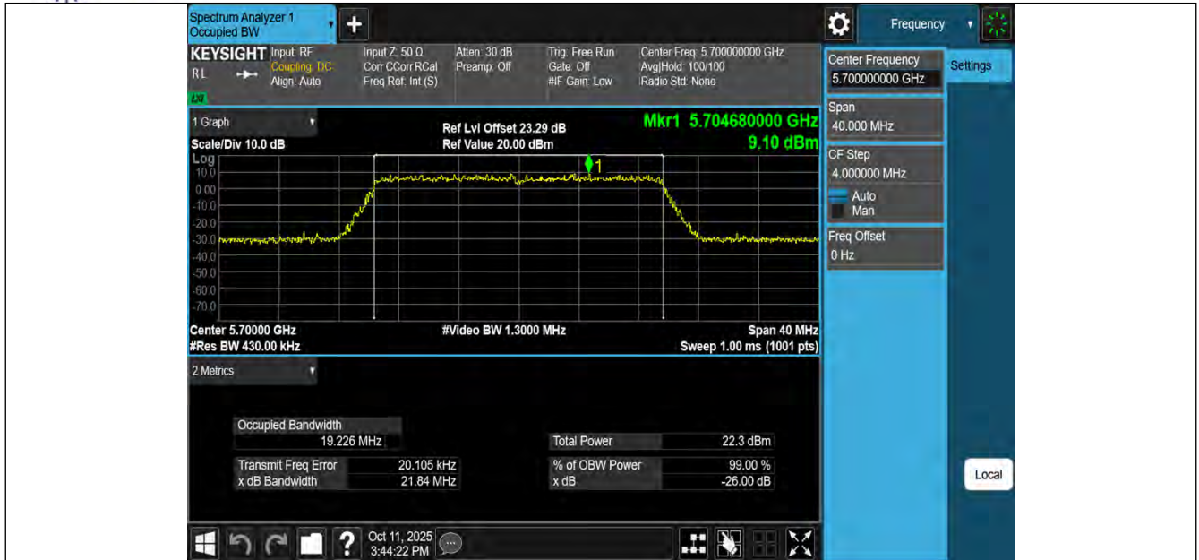
11BE20MIMO-Ant1-5700
