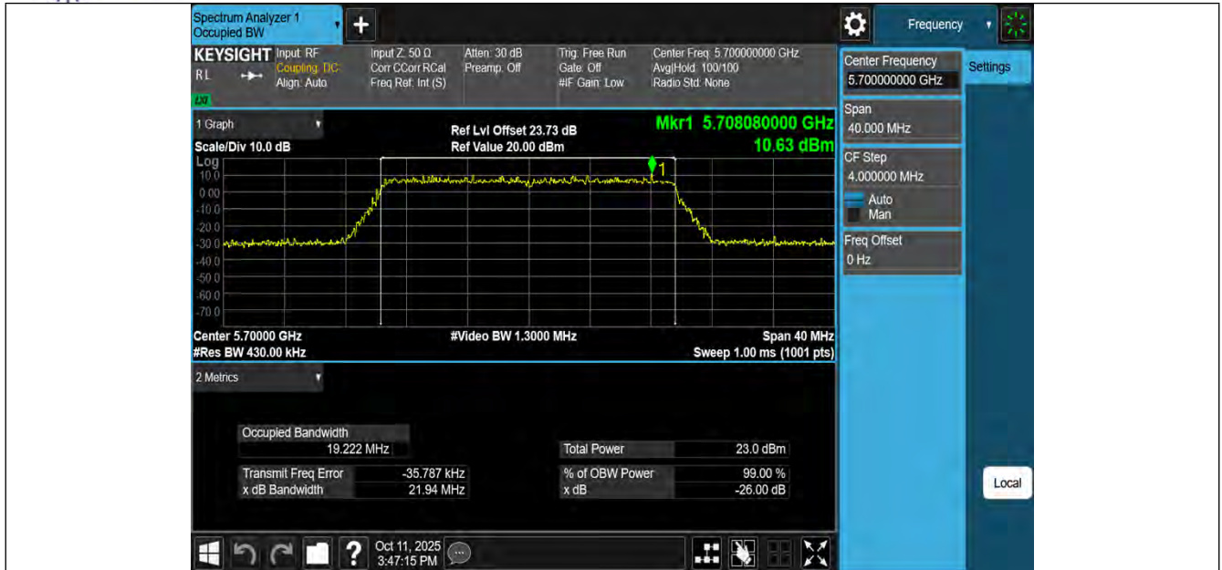
11BE20MIMO-Ant3-5700
