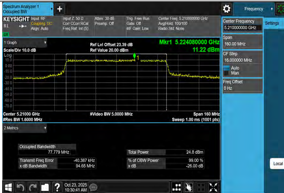
11BE80MIMO-Ant4-5210
