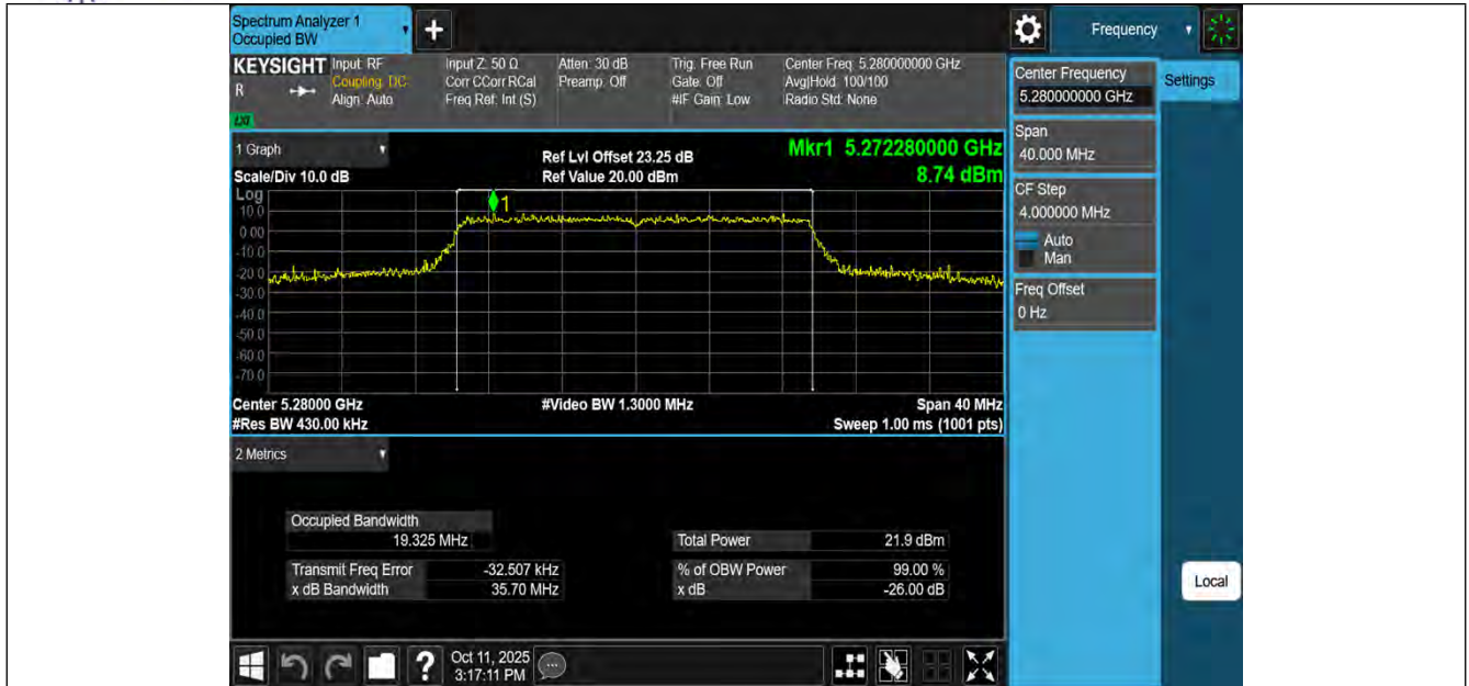
11BE20MIMO-Ant3-5280
