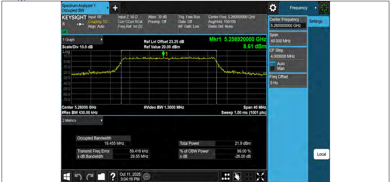
11BE20MIMO-Ant3-5260
