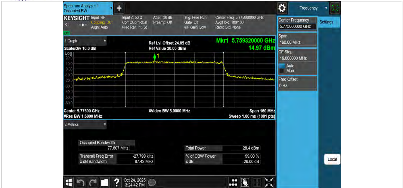
11BE80MIMO-Ant1-5775
