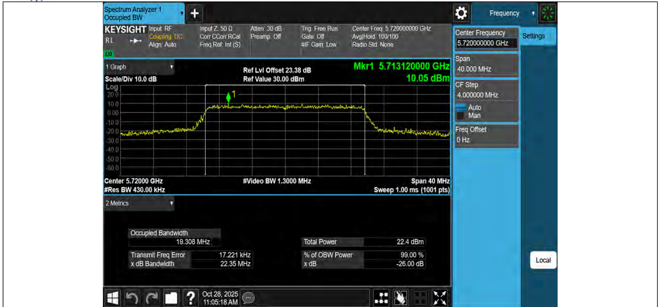
11BE20MIMO-Ant1-5720
