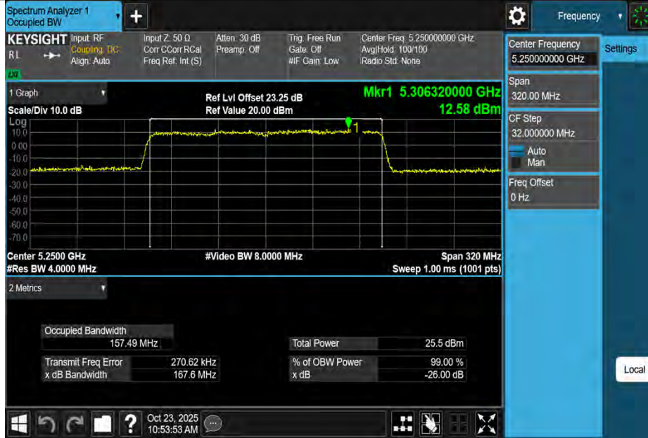
11BE160MIMO-Ant3-5250
