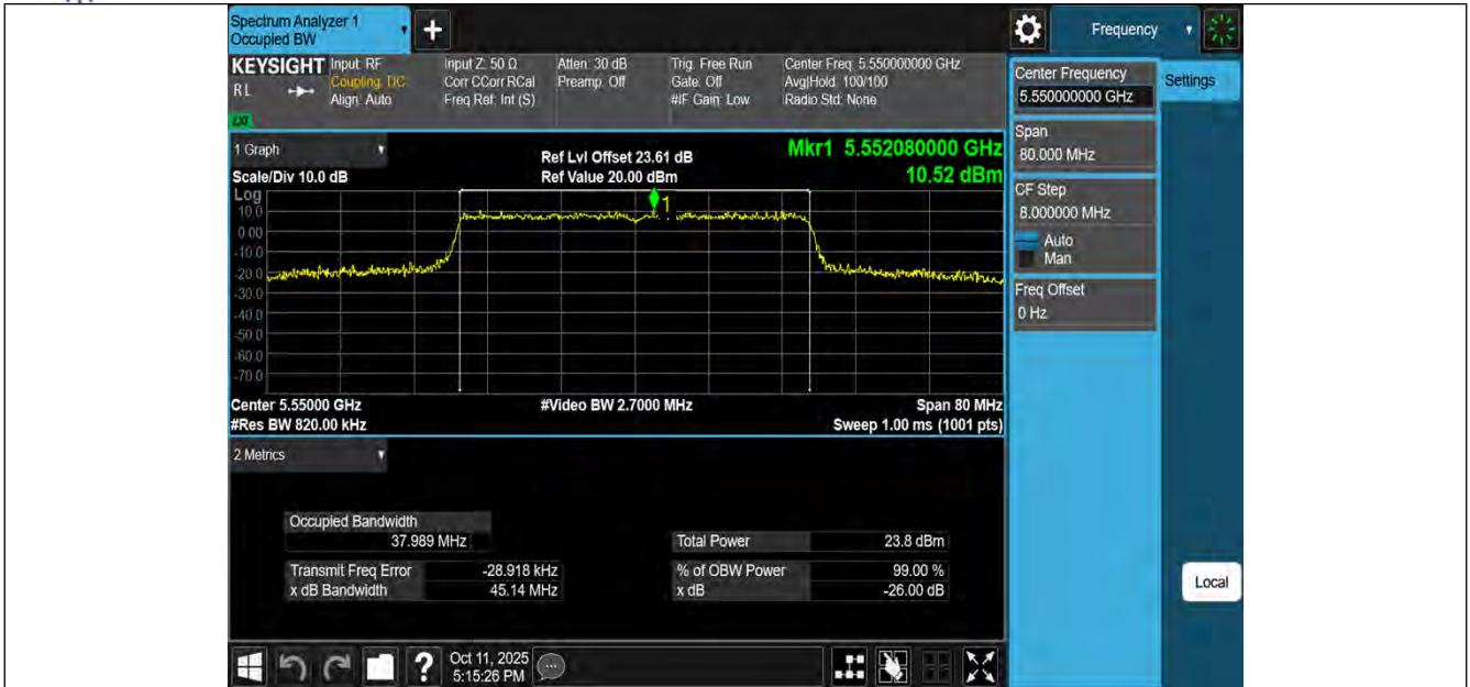
11BE40MIMO-Ant1-5550
