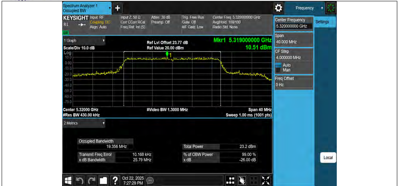
11BE20MIMO-Ant3-5320
