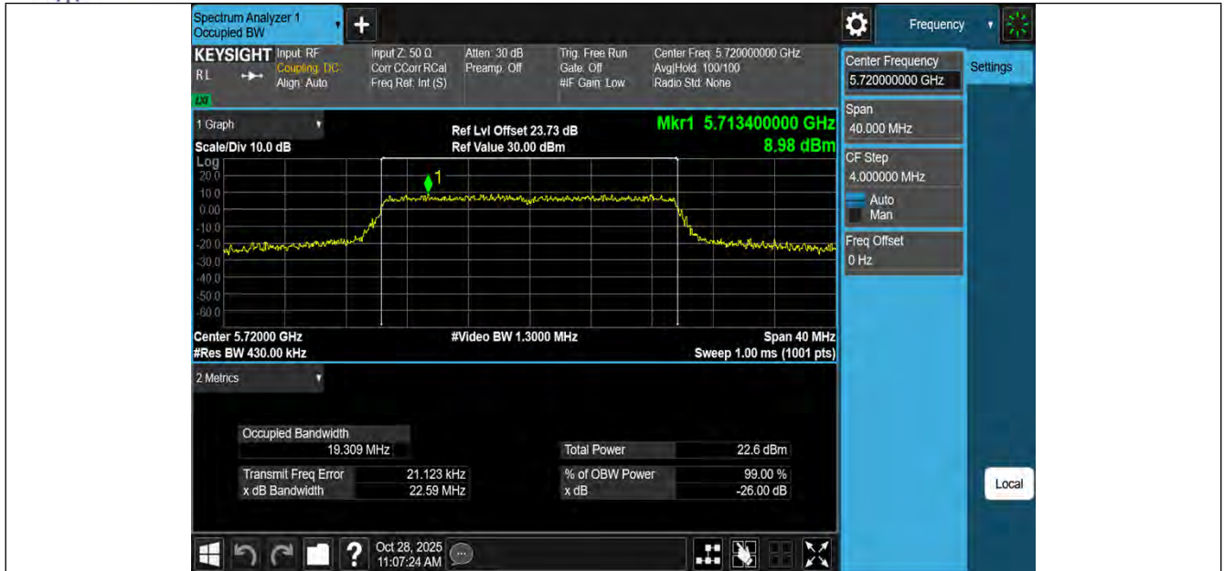
11BE20MIMO-Ant3-5720
