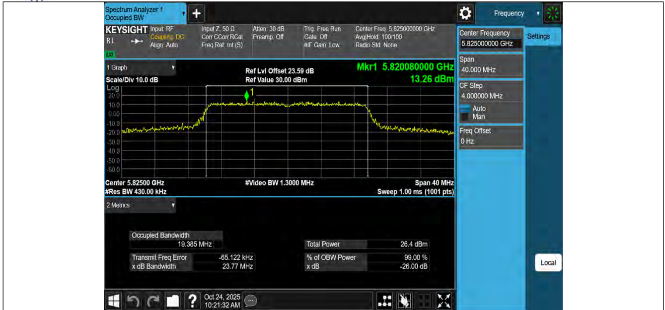
11BE20MIMO-Ant1-5825
