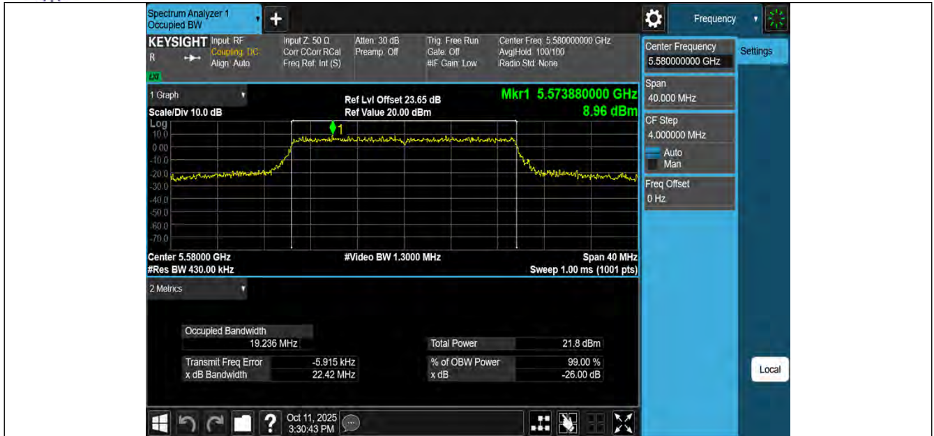
11BE20MIMO-Ant3-5580
