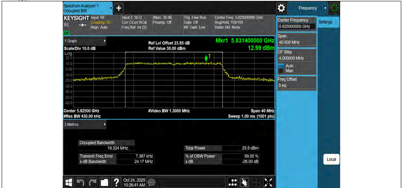
11BE20MIMO-Ant3-5825
