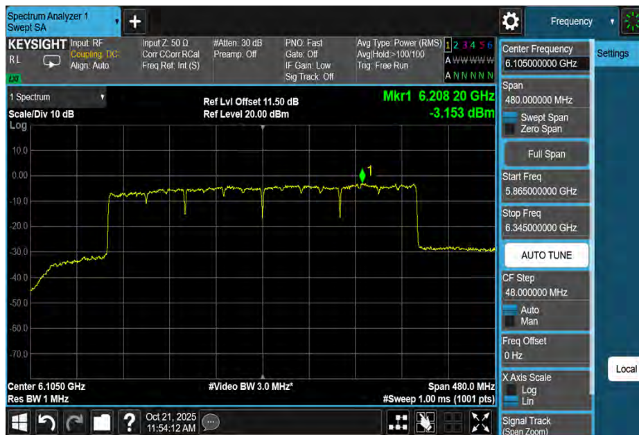
11BE320MIMO-Ant1-6105-PASS
