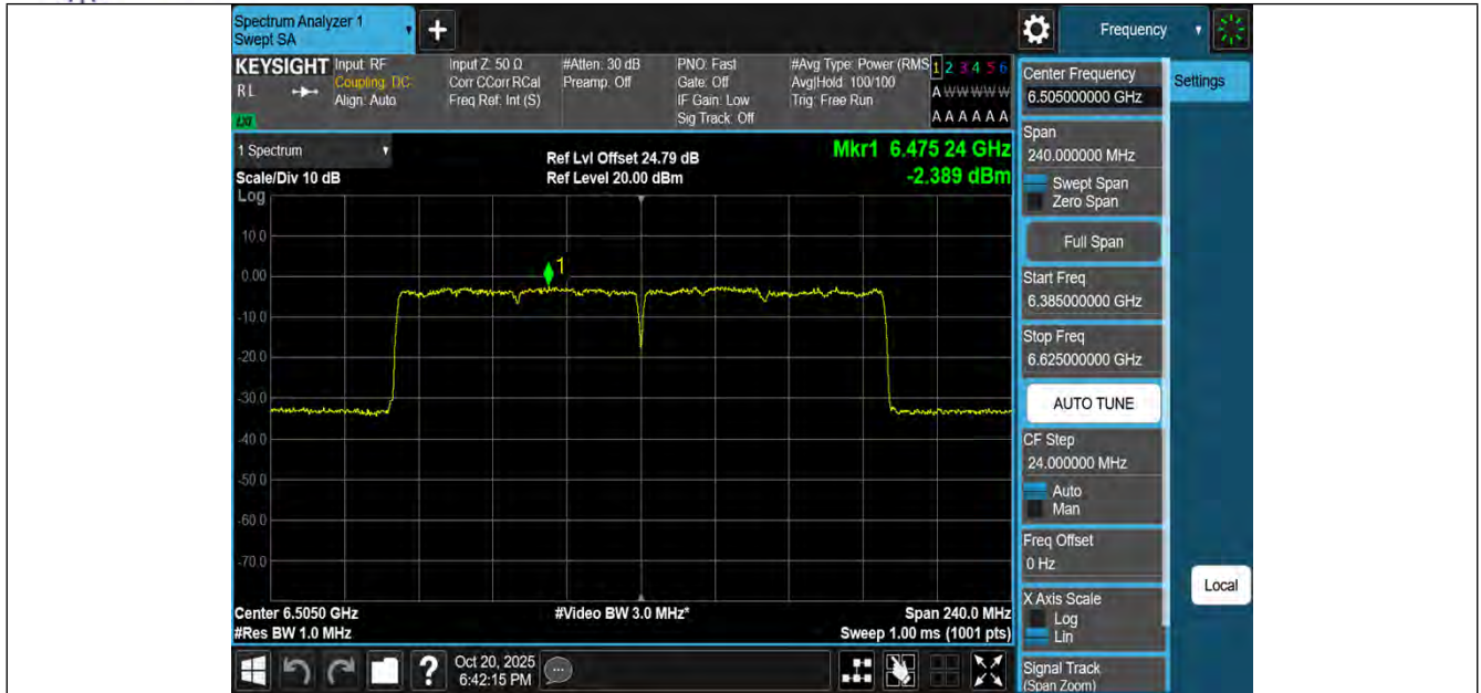
11BE160MIMO-Ant1-6505-PASS
