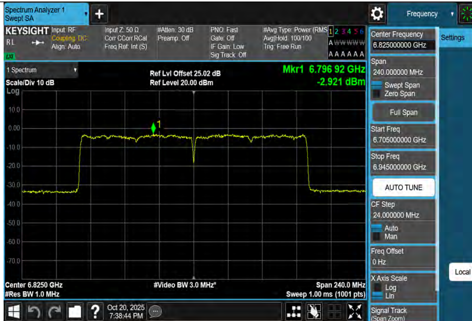
11BE160MIMO-Ant1-6825-PASS
