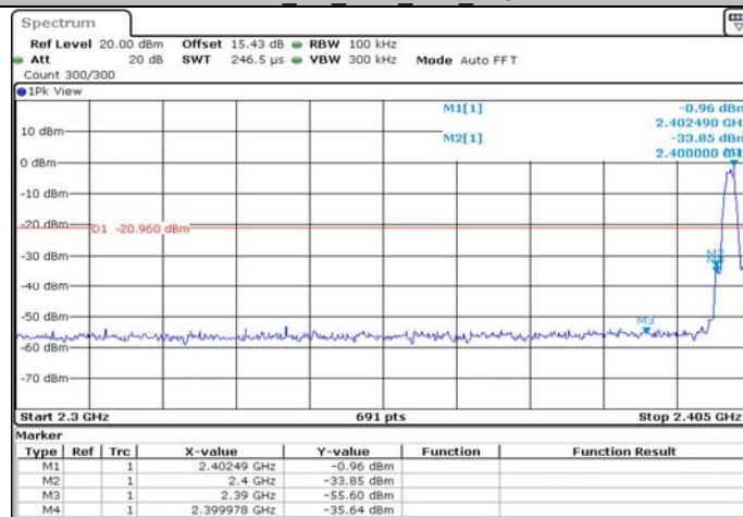
BLE_2M_Ant1_Low_2402
