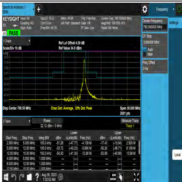
NTNV-Band14-5MHz-QPSK-23305-25RB#0--5.00--2.50-PASS
