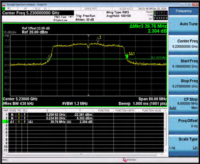
11N40MIMO Ant8 5230
