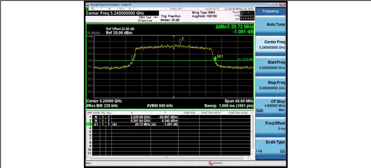
11AX20MIMO_Ant8_5240
