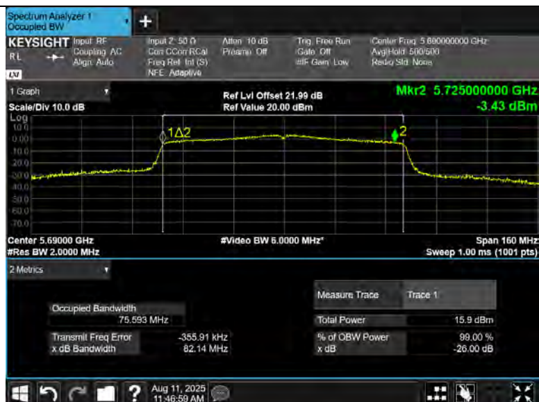
11AC80MIMO_Ant6_5690_UNII-2C
