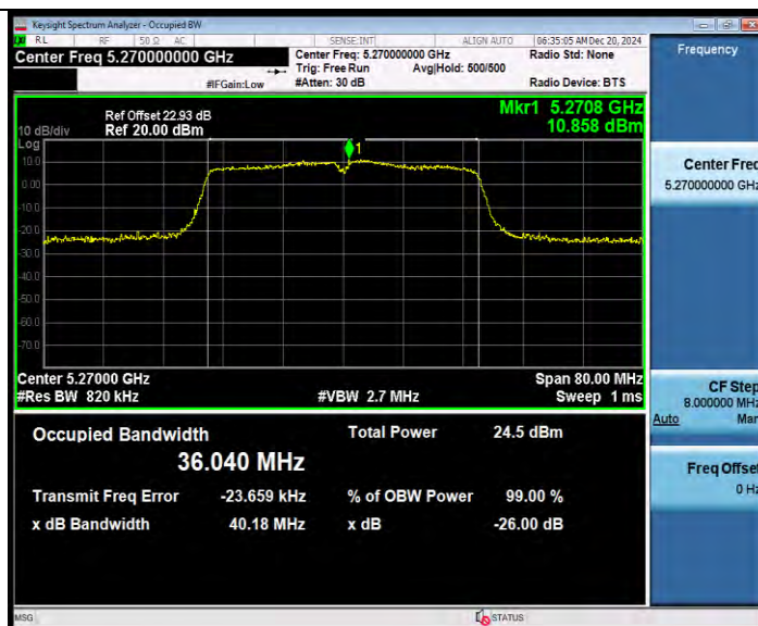
11N40MIMO_Ant8_5270
