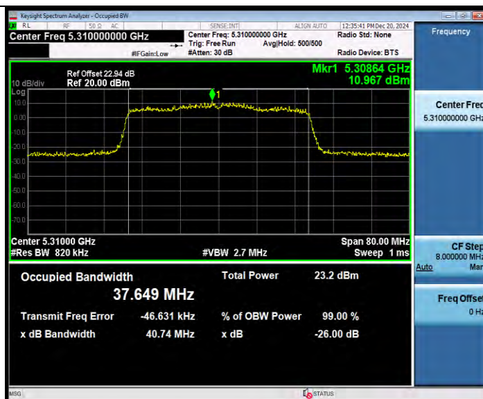
11AX40MIMO_Ant8_5310
