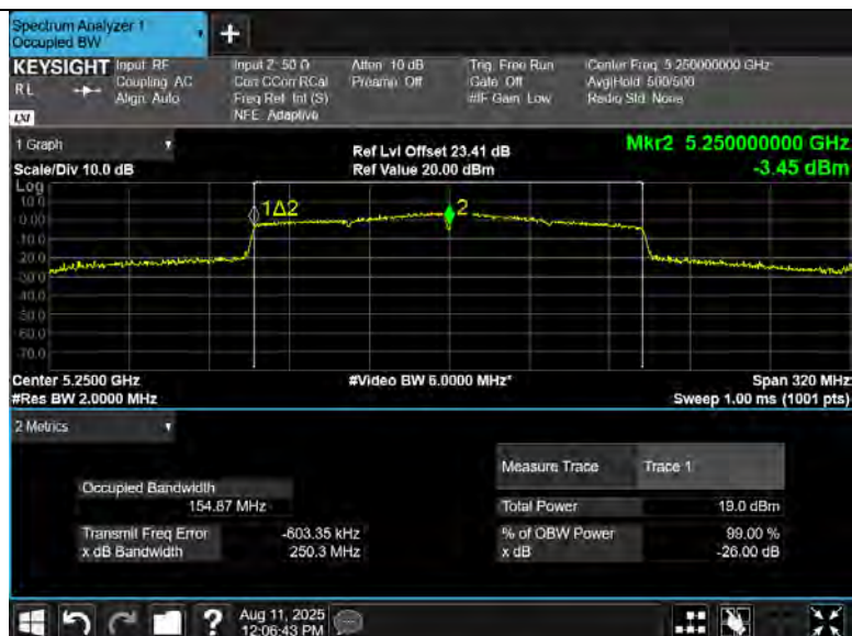
11AC160MIMO_Ant6_5250_UNII-1
