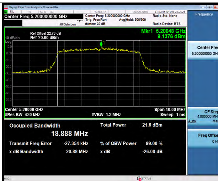
11AX20MIMO_Ant8_5200
