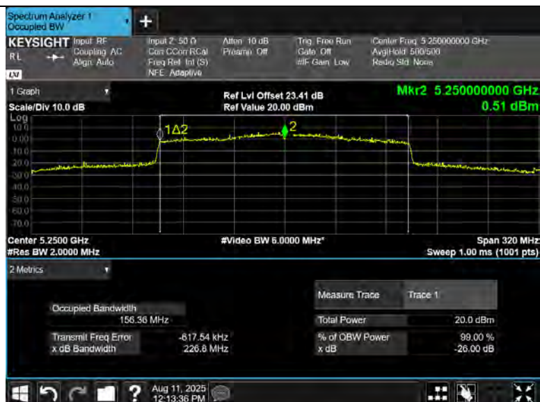
11AX160MIMO_Ant6_5250_UNII-1
