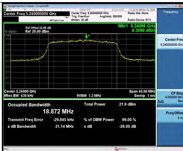
11AX20MIMO_Ant8_5240
