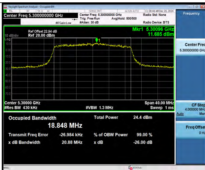
11AX20MIMO_Ant8_5300
