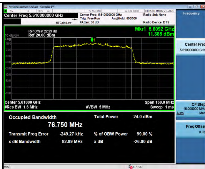
11AX80MIMO_Ant8_5610
