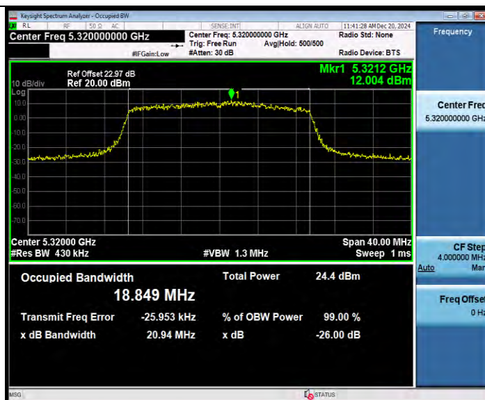
11AX20MIMO_Ant8_5320
