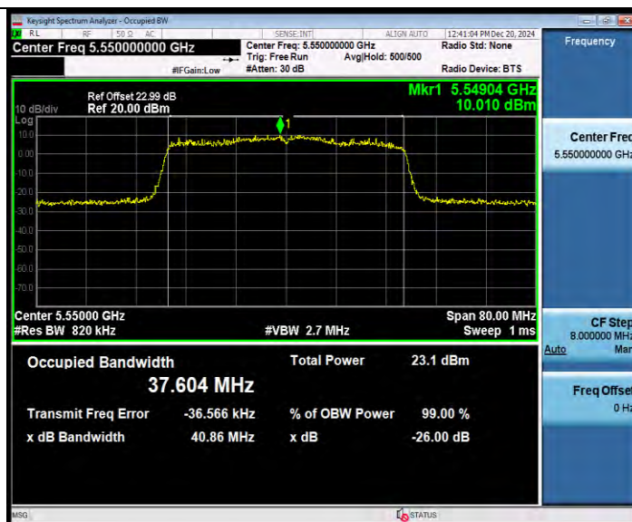
11AX40MIMO_Ant8_5550
