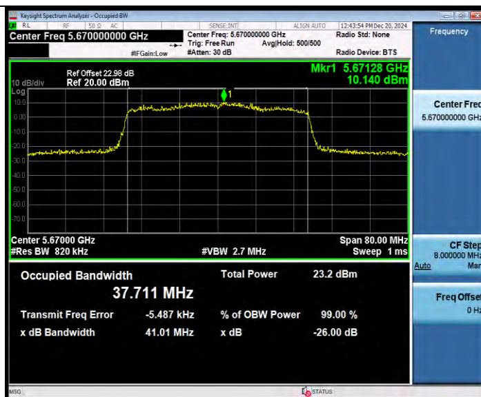
11AX40MIMO_Ant8_5670
