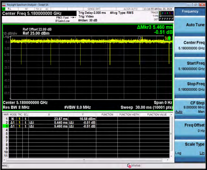
11AX20MIMO_Ant8_5180
