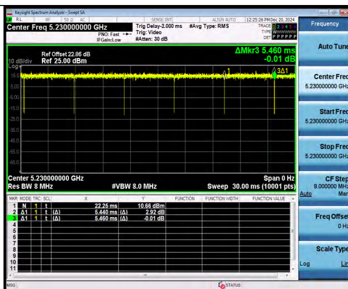
11AX40MIMO_Ant8_5230
