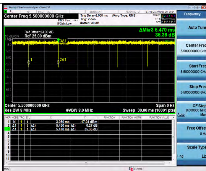
11AX20MIMO_Ant8_5500
