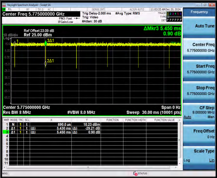
11AC80MIMO_Ant8_5775
