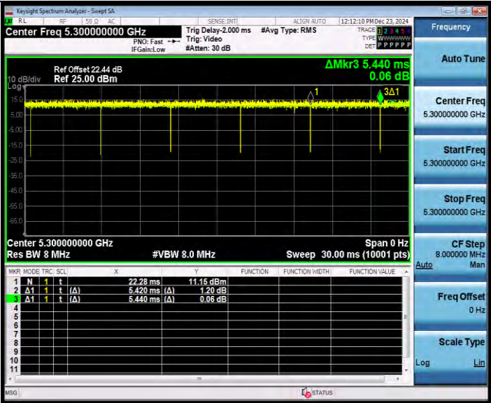
11N20MIMO Ant8 5300
