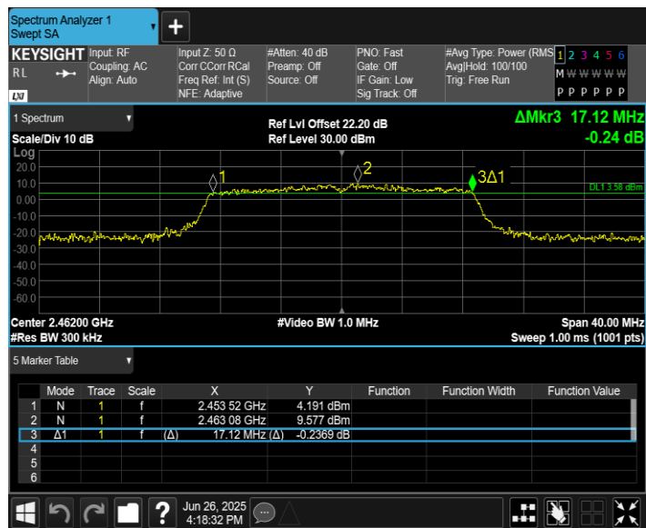
11N20MIMO_Ant8_2462
