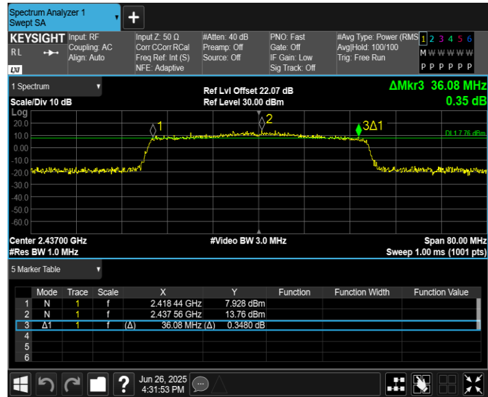
11AX40MIMO_Ant8_2437
