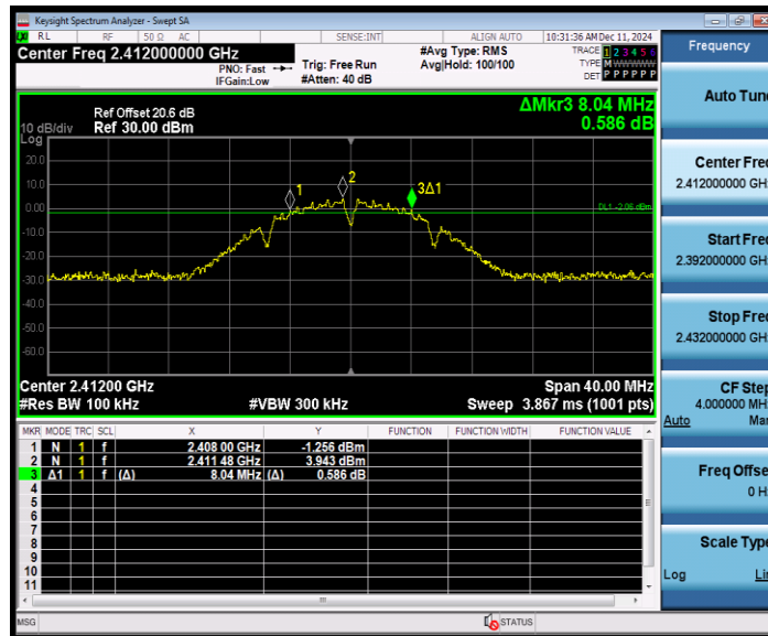
11B-CDD_Ant8_2412
