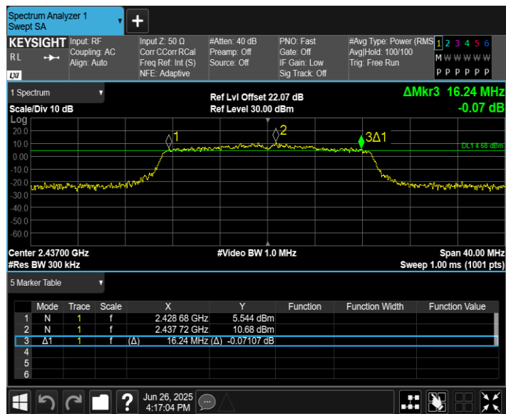
11N20MIMO_Ant8_2437
