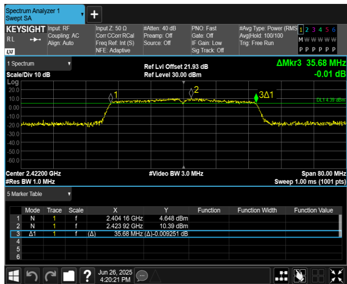
11N40MIMO_Ant8_2422
