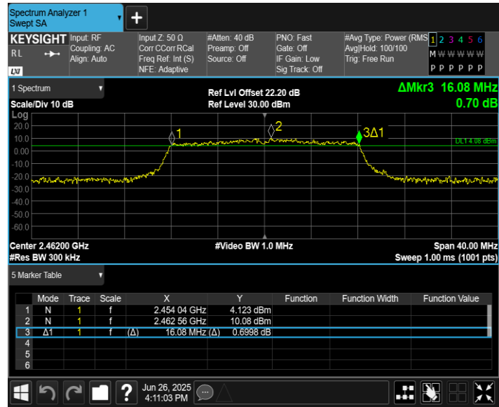
11G-CDD_Ant8_2462
