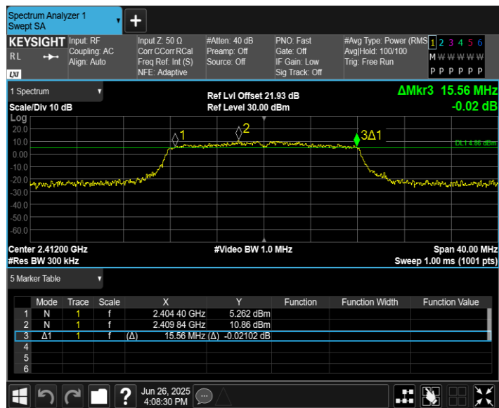
11G-CDD_Ant8_2412
