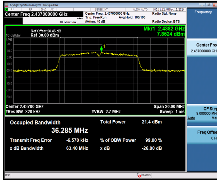
11N40MIMO_Ant8_2437
