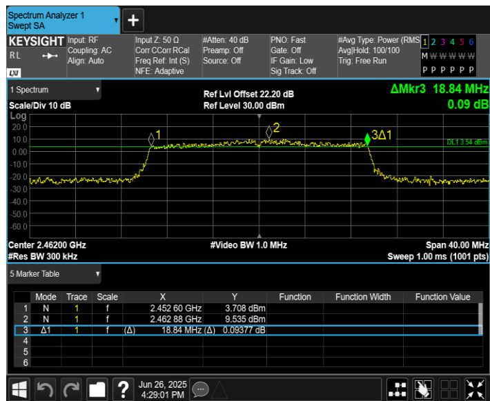
11AX20MIMO_Ant8_2462
