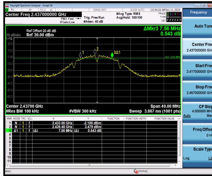
11B-CDD_Ant8_2437
