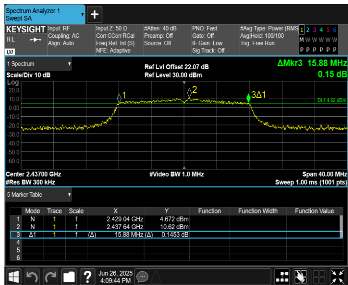
11G-CDD_Ant8_2437
