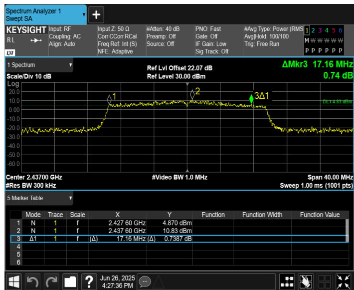
11AX20MIMO_Ant8_2437
