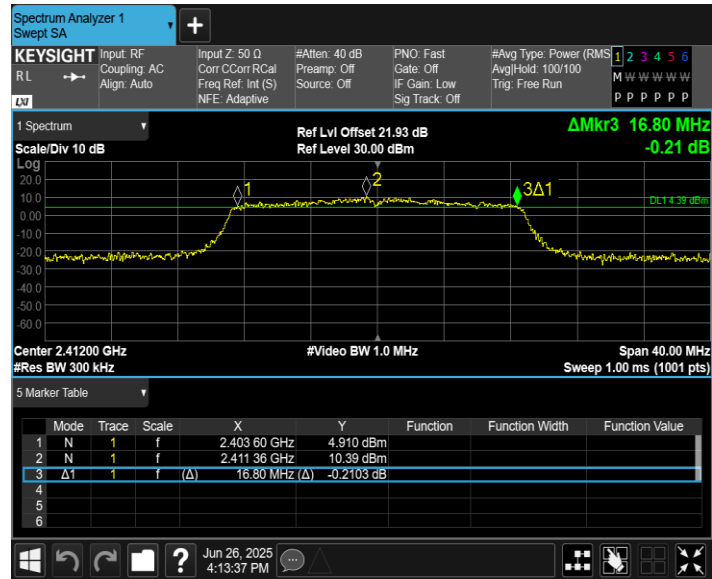
11N20MIMO_Ant8_2412
