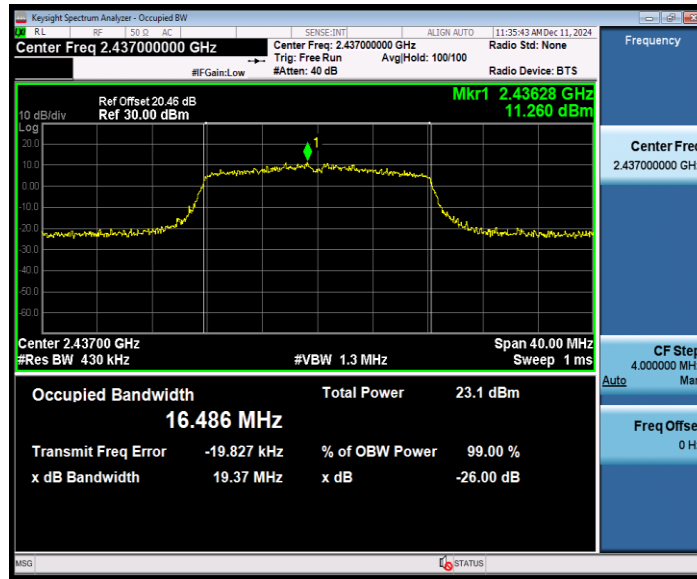
11G-CDD_Ant8_2437
