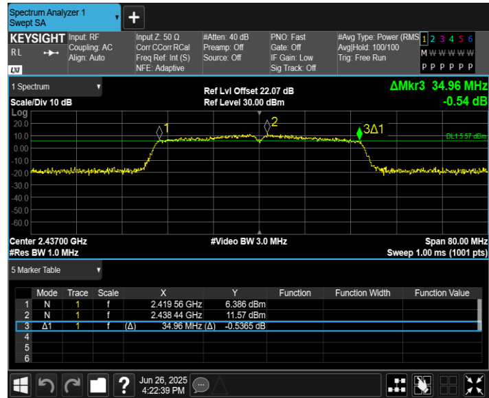
11N40MIMO_Ant8_2437
