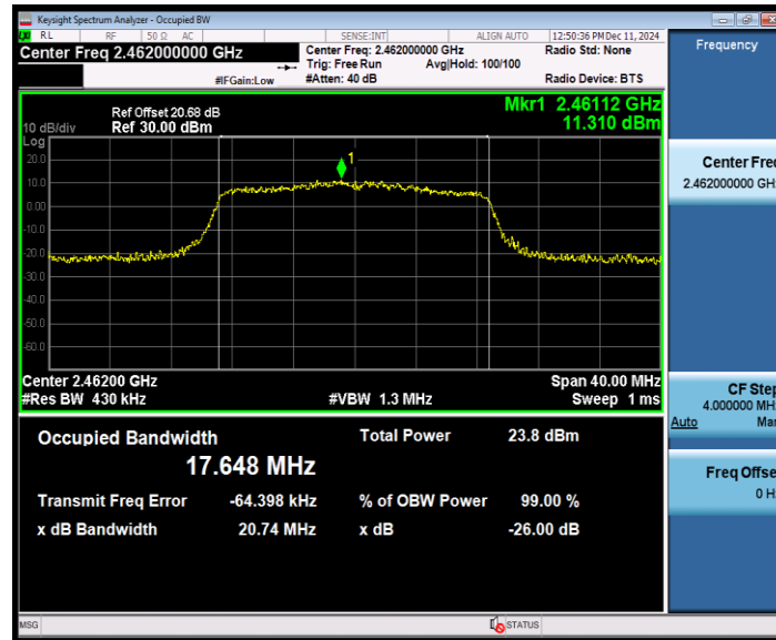
11N20MIMO_Ant8_2462
