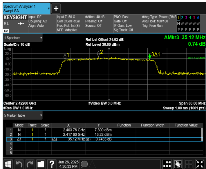
11AX40MIMO_Ant8_2422
