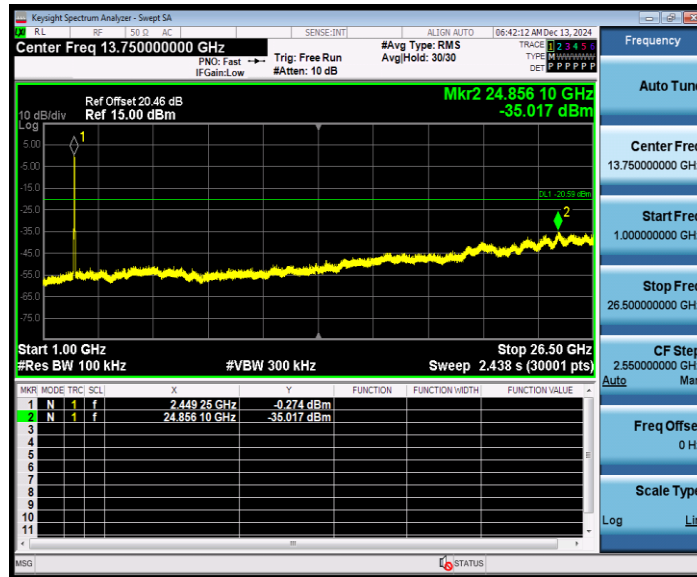
11N40MIMO_Ant8_2452_0~Reference
