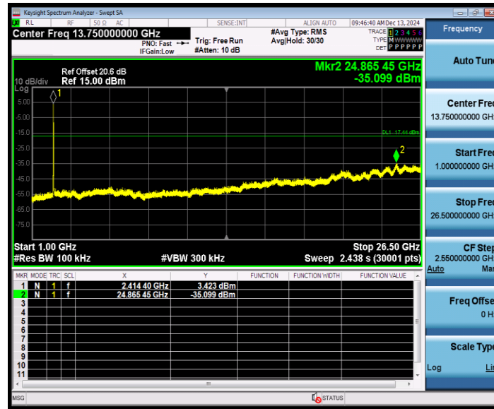
11AX20MIMO_Ant8_2412_0~Reference
