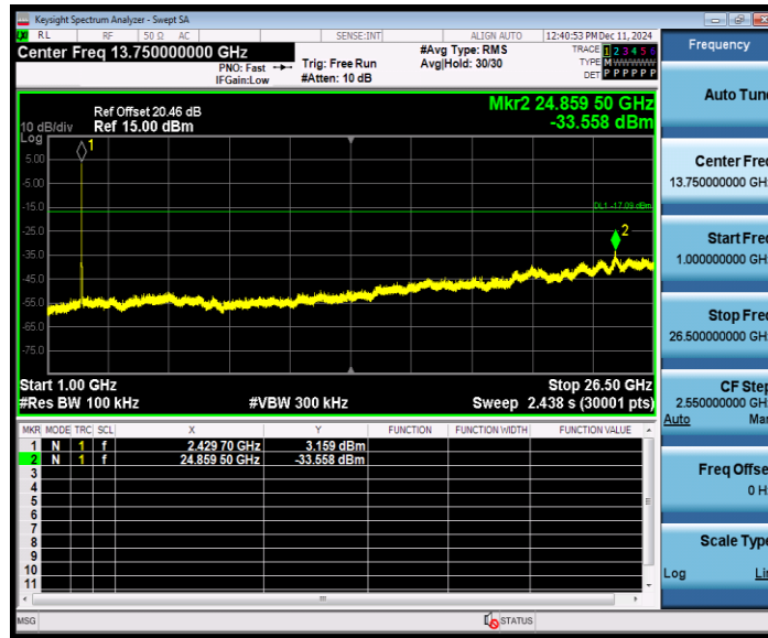
11N20MIMO_Ant8_2437_0~Reference
