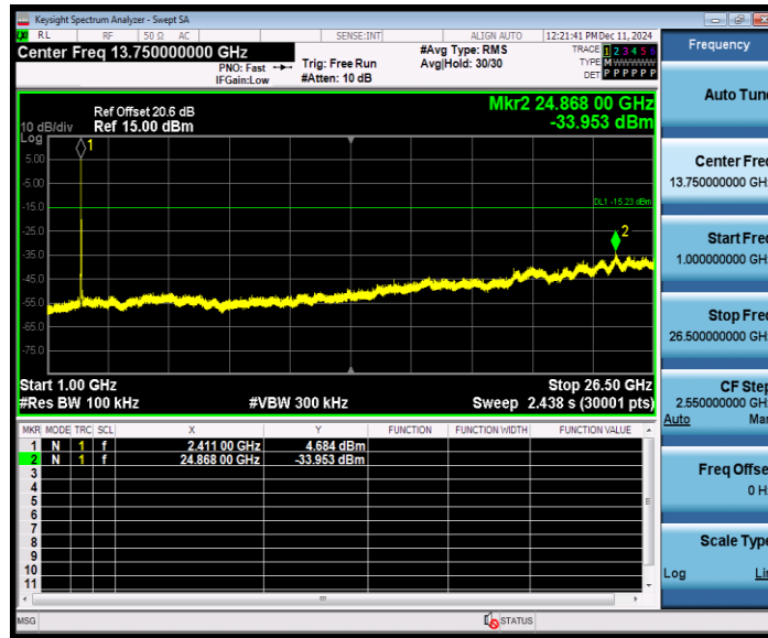
11N20MIMO_Ant8_2412_0~Reference
