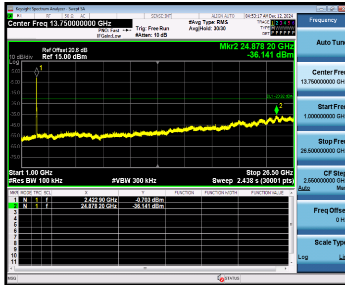
11N40MIMO_Ant8_2422_0~Reference
