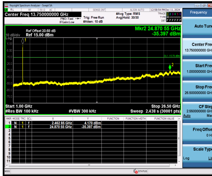
11N20MIMO_Ant8_2462_0~Reference
