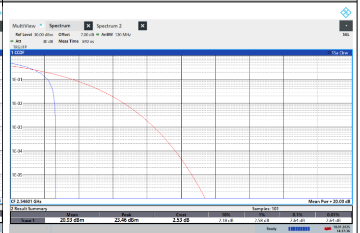
NTNV-N41-PC2-30-100-L-CP-QPSK-Edge_1RB_Left-PASS
