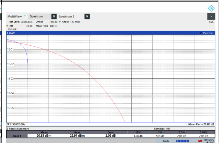
NTNV-N41-PC2-30-80-L-CP-16QPSK-Edge_1RB_Left-PASS
