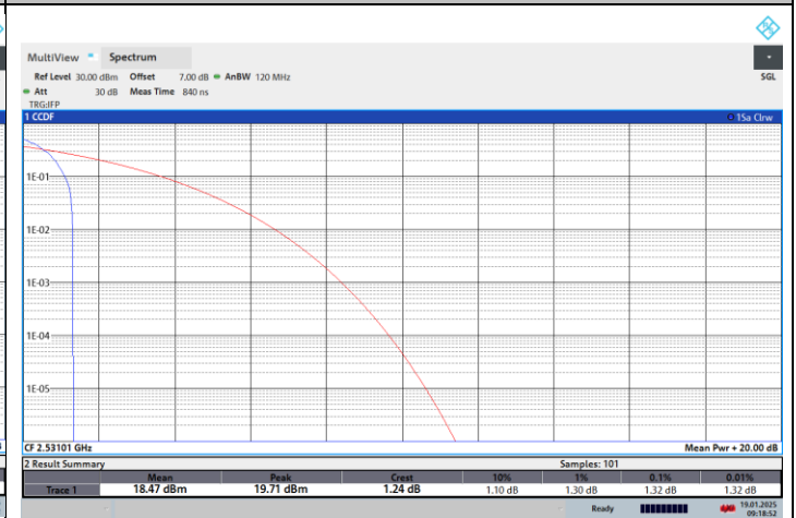
NTNV-N41-PC2-30-70-L-CP-256QPSK-Edge_1RB_Left-PASS
