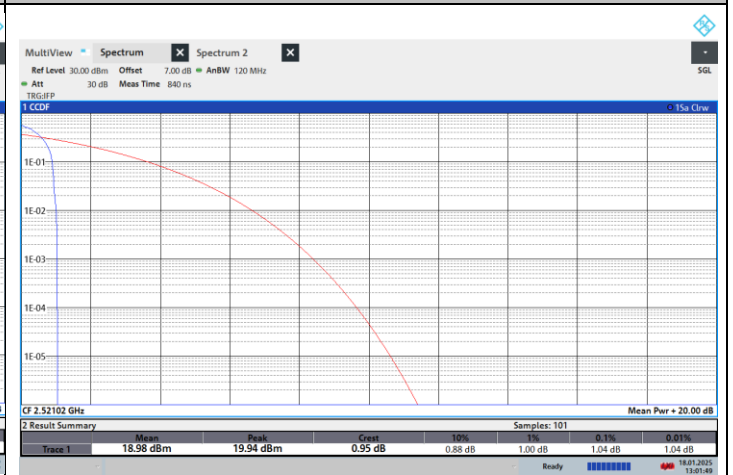
NTNV-N41-PC2-30-50-L-CP-64QPSK-Edge_1RB_Left-PASS
