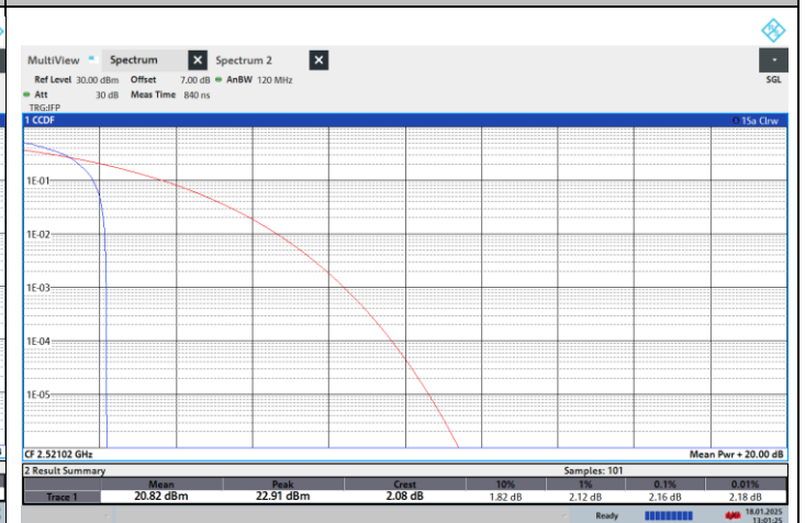
NTNV-N41-PC2-30-50-L-CP-16QPSK-Edge_1RB_Left-PASS
