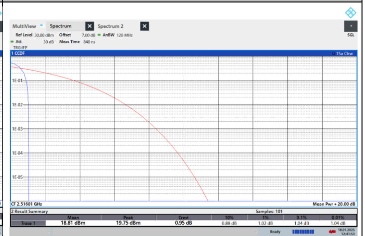
NTNV-N41-PC2-30-40-L-CP-256QPSK-Edge_1RB_Left-PASS
