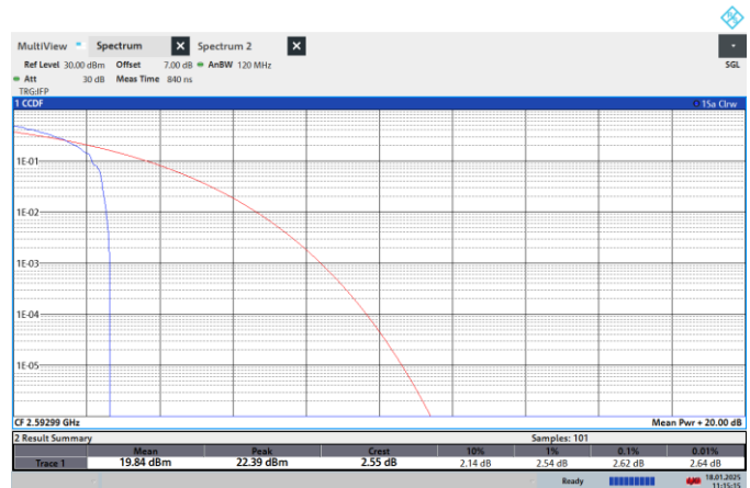
NTN-N41-PC2-30-20-M-CP-64QPSK-Edge_1RB_Left-PASS
