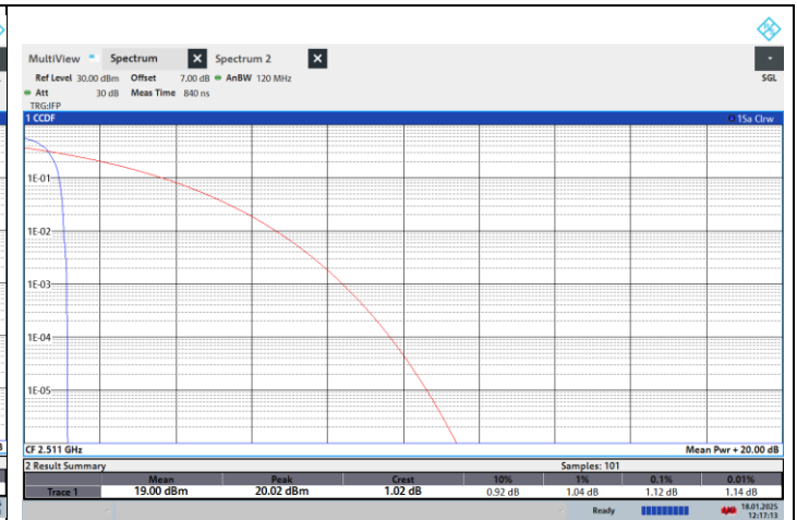
NTNV-N41-PC2-30-30-L-CP-64QPSK-Edge_1RB_Left-PASS
