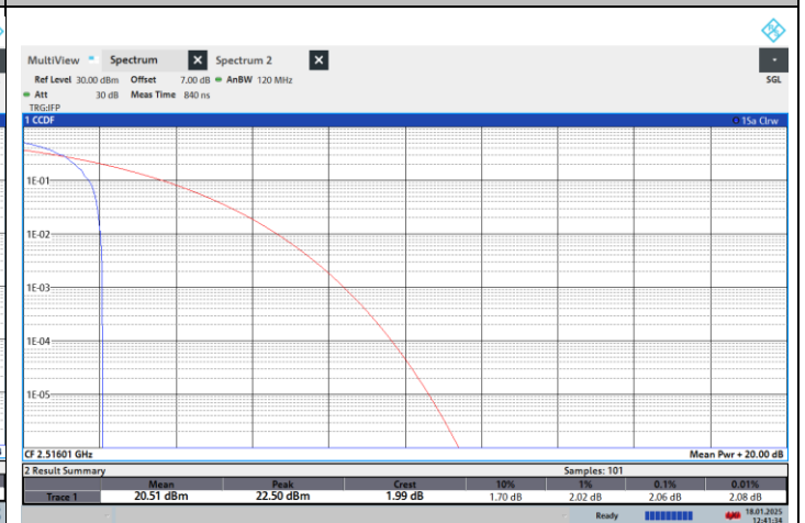
NTNV-N41-PC2-30-40-L-CP-64QPSK-Edge_1RB_Left-PASS
