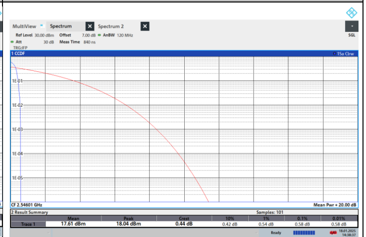
NTNV-N41-PC2-30-100-L-CP-256QPSK-Edge_1RB_Left-PASS
