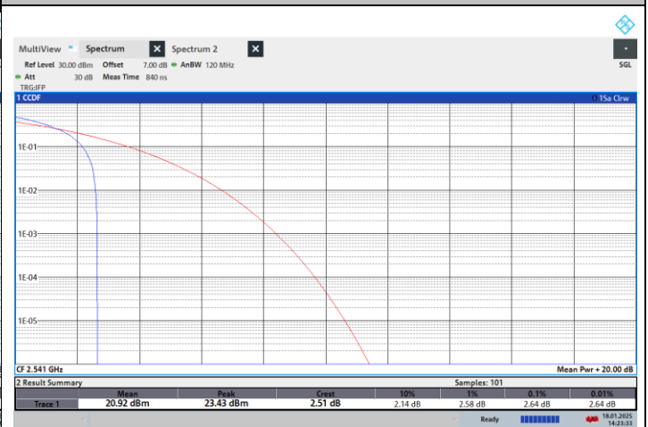
NTN-N41-PC2-30-90-L-CP-QPSK-Edge_1RB_Left-PASS
