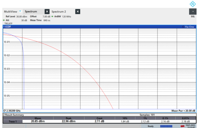
NTNV-N41-PC2-30-40-M-CP-16QPSK-Edge_1RB_Left-PASS
