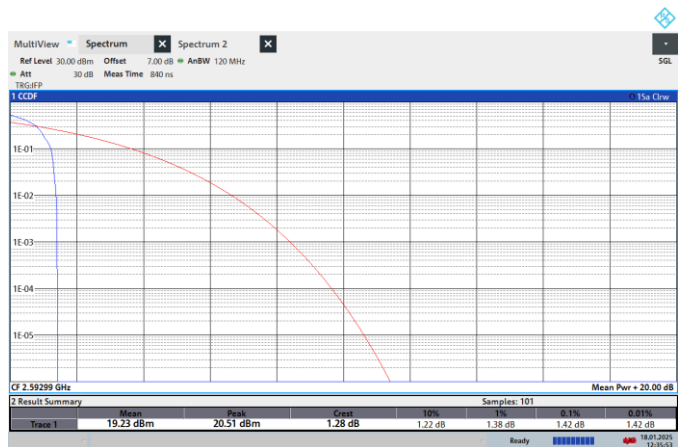
NTNV-N41-PC2-30-40-M-CP-256QPSK-Edge_1RB_Left-PASS
