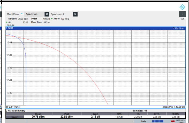
NTN-N41-PC2-30-30-L-CP-QPSK-Edge_1RB_Left-PASS
