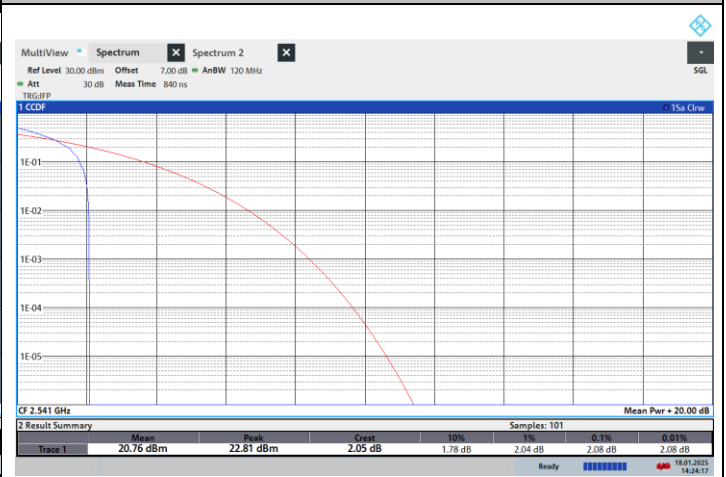
NTN-N41-PC2-30-90-L-CP-16QPSK-Edge_1RB_Left-PASS
