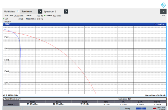
NTNV-N41-PC2-30-30-M-CP-16QPSK-Edge_1RB_Left-PASS
