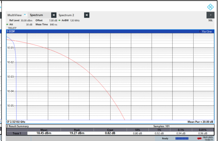
NTN-N41-PC2-30-50-L-CP-256QPSK-Edge_1RB_Left-PASS
