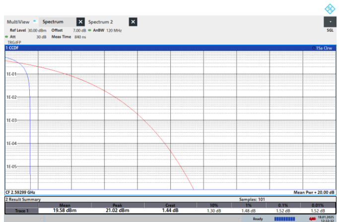
NTNV-N41-PC2-30-40-M-CP-64QPSK-Edge_1RB_Left-PASS
