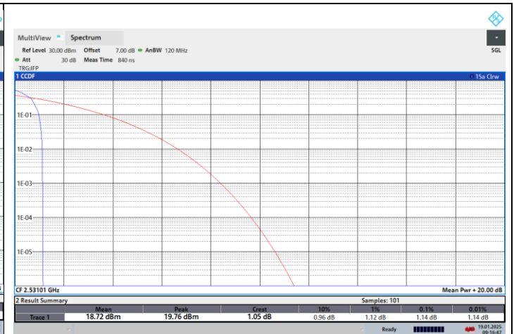
NTNV-N41-PC2-30-70-L-CP-16QPSK-Edge_1RB_Left-PASS
