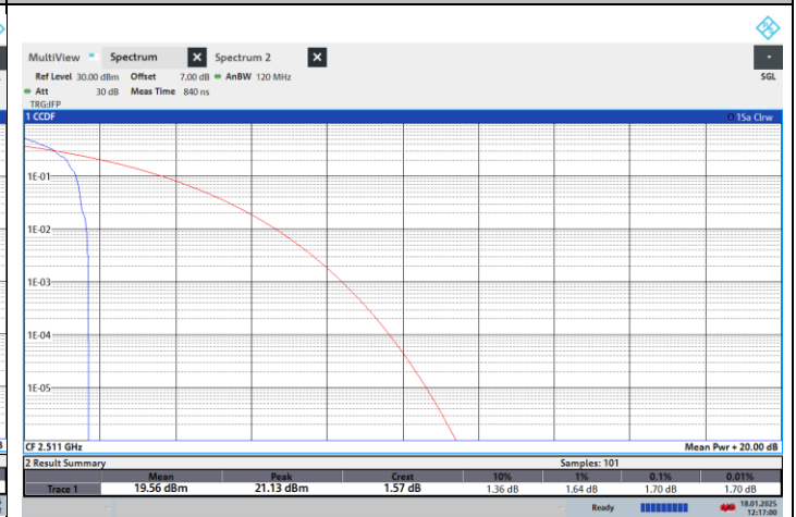
NTN-N41-PC2-30-30-L-CP-16QPSK-Edge_1RB_Left-PASS
