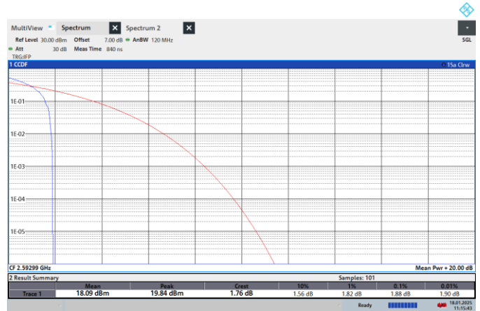
NTNV-N41-PC2-30-20-M-CP-256QPSK-Edge_1RB_Left-PASS
