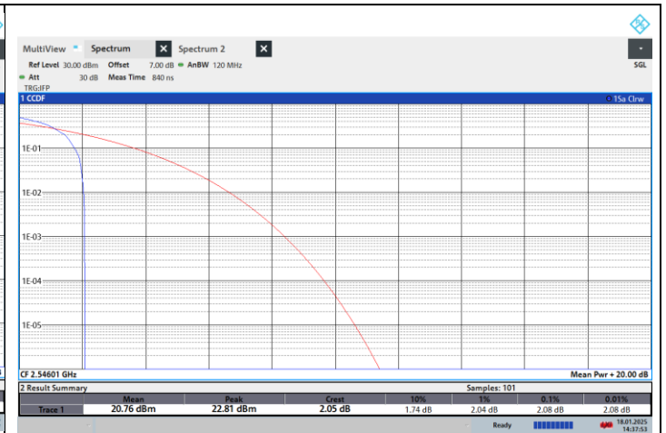
NTNV-N41-PC2-30-100-L-CP-16QPSK-Edge_1RB_Left-PASS
