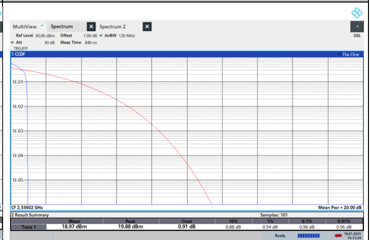
NTNV-N41-PC2-30-80-L-CP-64QPSK-Edge_1RB_Left-PASS
