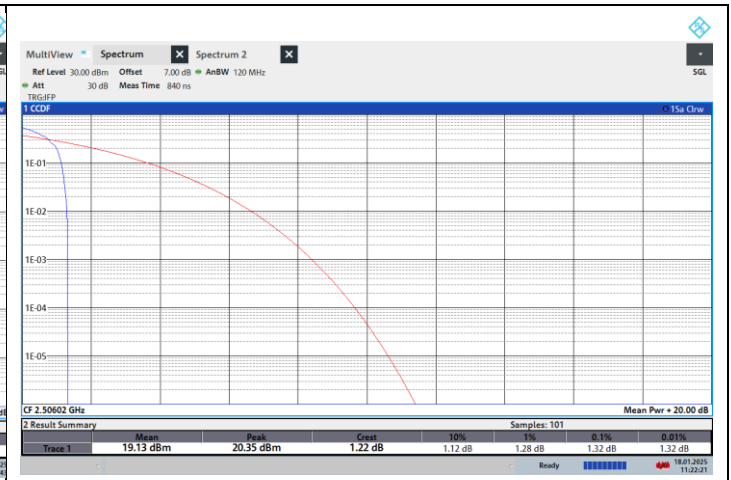
NTN-N41-PC2-30-20-L-CP-256QPSK-Edge_1RB_Left-PASS
