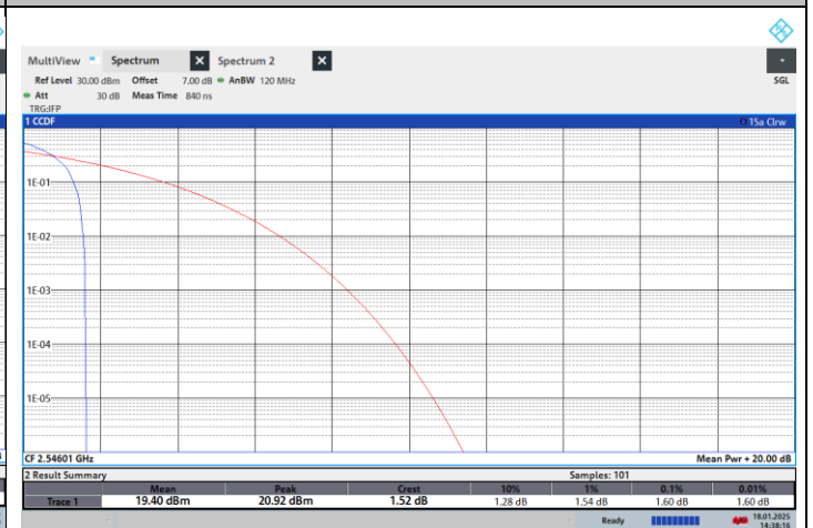
NTNV-N41-PC2-30-100-L-CP-64QPSK-Edge_1RB_Left-PASS
