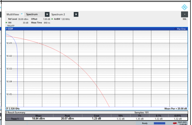
NTNV-N41-PC2-30-60-L-CP-256QPSK-Edge_1RB_Left-PASS
