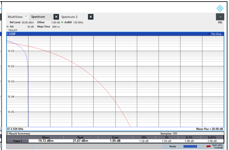
NTNV-N41-PC2-30-60-L-CP-64QPSK-Edge_1RB_Left-PASS
