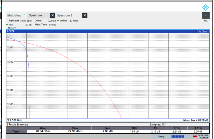
NTN-N41-PC2-30-60-L-CP-16QPSK-Edge_1RB_Left-PASS
