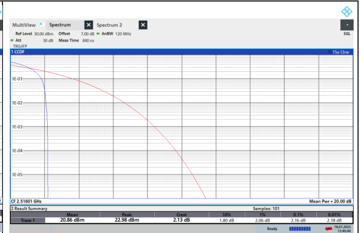
NTNV-N41-PC2-30-40-L-CP-16QPSK-Edge_1RB_Left-PASS
