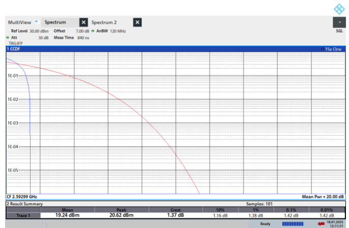
NTNV-N41-PC2-30-30-M-CP-256QPSK-Edge_1RB_Left-PASS
