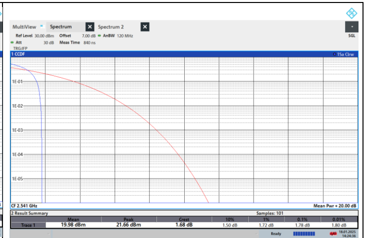
NTNV-N41-PC2-30-90-L-CP-64QPSK-Edge_1RB_Left-PASS
