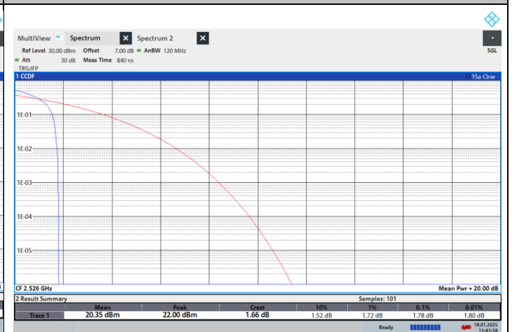
NTN-N41-PC2-30-60-L-CP-QPSK-Edge_1RB_Left-PASS
