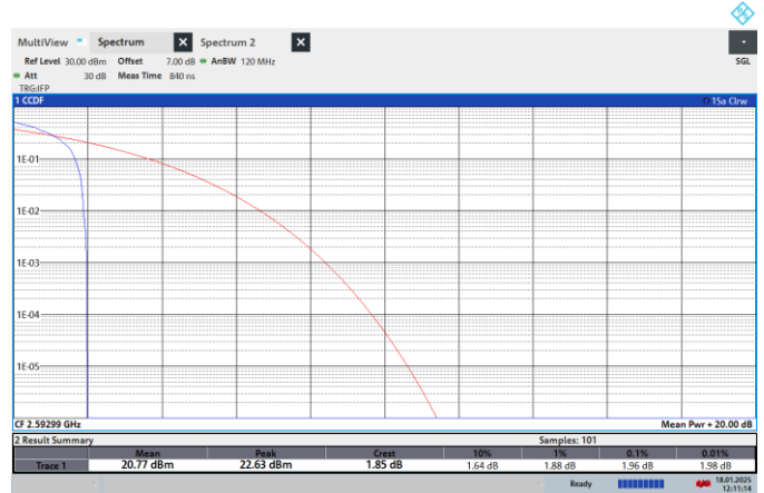
NTNV-N41-PC2-30-30-M-CP-64QPSK-Edge_1RB_Left-PASS
