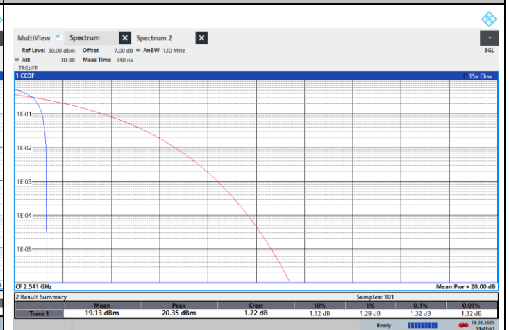
NTNV-N41-PC2-30-90-L-CP-256QPSK-Edge_1RB_Left-PASS
