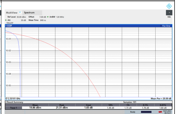
NTNV-N41-PC2-30-70-L-CP-QPSK-Edge_1RB_Left-PASS
