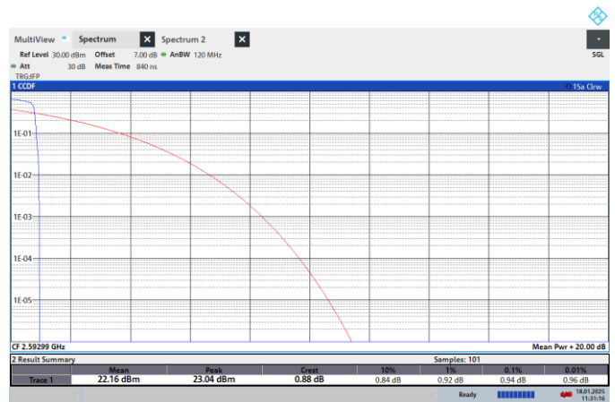
NTNV-N41-PC2-30-30-M-CP-QPSK-Edge_1RB_Left-PASS
