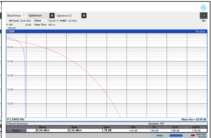
NTNV-N41-PC2-30-80-L-CP-QPSK-Edge_1RB_Left-PASS
