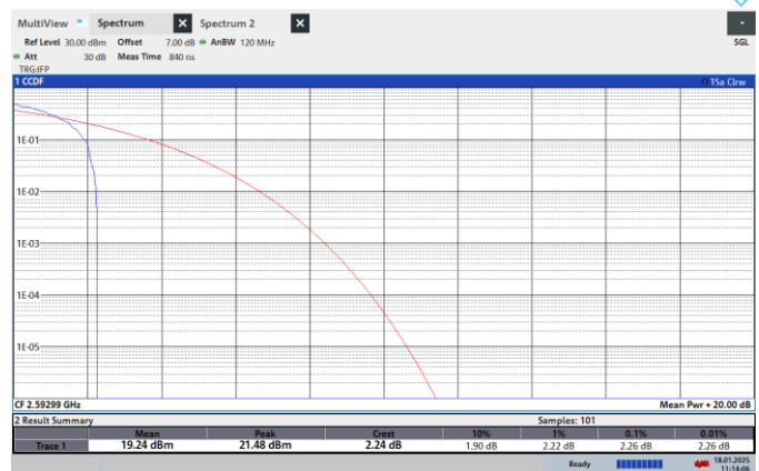
NTN-N41-PC2-30-20-M-CP-16QPSK-Edge_1RB_Left-PASS
