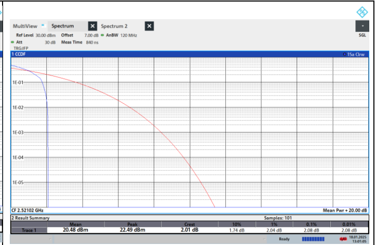
NTNV-N41-PC2-30-50-L-CP-QPSK-Edge_1RB_Left-PASS
