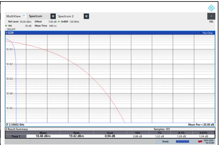
NTN-N41-PC2-30-80-L-CP-256QPSK-Edge_1RB_Left-PASS
