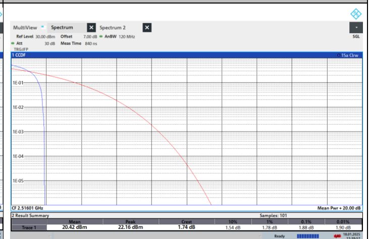
NTNV-N41-PC2-30-40-L-CP-QPSK-Edge_1RB_Left-PASS
