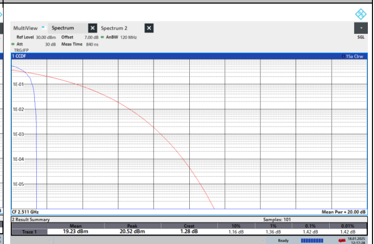
NTNV-N41-PC2-30-30-L-CP-256QPSK-Edge_1RB_Left-PASS
