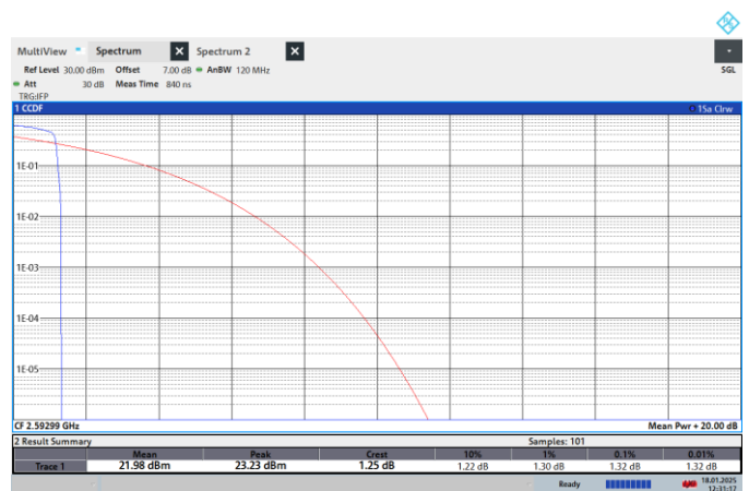
NTNV-N41-PC2-30-40-M-CP-QPSK-Edge_1RB_Left-PASS
