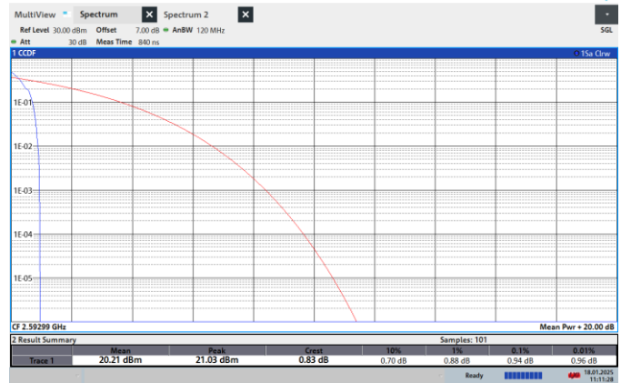
NTN-N41-PC2-30-20-M-CP-QPSK-Edge_1RB_Left-PASS
