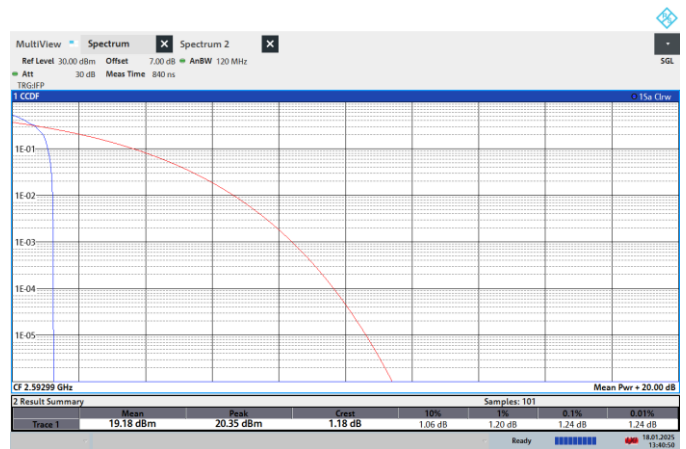
NTNV-N41-PC2-30-60-M-CP-256QPSK-Edge_1RB_Left-PASS
