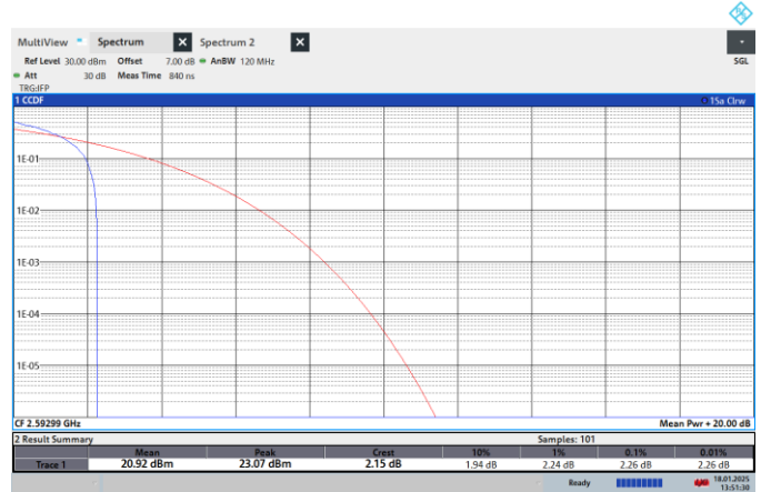
NTNV-N41-PC2-30-70-M-CP-16QPSK-Edge_1RB_Left-PASS
