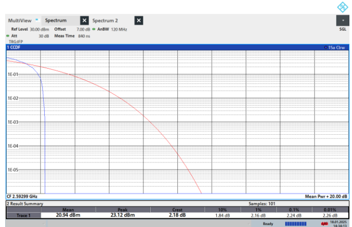
NTNV-N41-PC2-30-100-M-CP-16QPSK-Edge_1RB_Left-PASS
