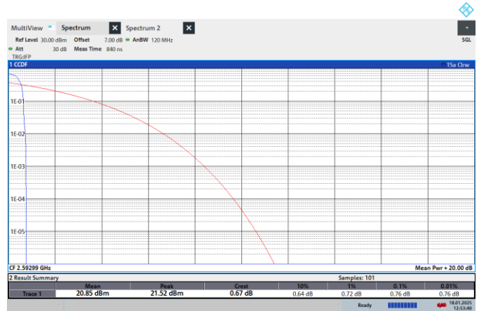
NTN-N41-PC2-30-50-M-CP-QPSK-Edge_1RB_Left-PASS
