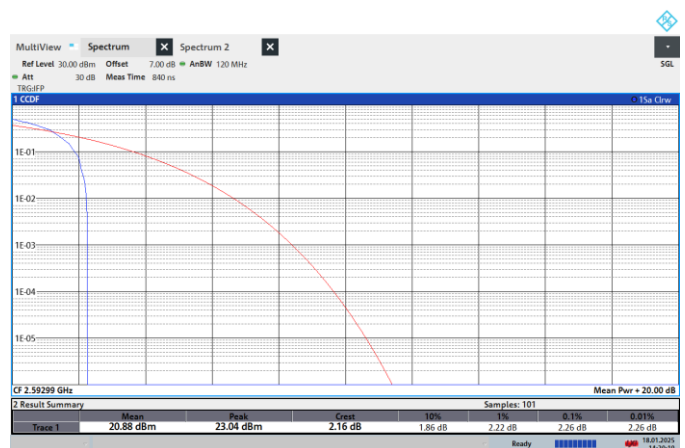
NTNV-N41-PC2-30-90-M-CP-16QPSK-Edge_1RB_Left-PASS
