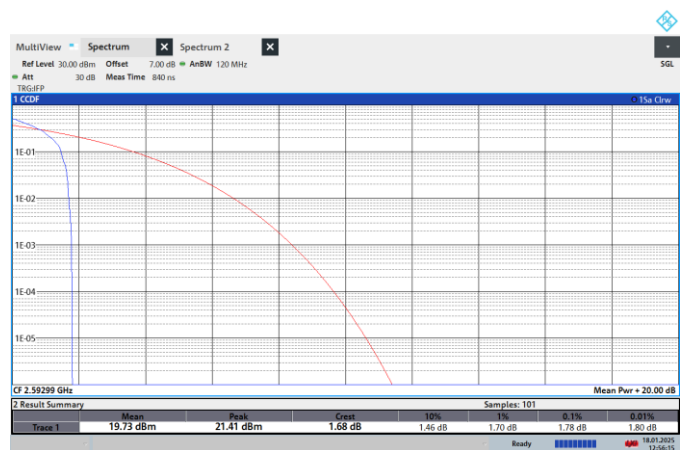
NTN-N41-PC2-30-50-M-CP-64QPSK-Edge_1RB_Left-PASS
