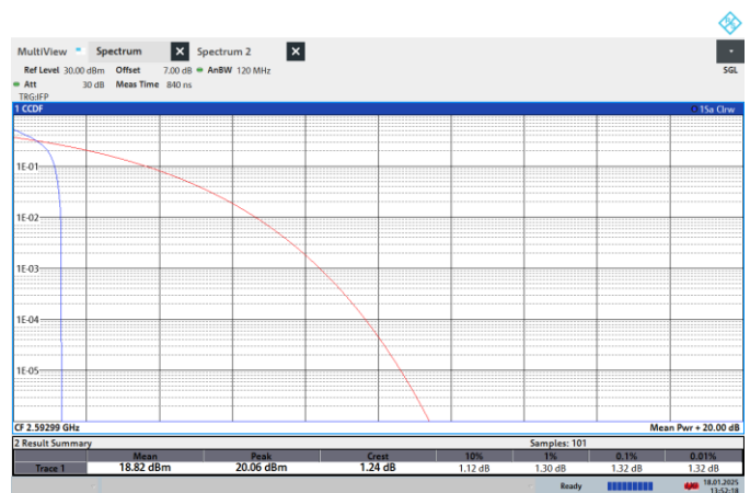
NTNV-N41-PC2-30-70-M-CP-256QPSK-Edge_1RB_Left-PASS
