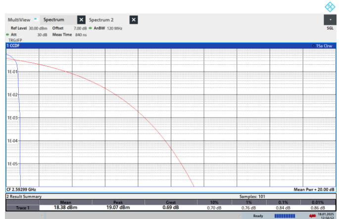
NTNV-N41-PC2-30-50-M-CP-256QPSK-Edge_1RB_Left-PASS
