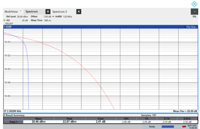
NTNV-N41-PC2-30-60-M-CP-64QPSK-Edge_1RB_Left-PASS
