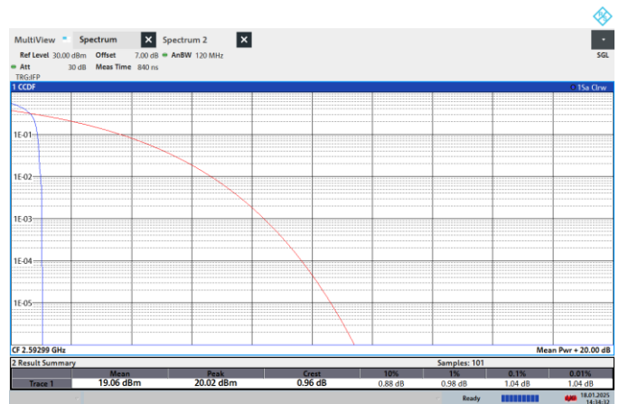
NTNV-N41-PC2-30-100-M-CP-64QPSK-Edge_1RB_Left-PASS
