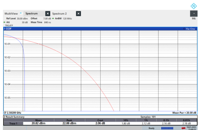
NTNV-N41-PC2-30-60-M-CP-16QPSK-Edge_1RB_Left-PASS
