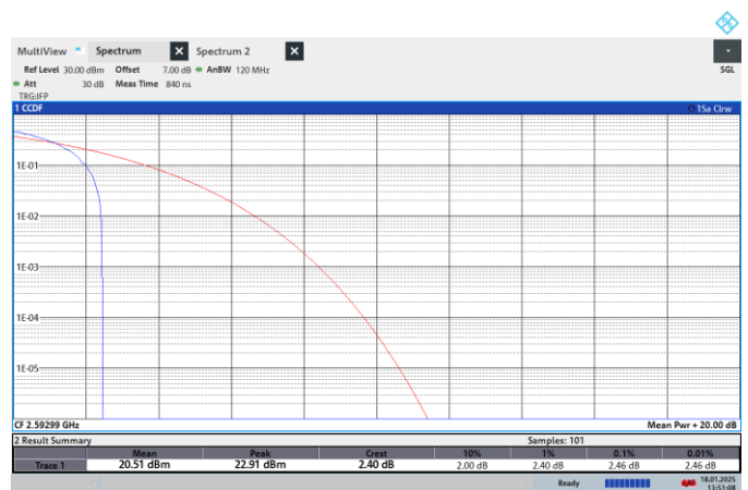
NTNV-N41-PC2-30-70-M-CP-QPSK-Edge_1RB_Left-PASS
