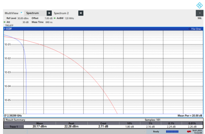
NTNV-N41-PC2-30-70-M-CP-64QPSK-Edge_1RB_Left-PASS
