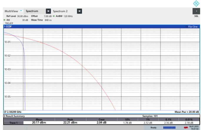
NTN-N41-PC2-30-80-M-CP-QPSK-Edge_1RB_Left-PASS
