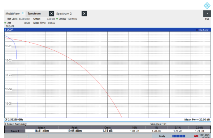
NTNV-N41-PC2-30-90-M-CP-256QPSK-Edge_1RB_Left-PASS
