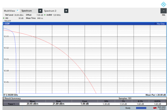
NTN-N41-PC2-30-50-M-CP-16QPSK-Edge_1RB_Left-PASS
