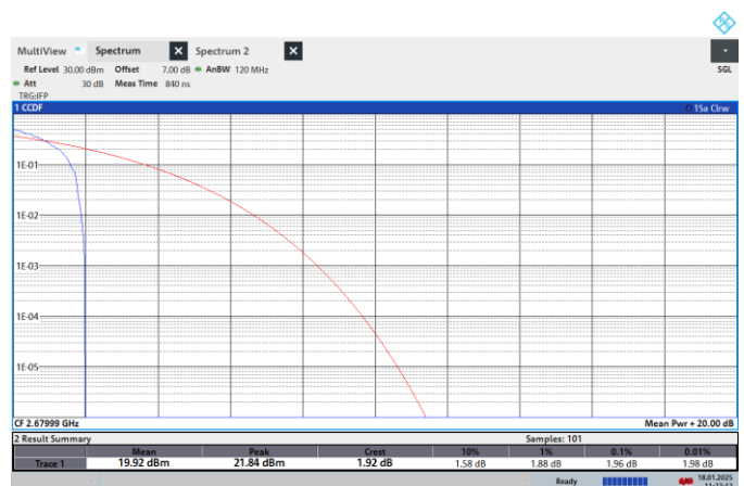
NTNV-N41-PC2-30-20-H-CP-64QPSK-Edge_1RB_Left-PASS
