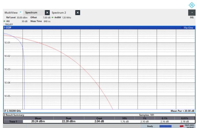
NTNV-N41-PC2-30-90-M-CP-QPSK-Edge_1RB_Left-PASS
