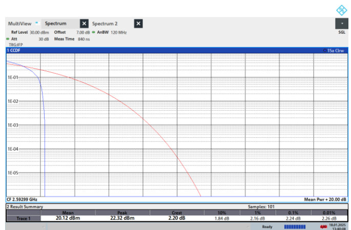
NTNV-N41-PC2-30-60-M-CP-QPSK-Edge_1RB_Left-PASS
