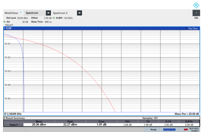
NTN-N41-PC2-30-80-M-CP-16QPSK-Edge_1RB_Left-PASS
