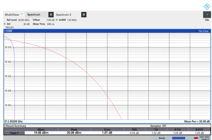
NTN-N41-PC2-30-80-M-CP-64QPSK-Edge_1RB_Left-PASS
