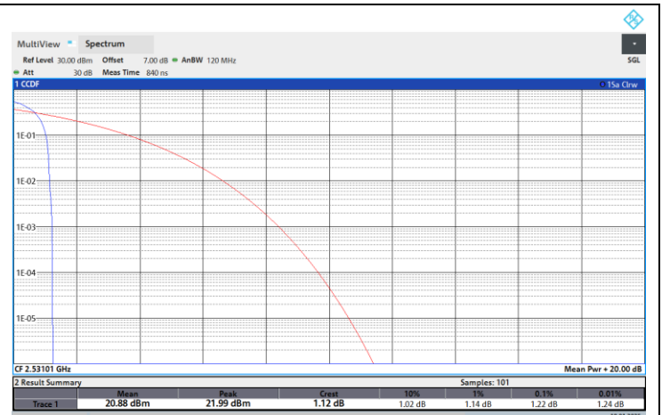
NTNV-N41-PC2-30-70-L-CP-16QPSK-Edge_1RB_Left-PASS
