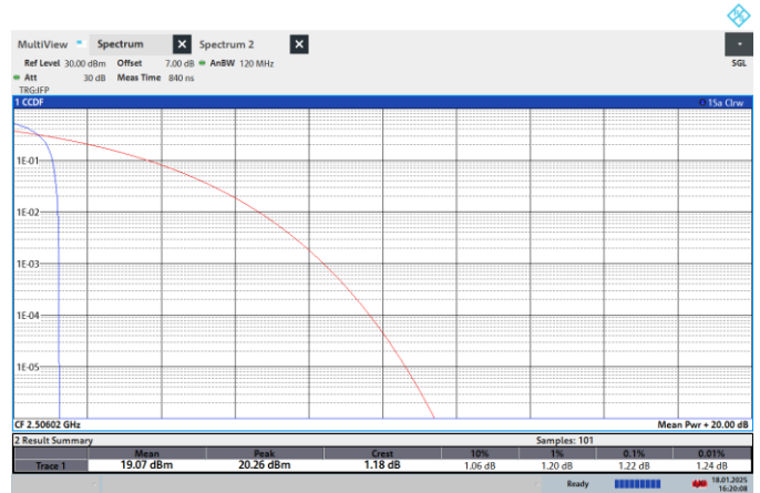
NTNV-N41-PC2-30-20-L-CP-256QPSK-Edge_1RB_Left-PASS
