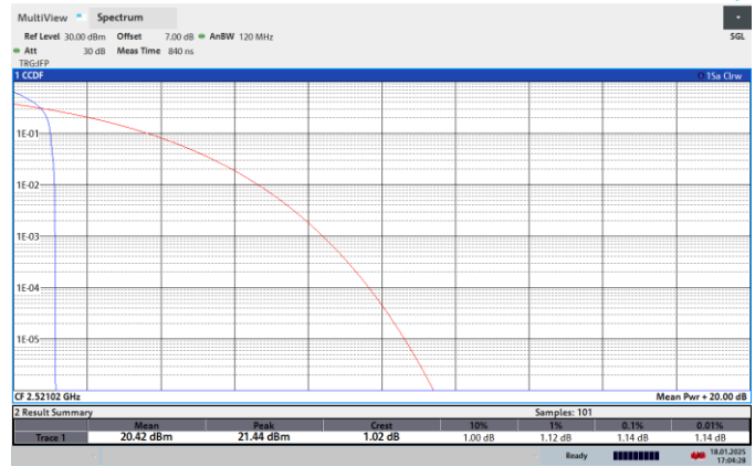
NTNV-N41-PC2-30-50-L-CP-QPSK-Edge_1RB_Left-PASS
