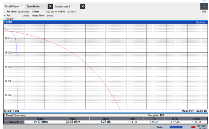
NTNV-N41-PC2-30-30-L-CP-256QPSK-Edge_1RB_Left-PASS
