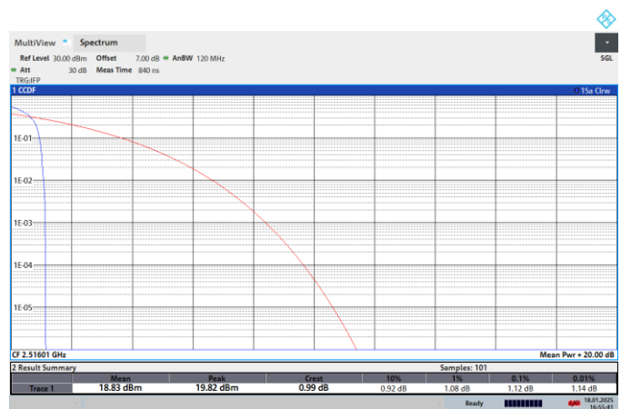
NTNV-N41-PC2-30-40-L-CP-256QPSK-Edge_1RB_Left-PASS
