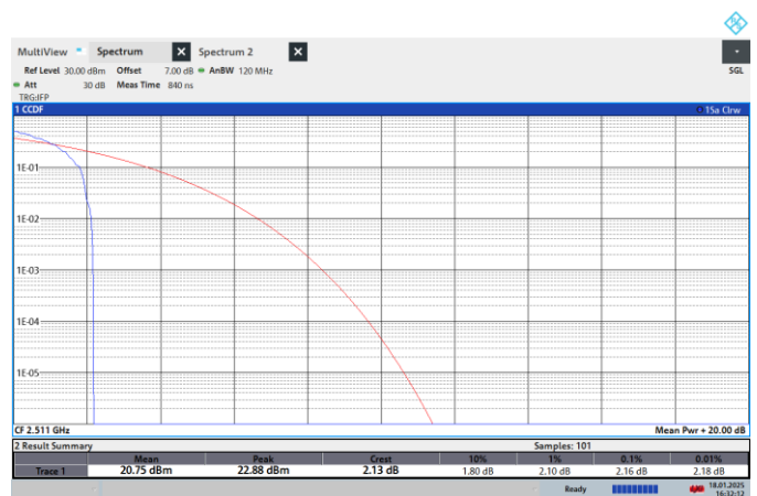
NTNV-N41-PC2-30-30-L-CP-16QPSK-Edge_1RB_Left-PASS
