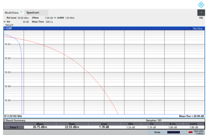
NTNV-N41-PC2-30-50-L-CP-64QPSK-Edge_1RB_Left-PASS
