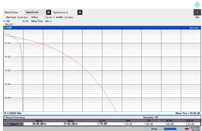
NTNV-N41-PC2-30-20-L-CP-QPSK-Edge_1RB_Left-PASS
