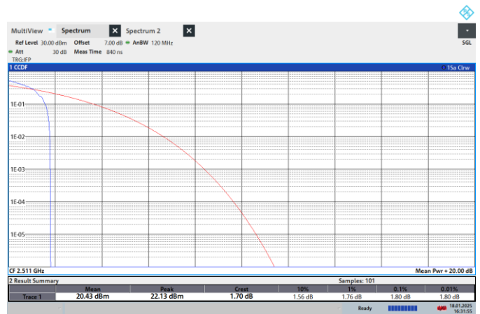
NTNV-N41-PC2-30-30-L-CP-QPSK-Edge_1RB_Left-PASS
