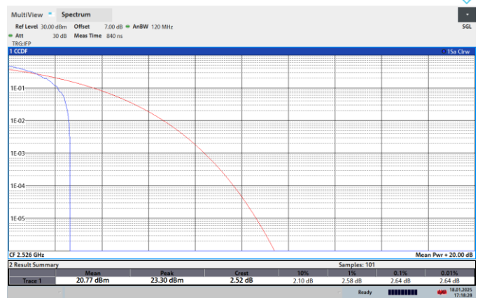
NTNV-N41-PC2-30-60-L-CP-QPSK-Edge_1RB_Left-PASS
