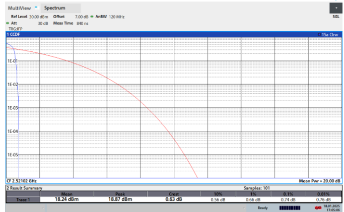
NTNV-N41-PC2-30-50-L-CP-256QPSK-Edge_1RB_Left-PASS
