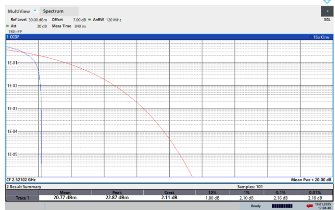
NTNV-N41-PC2-30-50-L-CP-16QPSK-Edge_1RB_Left-PASS
