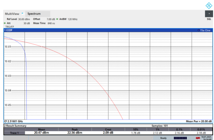
NTNV-N41-PC2-30-40-L-CP-QPSK-Edge_1RB_Left-PASS
