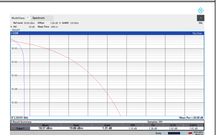
NTNV-N41-PC2-30-70-L-CP-256QPSK-Edge_1RB_Left-PASS
