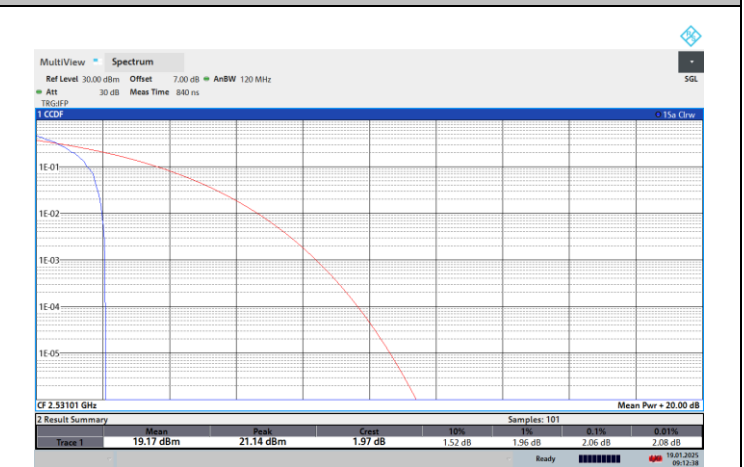
NTNV-N41-PC2-30-70-L-CP-64QPSK-Edge_1RB_Left-PASS
