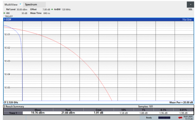
NTNV-N41-PC2-30-60-L-CP-64QPSK-Edge_1RB_Left-PASS
