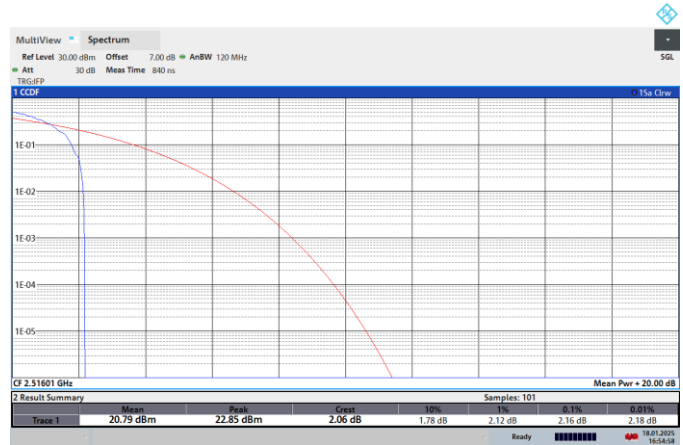
NTNV-N41-PC2-30-40-L-CP-16QPSK-Edge_1RB_Left-PASS
