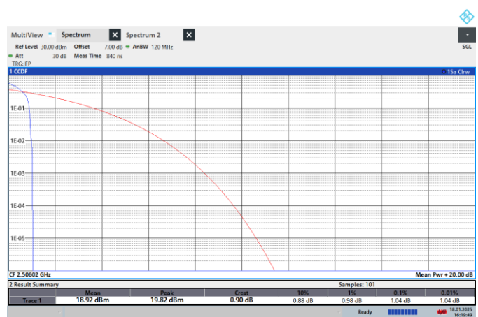
NTNV-N41-PC2-30-20-L-CP-64QPSK-Edge_1RB_Left-PASS
