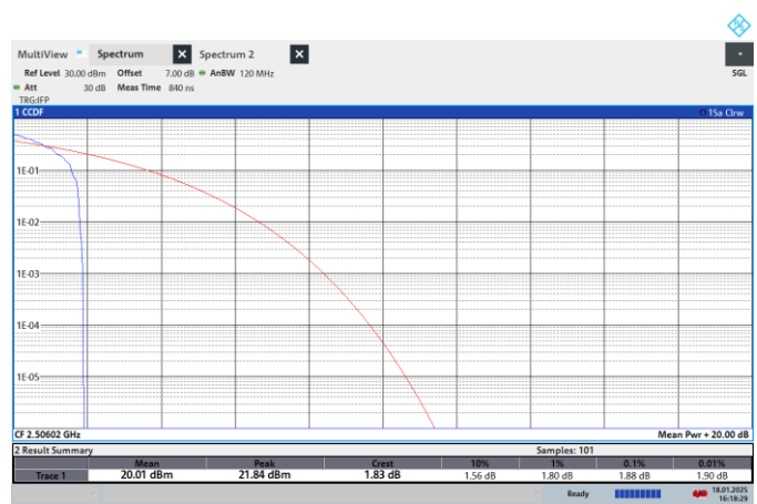
NTNV-N41-PC2-30-20-L-CP-16QPSK-Edge_1RB_Left-PASS
