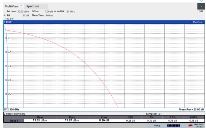
NTNV-N41-PC2-30-60-L-CP-256QPSK-Edge_1RB_Left-PASS
