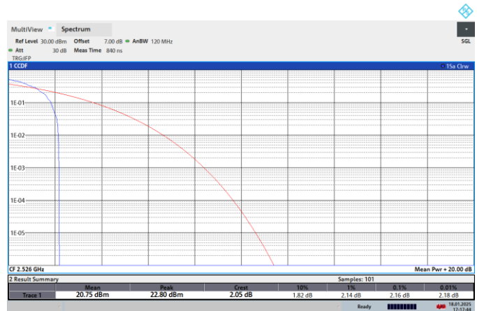
NTNV-N41-PC2-30-60-L-CP-16QPSK-Edge_1RB_Left-PASS
