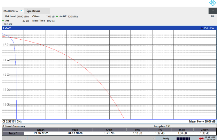
NTNV-N41-PC2-30-70-L-CP-QPSK-Edge_1RB_Left-PASS
