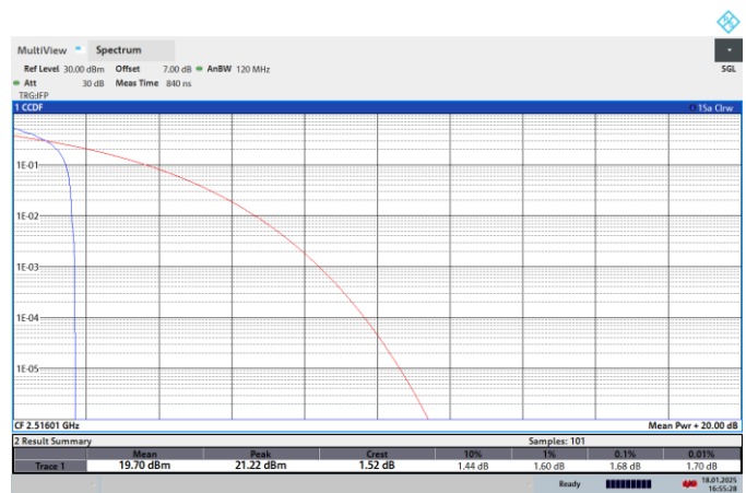
NTNV-N41-PC2-30-40-L-CP-64QPSK-Edge_1RB_Left-PASS
