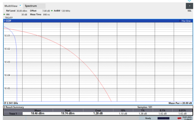
NTNV-N41-PC2-30-90-L-CP-256QPSK-Edge_1RB_Left-PASS
