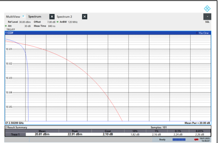
NTNV-N41-PC2-30-40-M-CP-16QPSK-Edge_1RB_Left-PASS
