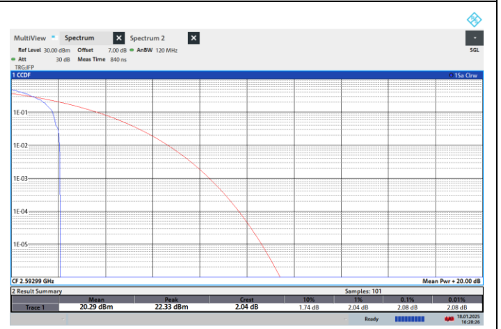
NTNV-N41-PC2-30-30-M-CP-16QPSK-Edge_1RB_Left-PASS
