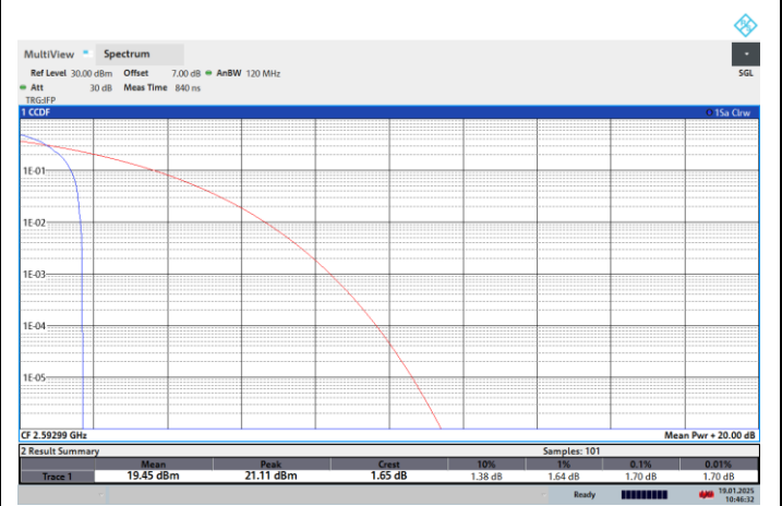
NTNV-N41-PC2-30-80-M-CP-16QPSK-Edge_1RB_Left-PASS
