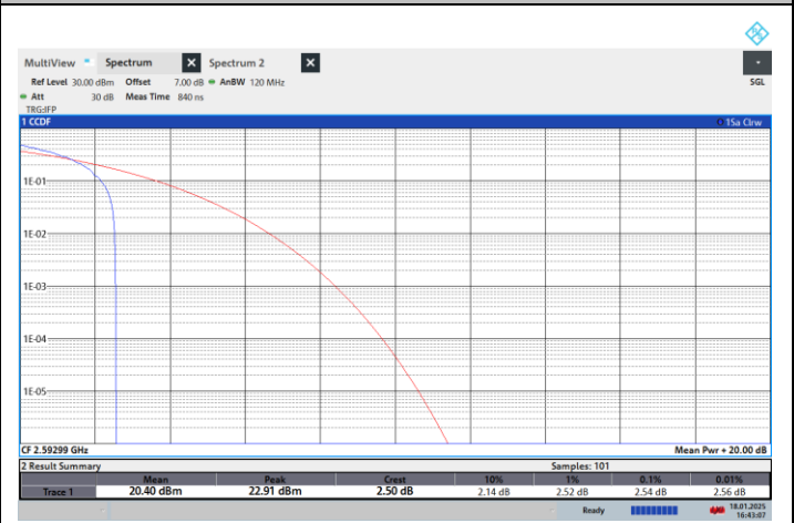
NTNV-N41-PC2-30-40-M-CP-QPSK-Edge_1RB_Left-PASS
