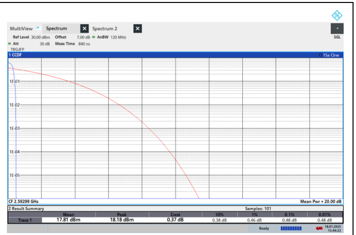
NTNV-N41-PC2-30-20-M-CP-256QPSK-Edge_1RB_Left-PASS
