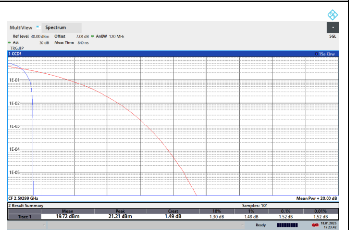
NTNV-N41-PC2-30-70-M-CP-64QPSK-Edge_1RB_Left-PASS
