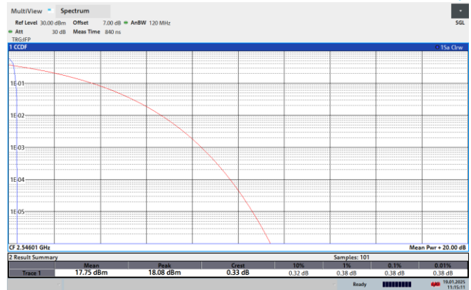
NTNV-N41-PC2-30-100-L-CP-16QPSK-Edge_1RB_Left-PASS
