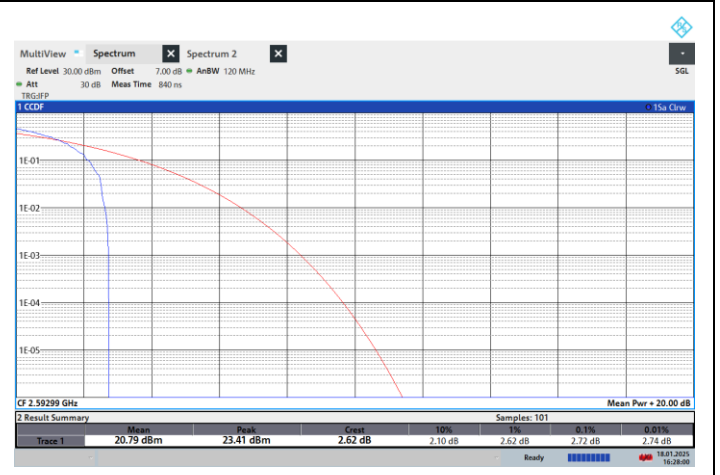
NTNV-N41-PC2-30-30-M-CP-QPSK-Edge_1RB_Left-PASS
