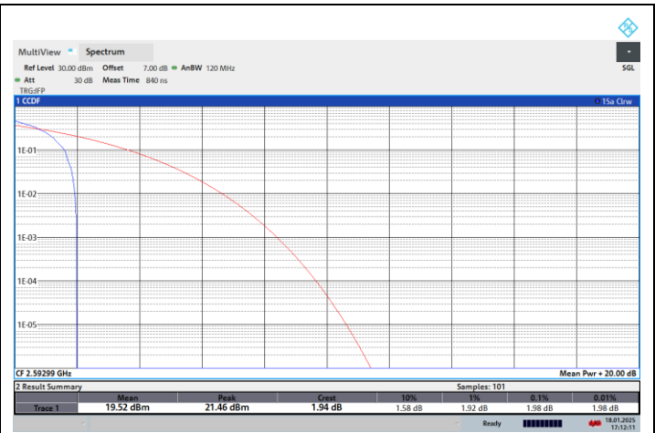
NTNV-N41-PC2-30-60-M-CP-64QPSK-Edge_1RB_Left-PASS
