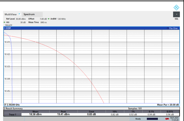
NTNV-N41-PC2-30-70-M-CP-256QPSK-Edge_1RB_Left-PASS
