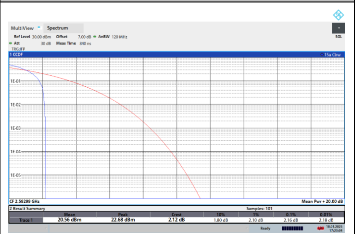
NTNV-N41-PC2-30-70-M-CP-QPSK-Edge_1RB_Left-PASS
