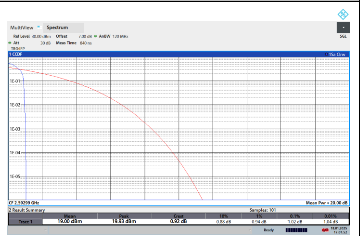
NTNV-N41-PC2-30-50-M-CP-64QPSK-Edge_1RB_Left-PASS
