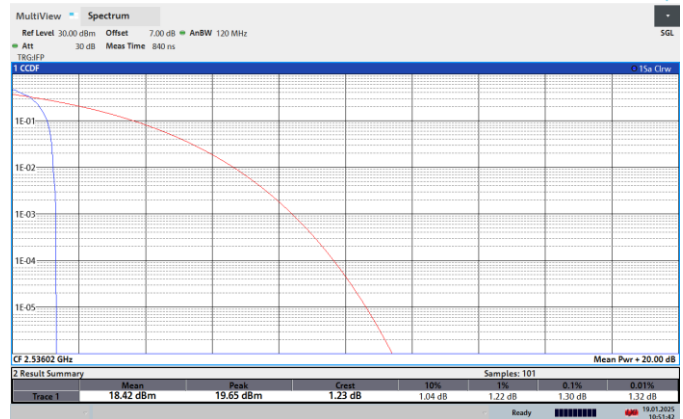
NTNV-N41-PC2-30-80-L-CP-256QPSK-Edge_1RB_Left-PASS
