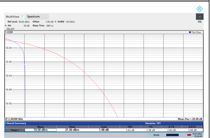
NTNV-N41-PC2-30-40-M-CP-64QPSK-Edge_1RB_Left-PASS
