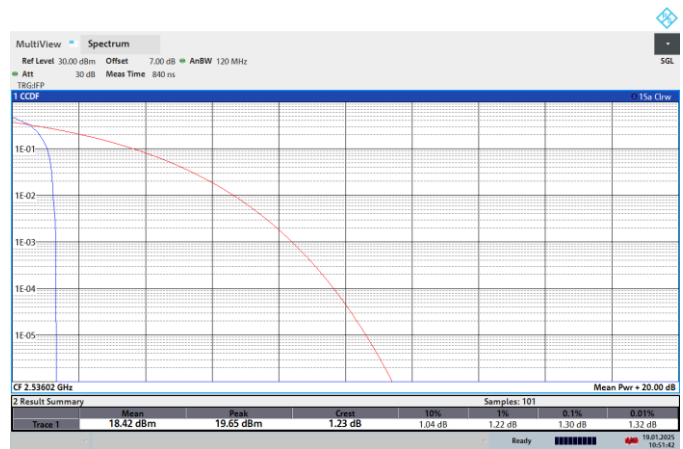
NTNV-N41-PC2-30-80-L-CP-16QPSK-Edge_1RB_Left-PASS
