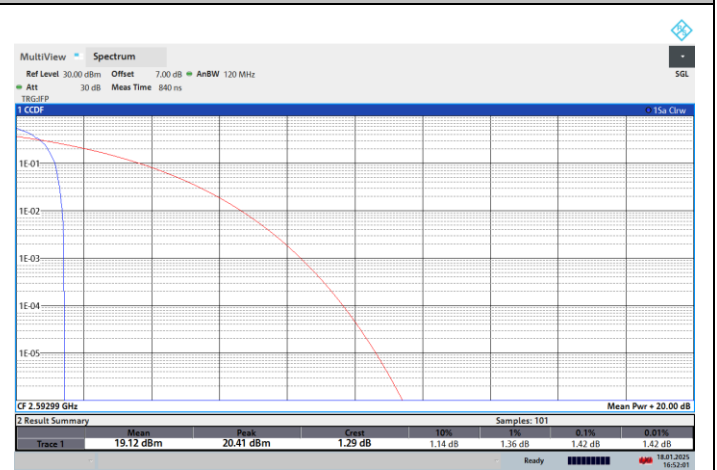
NTNV-N41-PC2-30-40-M-CP-256QPSK-Edge_1RB_Left-PASS
