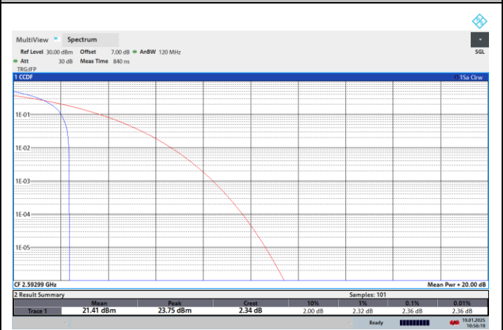
NTNV-N41-PC2-30-90-M-CP-QPSK-Edge_1RB_Left-PASS
