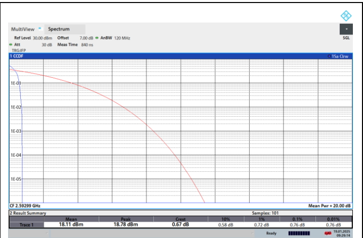
NTNV-N41-PC2-30-80-M-CP-QPSK-Edge_1RB_Left-PASS
