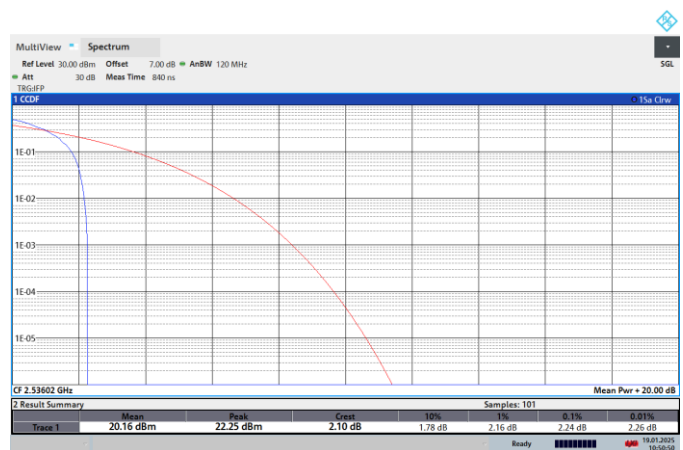
NTNV-N41-PC2-30-80-L-CP-64QPSK-Edge_1RB_Left-PASS
