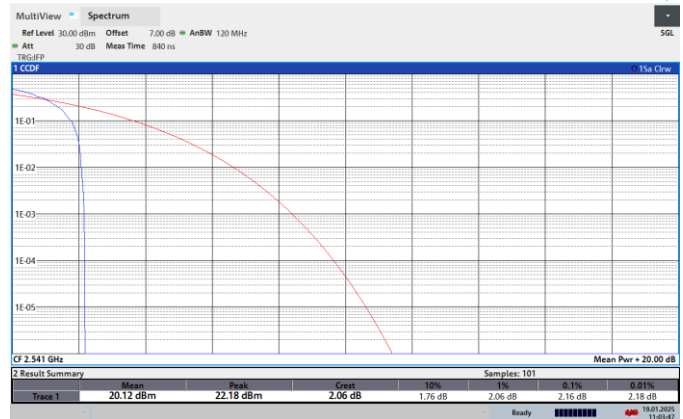
NTNV-N41-PC2-30-90-L-CP-64QPSK-Edge_1RB_Left-PASS
