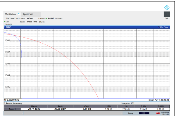
NTNV-N41-PC2-30-70-M-CP-16QPSK-Edge_1RB_Left-PASS
