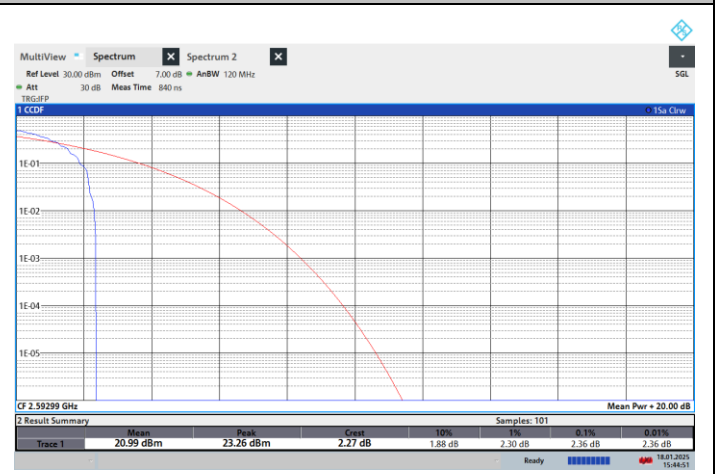
NTNV-N41-PC2-30-20-M-CP-16QPSK-Edge_1RB_Left-PASS
