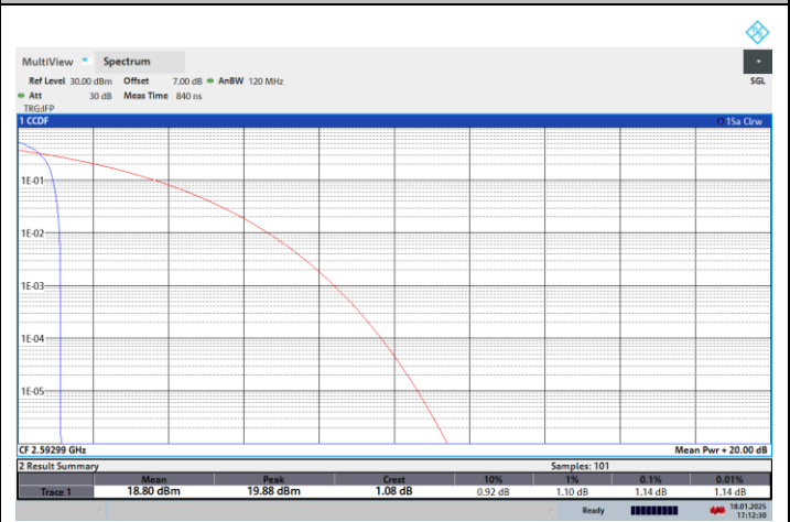
NTNV-N41-PC2-30-60-M-CP-256QPSK-Edge_1RB_Left-PASS
