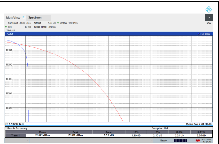
NTNV-N41-PC2-30-50-M-CP-QPSK-Edge_1RB_Left-PASS
