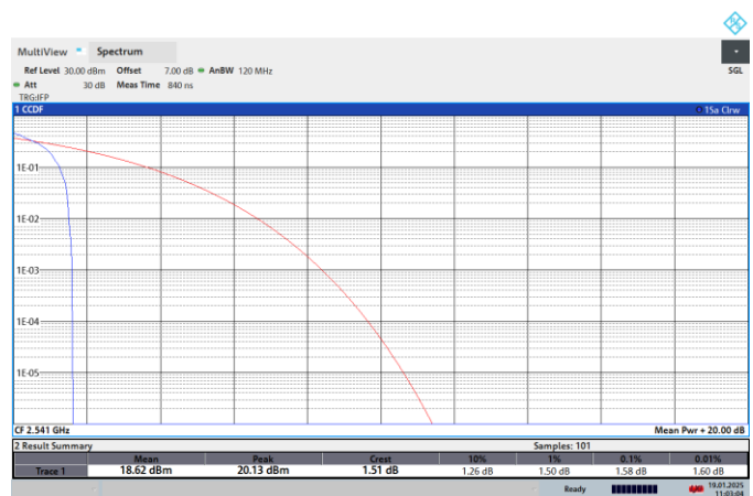
NTNV-N41-PC2-30-90-L-CP-16QPSK-Edge_1RB_Left-PASS
