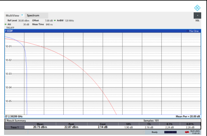
NTNV-N41-PC2-30-50-M-CP-16QPSK-Edge_1RB_Left-PASS
