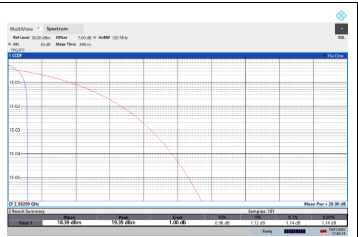
NTNV-N41-PC2-30-50-M-CP-256QPSK-Edge_1RB_Left-PASS
