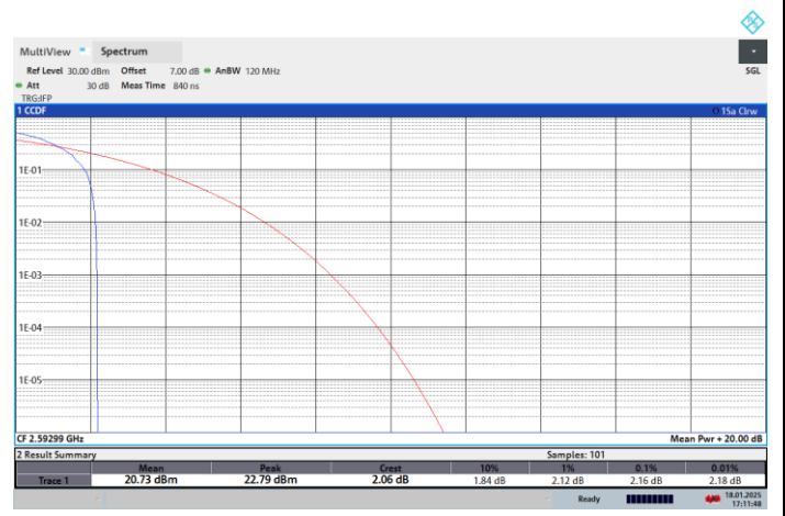
NTNV-N41-PC2-30-60-M-CP-16QPSK-Edge_1RB_Left-PASS
