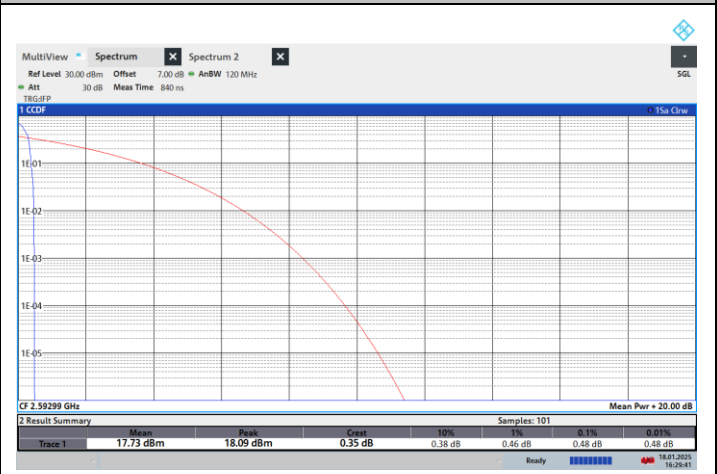
NTNV-N41-PC2-30-30-M-CP-256QPSK-Edge_1RB_Left-PASS
