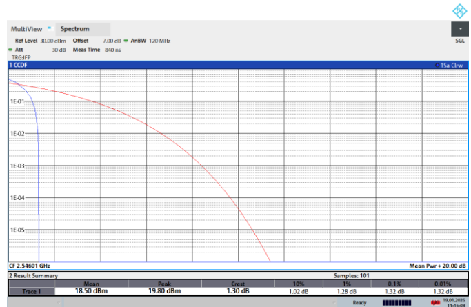
NTNV-N41-PC2-30-100-L-CP-256QPSK-Edge_1RB_Left-PASS
