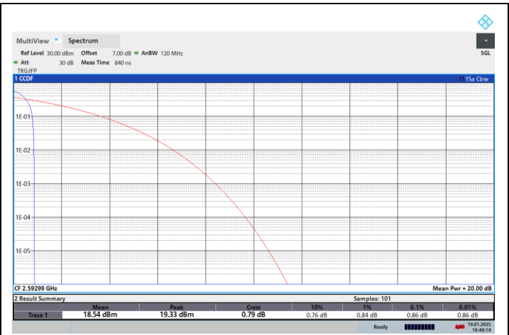
NTNV-N41-PC2-30-80-M-CP-256QPSK-Edge_1RB_Left-PASS
