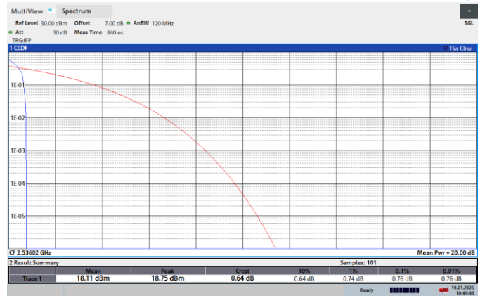
NTNV-N41-PC2-30-80-L-CP-QPSK-Edge_1RB_Left-PASS
