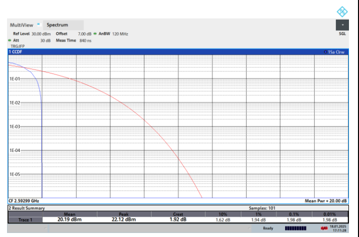
NTNV-N41-PC2-30-60-M-CP-QPSK-Edge_1RB_Left-PASS
