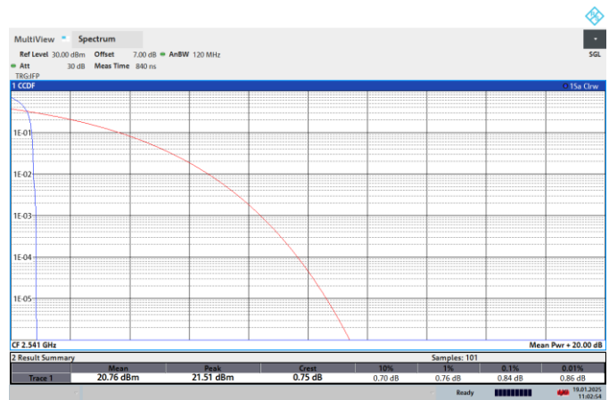
NTNV-N41-PC2-30-90-L-CP-QPSK-Edge_1RB_Left-PASS
