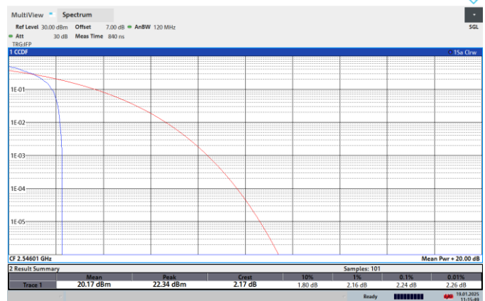
NTNV-N41-PC2-30-100-L-CP-64QPSK-Edge_1RB_Left-PASS
