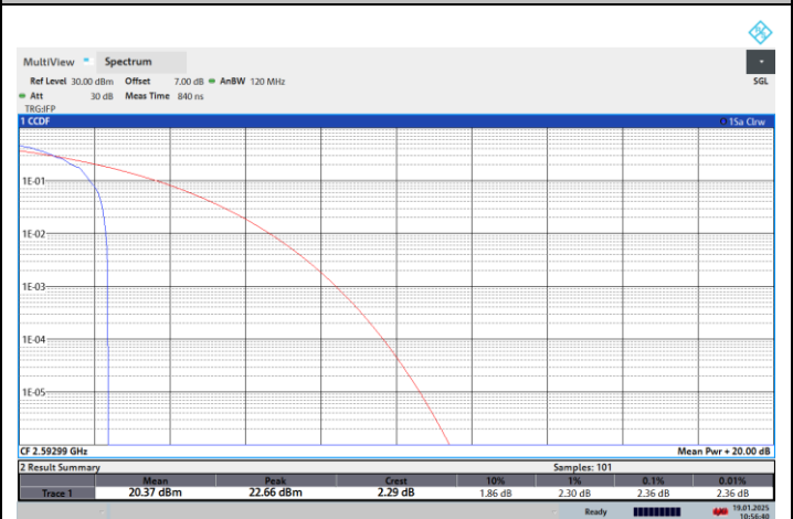
NTNV-N41-PC2-30-90-M-CP-16QPSK-Edge_1RB_Left-PASS
