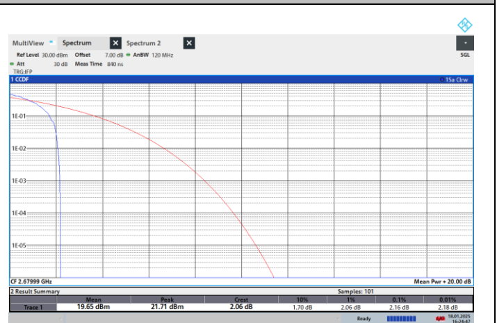
NTNV-N41-PC2-30-20-H-CP-64QPSK-Edge_1RB_Left-PASS
