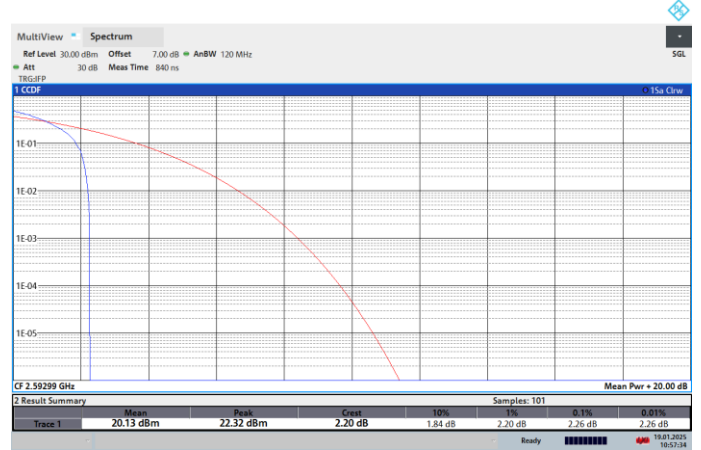
NTNV-N41-PC2-30-90-M-CP-64QPSK-Edge_1RB_Left-PASS
