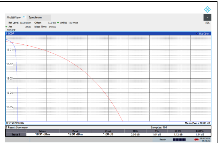
NTNV-N41-PC2-30-100-M-CP-16QPSK-Edge_1RB_Left-PASS
