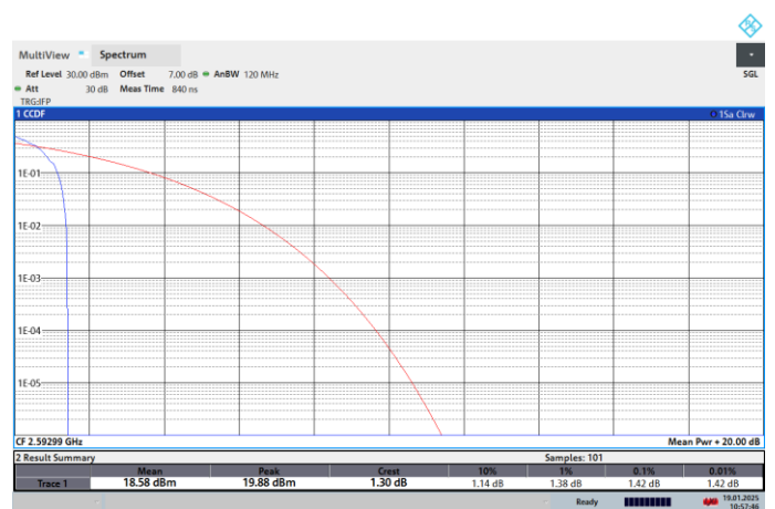
NTNV-N41-PC2-30-90-M-CP-256QPSK-Edge_1RB_Left-PASS
