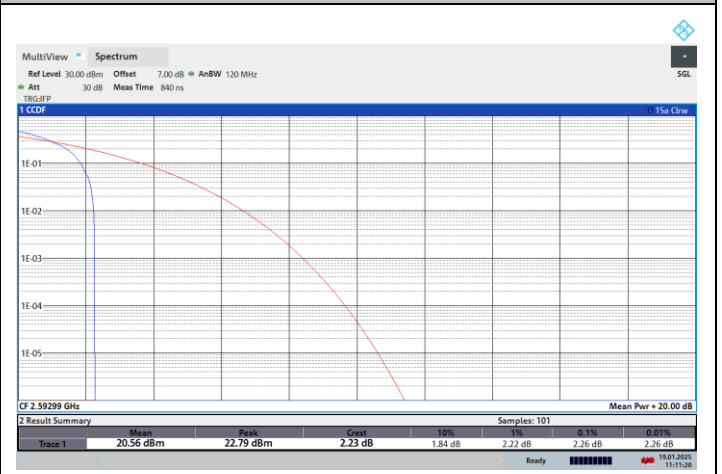
NTNV-N41-PC2-30-100-M-CP-64QPSK-Edge_1RB_Left-PASS
