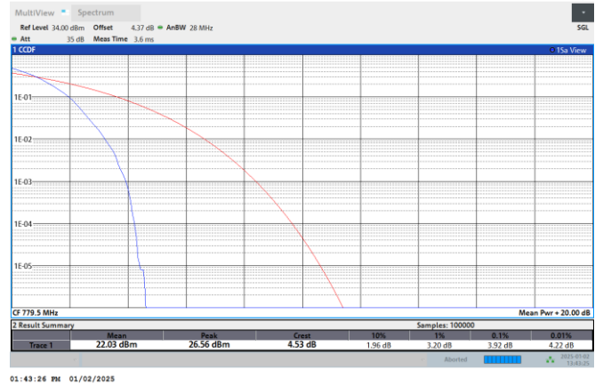
NTNV-N13-PC3-15-5-DFT-PI/2-BPSK-M- Edge_Outer_Full
