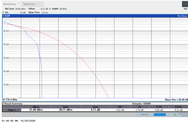
NTNV-N13-PC3-15-5-DFT-PI/2-BPSK-M- Edge_1RB_Left
