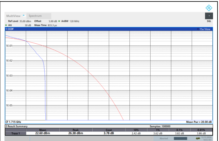
NTNV-N66-PC3-15-10-L-DFT-QPSK-Edge_1RB_Left-PASS
