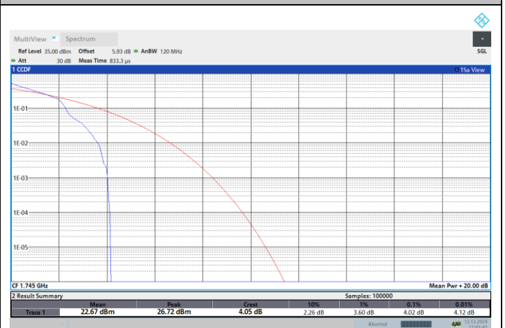
NTNV-N66-PC3-15-10-M-DFT-QPSK-Edge_1RB_Left-PASS
