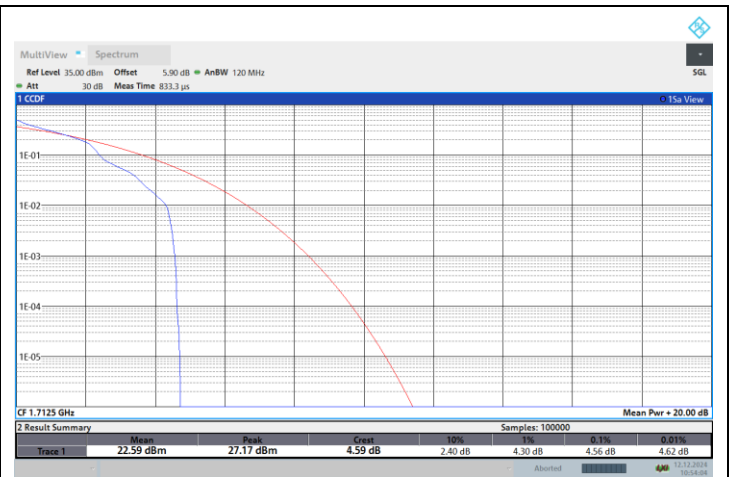
NTNV-N66-PC3-15-5-L-DFT-QPSK-Edge_1RB_Left-PASS
