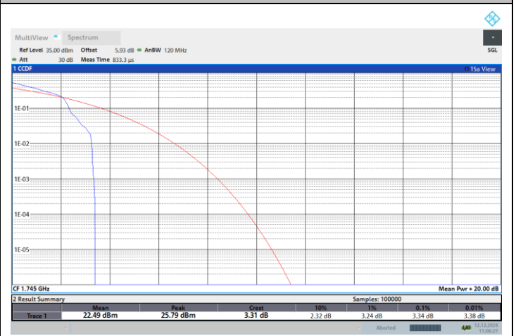
NTNV-N66-PC3-15-20-M-DFT-QPSK-Edge_1RB_Left-PASS
