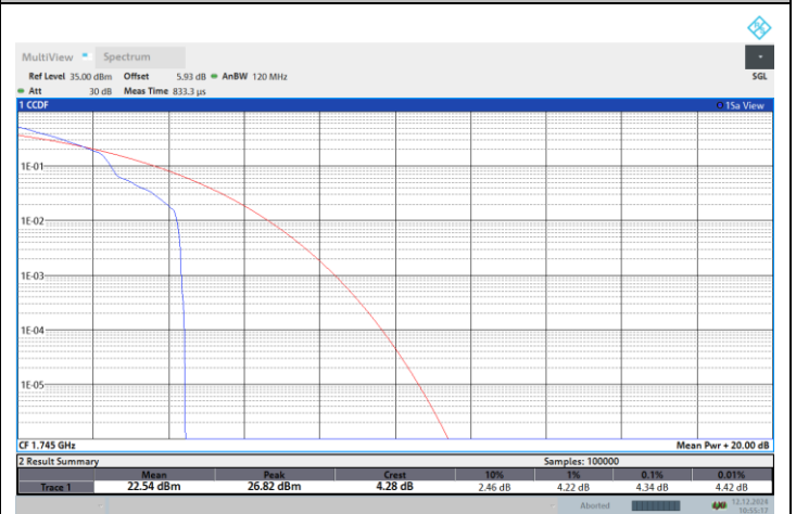
NTNV-N66-PC3-15-5-M-DFT-QPSK-Edge_1RB_Left-PASS
