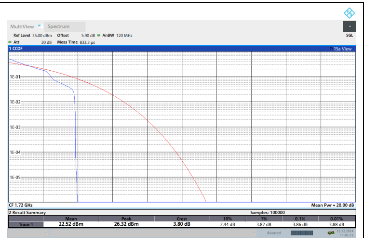
NTNV-N66-PC3-15-20-L-DFT-QPSK-Edge_1RB_Left-PASS
