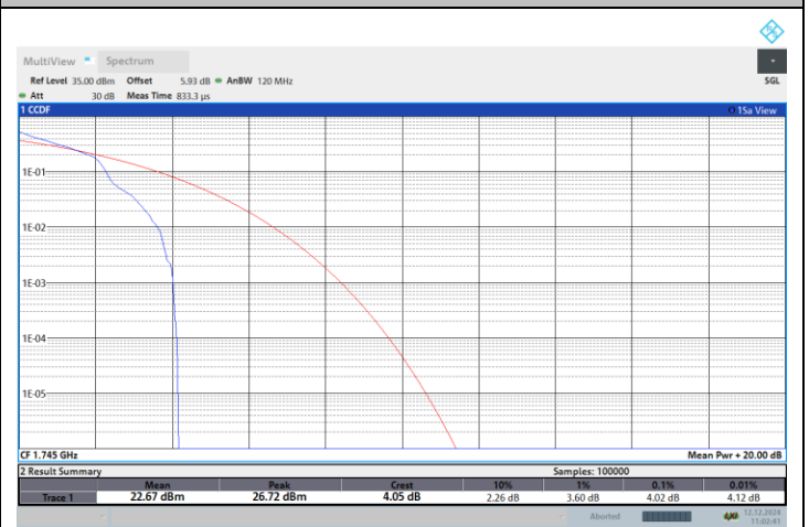
NTNV-N66-PC3-15-15-M-DFT-QPSK-Edge_1RB_Left-PASS
