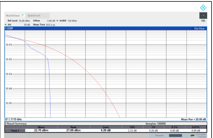
NTNV-N66-PC3-15-15-L-DFT-QPSK-Edge_1RB_Left-PASS
