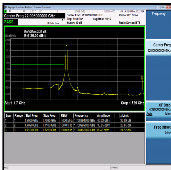
NTNV-N66-PC3-15-15-L-DFT-QPSK- Edge_1RB_Left-Ant1-PASS
