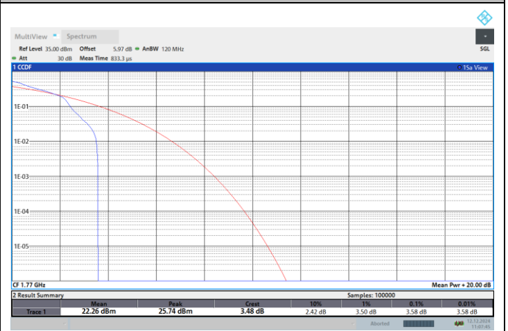
NTNV-N66-PC3-15-20-H-DFT-QPSK-Edge_1RB_Left-PASS
