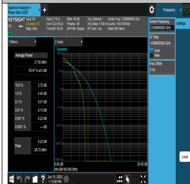
NTNV-N77-3700-3980-PC2-30-80-M-DFT-QPSK- Edge_1RB_Left-PASS
