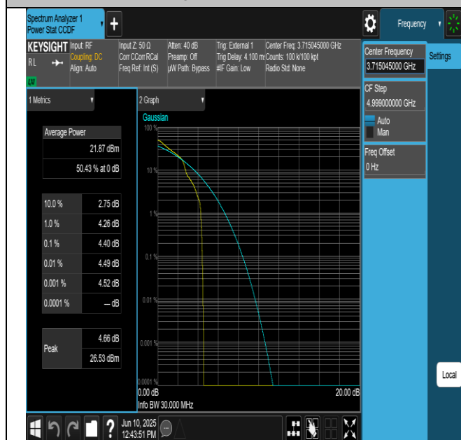
NTNV-N77-3700-3980-PC2-30-30-L-DFT-QPSK- Edge_1RB_Left-PASS
