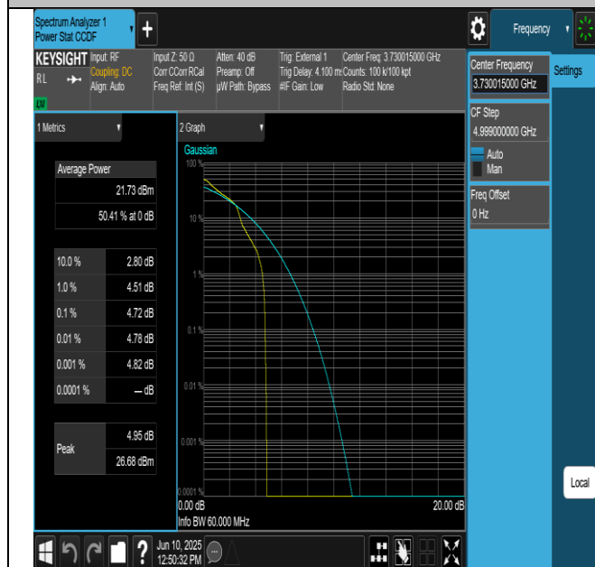
NTNV-N77-3700-3980-PC2-30-60-L-DFT-QPSK- Edge_1RB_Left-PASS
