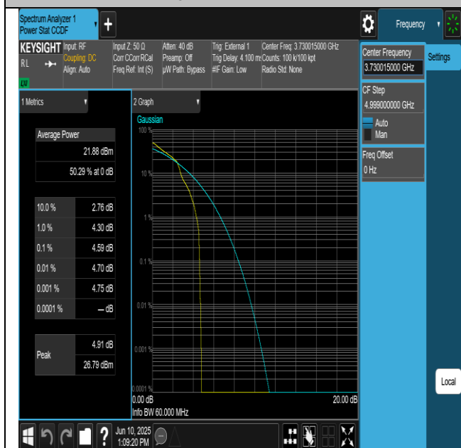
NTNV-N77-3700-3980-PC2-30-60-L-DFT-QPSK- Edge_1RB_Left-PASS
