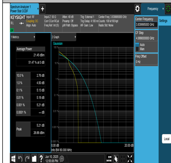
NTNV-N77-3700-3980-PC2-30-80-M-DFT-QPSK- Edge_1RB_Left-PASS
