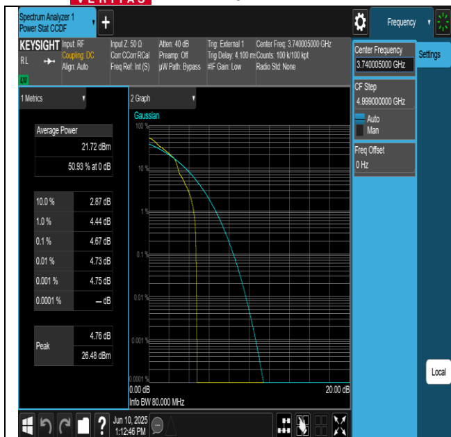
NTNV-N77-3700-3980-PC2-30-80-L-DFT-QPSK- Edge_1RB_Left-PASS
