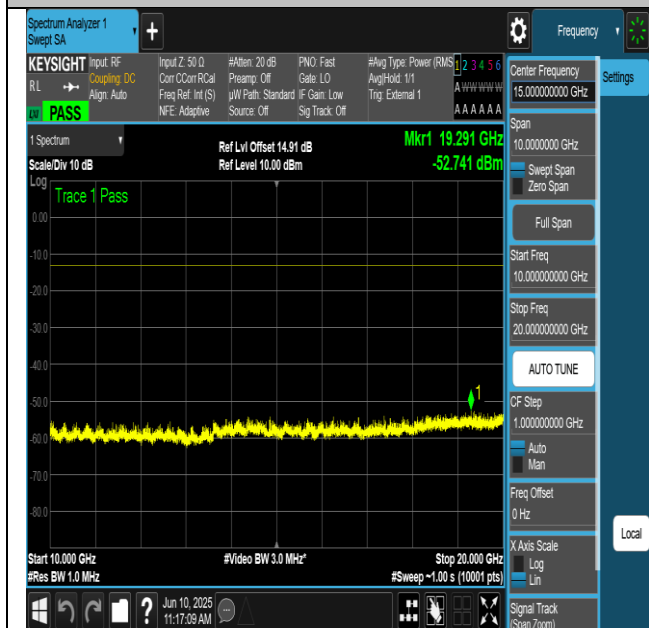
NTNV-N77-3450-3550-PC2-30-20-L-DFT-QPSK-
