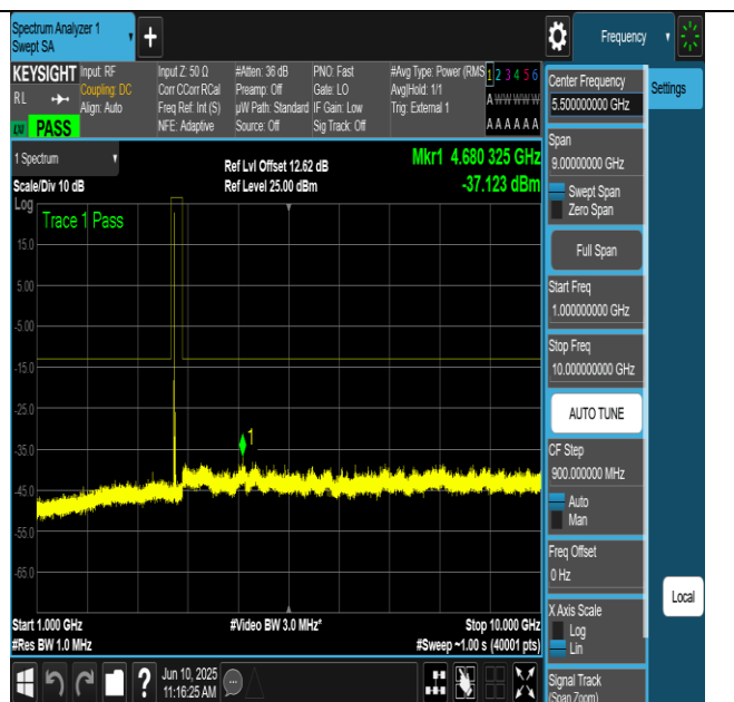
NTNV-N77-3450-3550-PC2-30-20-L-DFT-QPSK-
