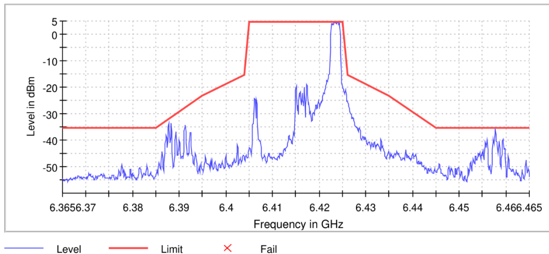
11AX20MIMO_Ant8_6415_RU26/8
