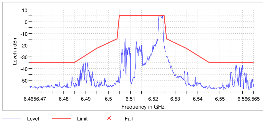
11AX20MIMO_Ant8_6515_RU26/8
