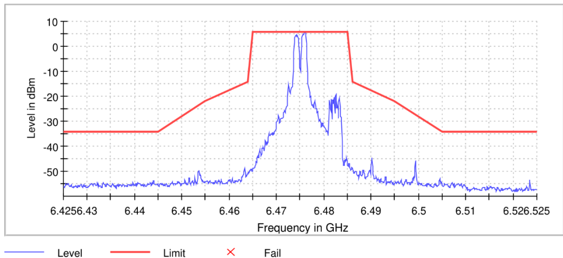
11AX20MIMO_Ant8_6475_RU26/4
