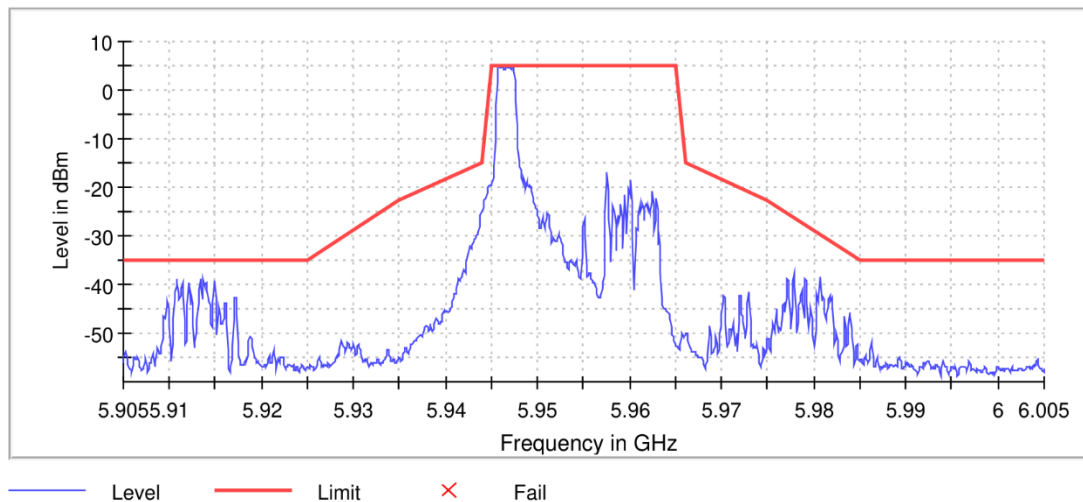
11AX20MIMO_Ant8_5955_RU26/0
