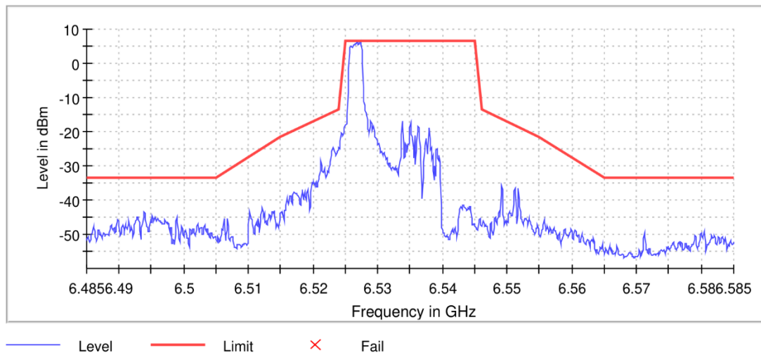
11AX20MIMO_Ant8_6535_RU26/0
