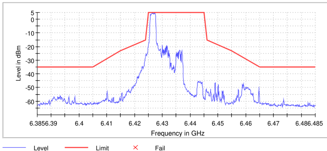
11AX20MIMO_Ant8_6435_RU26/0
