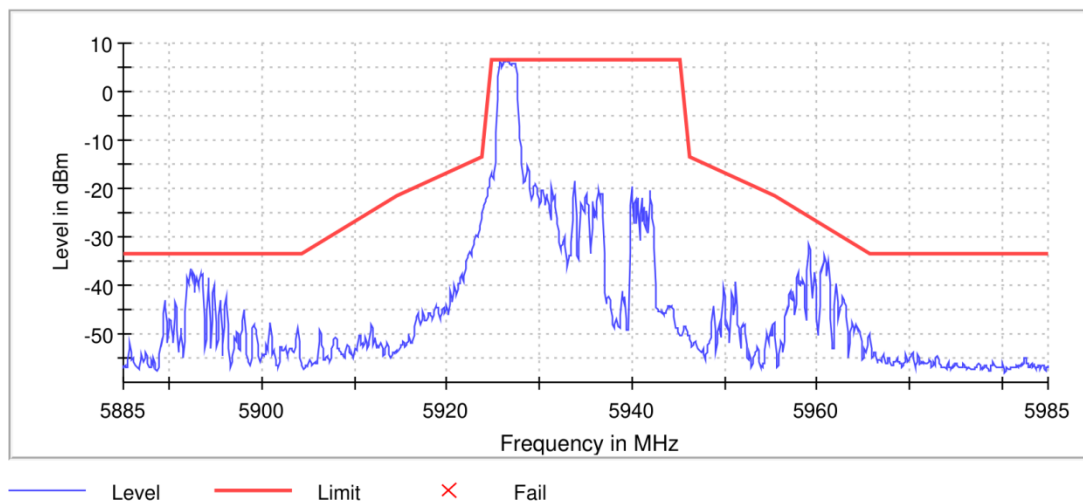
11AX20MIMO_Ant8_5935_RU26/0
