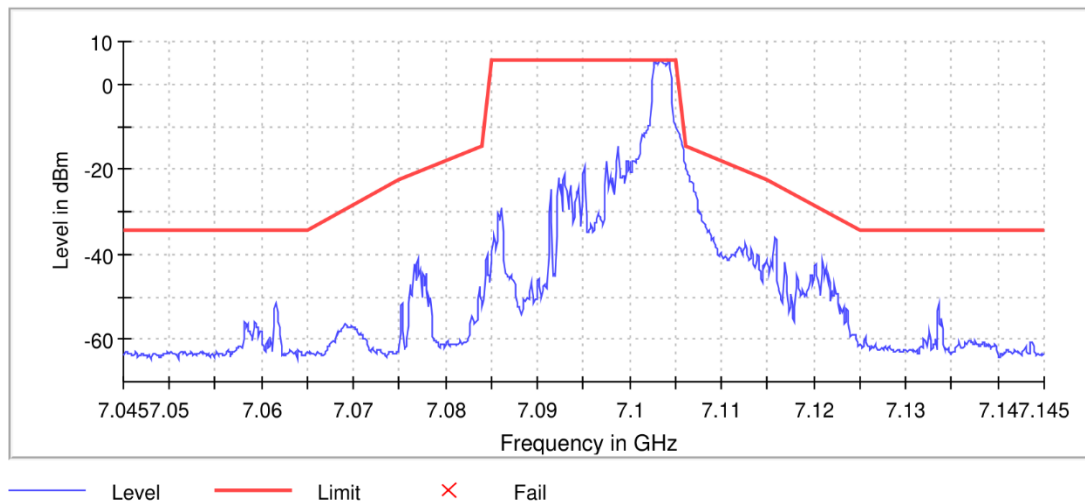
11AX20MIMO_Ant8_7095_RU26/8
