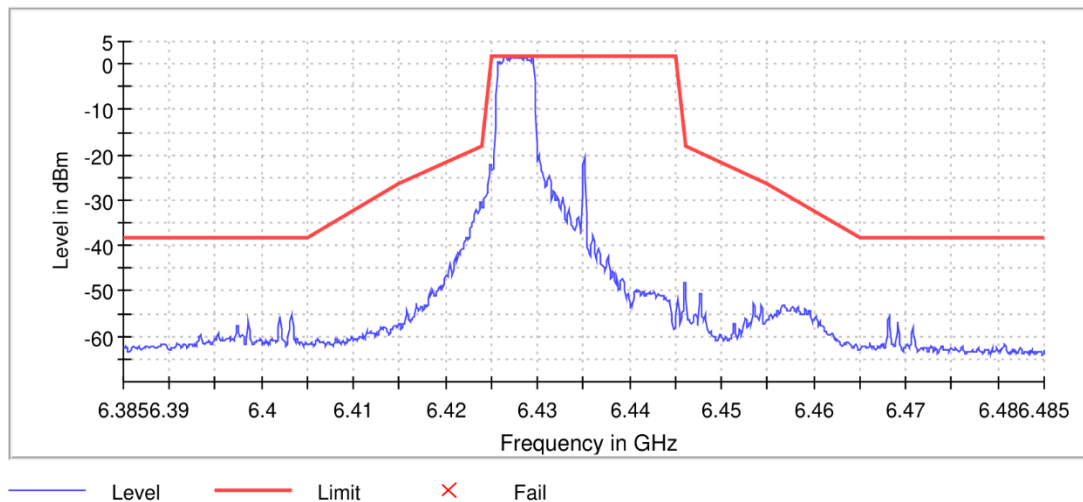
11AX20MIMO_Ant8_6435_RU52/37
