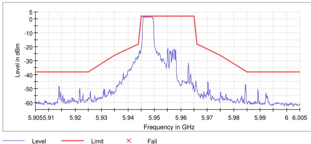
11AX20MIMO_Ant8_5955_RU52/37
