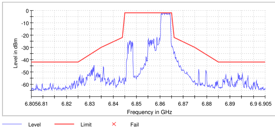
11AX20MIMO_Ant8_6855_RU52/40
