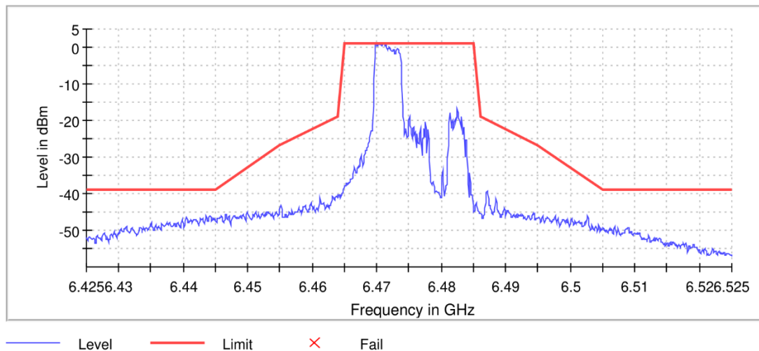
11AX20MIMO_Ant8_6475_RU52/38
