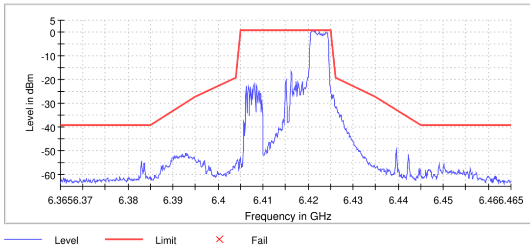
11AX20MIMO_Ant8_6415_RU52/40
