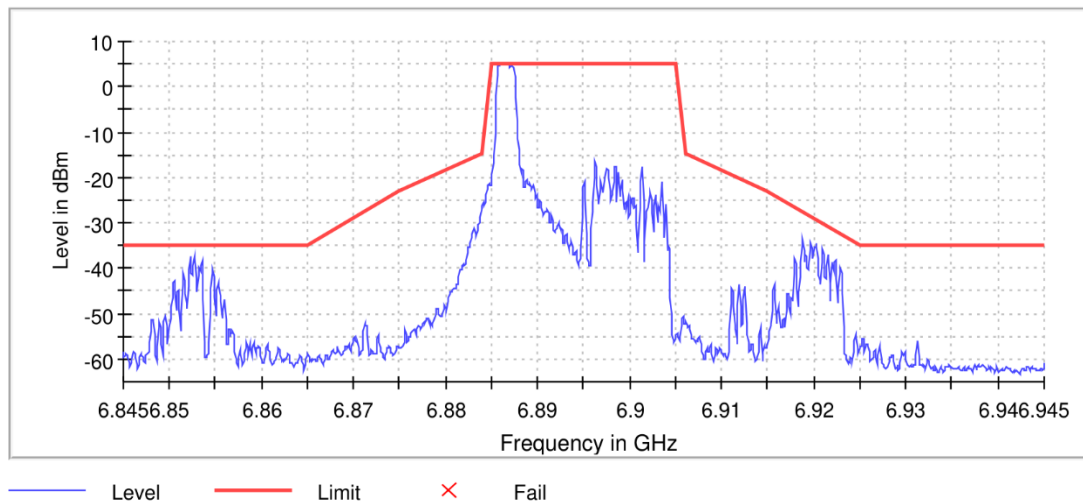
11AX20MIMO_Ant8_6895_RU26/0
