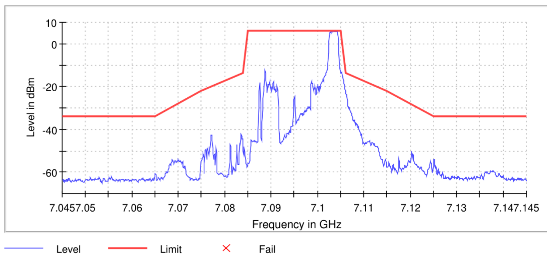
11AX20MIMO_Ant6_7115_RU26/8
