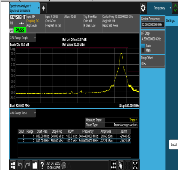
26(824-849)-10MHz-256QAM-26840-1RB#0-PASS
