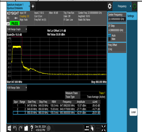
26(824-849)-3MHz-QPSK-26805-15RB#0-PASS
