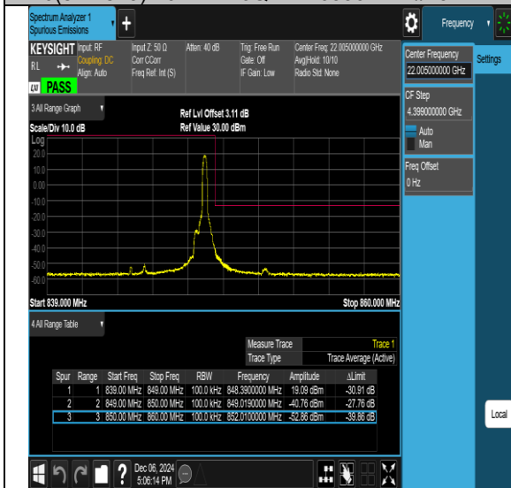
26(824-849)-15MHz-QPSK-26865-1RB#0-PASS
