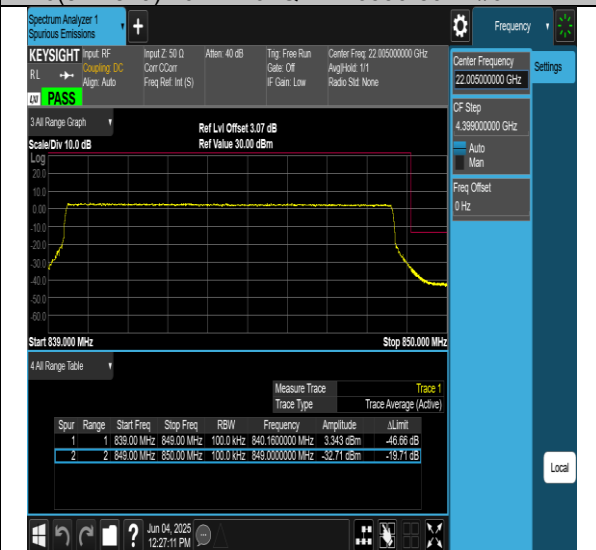
26(824-849)-10MHz-256QAM-26840-50RB#0-PASS
