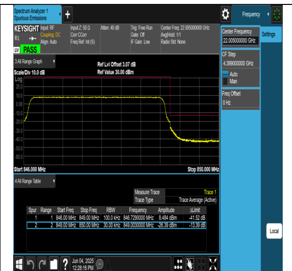
26(824-849)-3MHz-256QAM-26805-15RB#0-PASS
