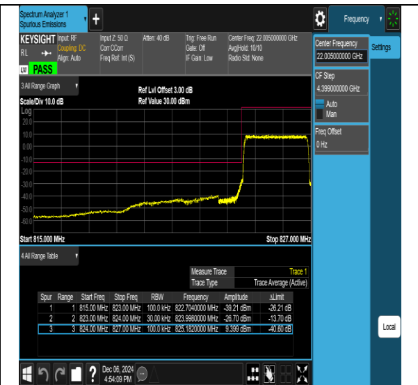
26(824-849)-3MHz-QPSK-27025-15RB#0-PASS
