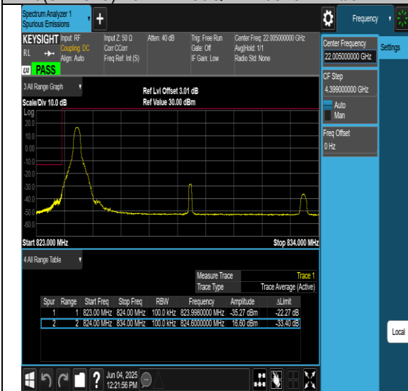
26(824-849)-10MHz-256QAM-26990-1RB#49-PASS
