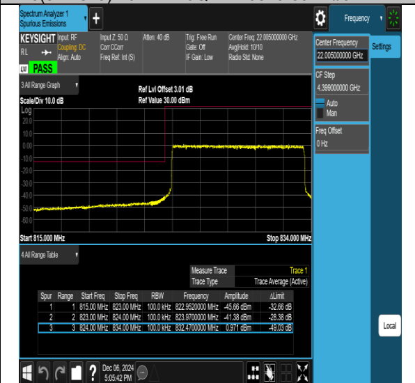
26(824-849)-10MHz-16QAM-26990-50RB#0-PASS
