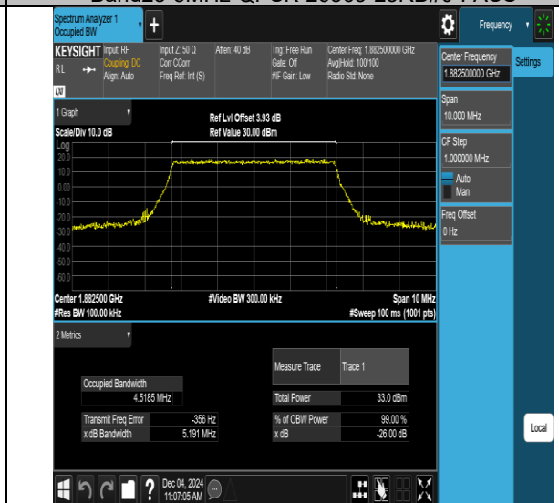
Band25-5MHz-QPSK-26365-25RB#0-PASS
