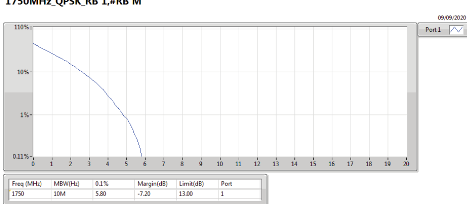
Band 4_LTE_10MHz_Nss1,QPSK_1TX 1750MHz_QPSK_RB 1,#RB M
