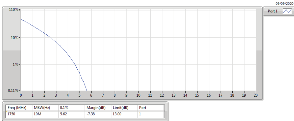
Band 4_LTE_10MHz_Nss1,QPSK_1TX 1750MHz_QPSK_RB 50,#RB 0
