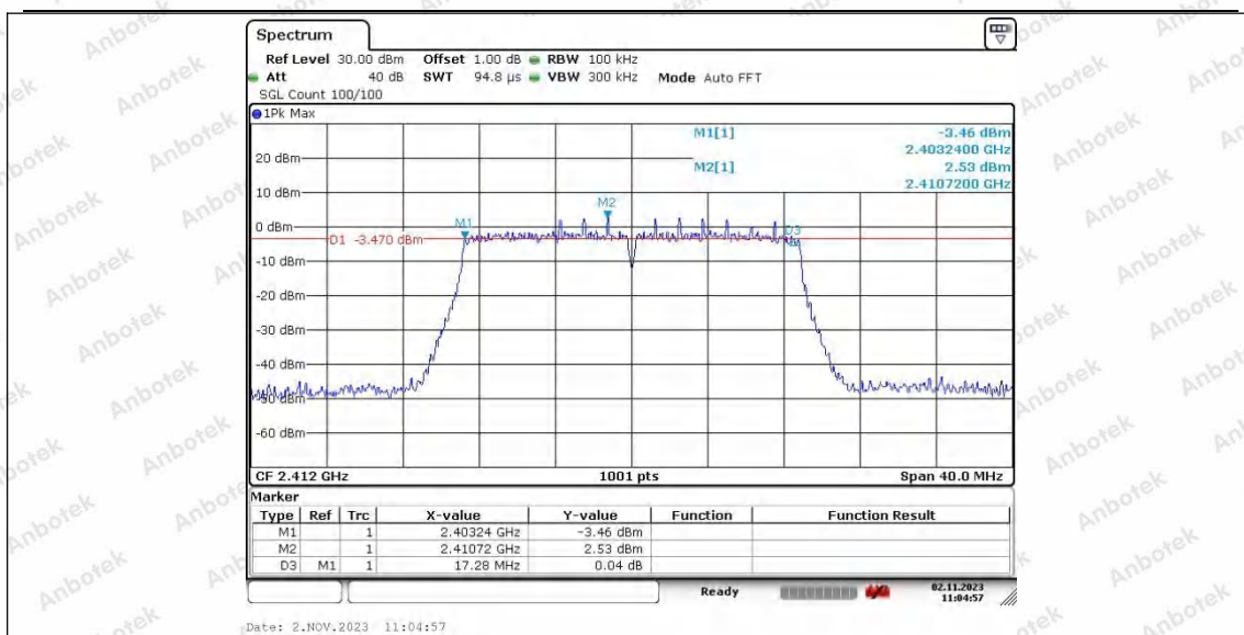
11N20SISO_Ant2_2412
