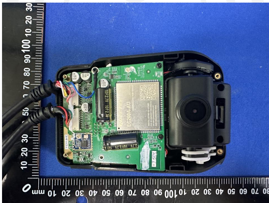
WWAN ANT
