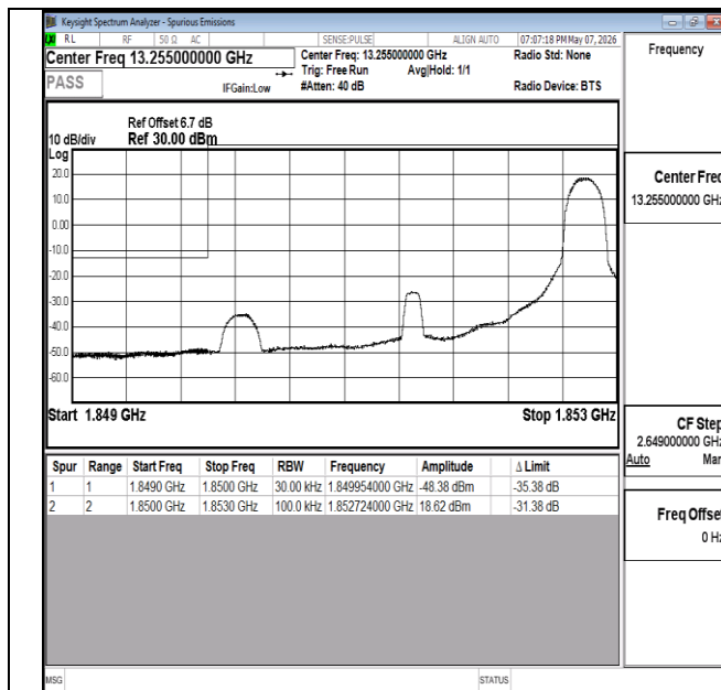
Band2-3MHz-16QAM-18615-1RB#14-PASS
