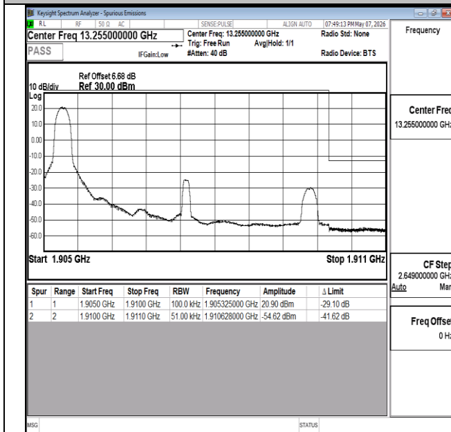
Band2-5MHz-QPSK-19175-1RB#0-PASS
