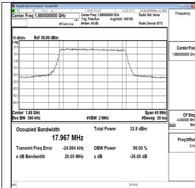
Band2-20MHz-QPSK-18900-100RB#0-PASS
