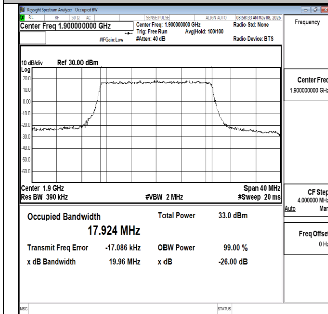
Band2-20MHz-QPSK-19100-100RB#0-PASS
