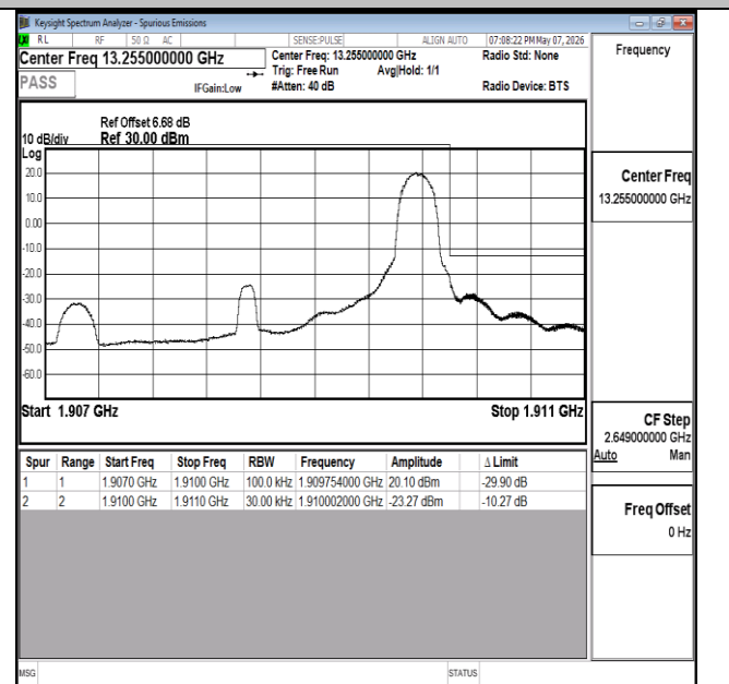
Band2-3MHz-QPSK-19185-1RB#14-PASS
