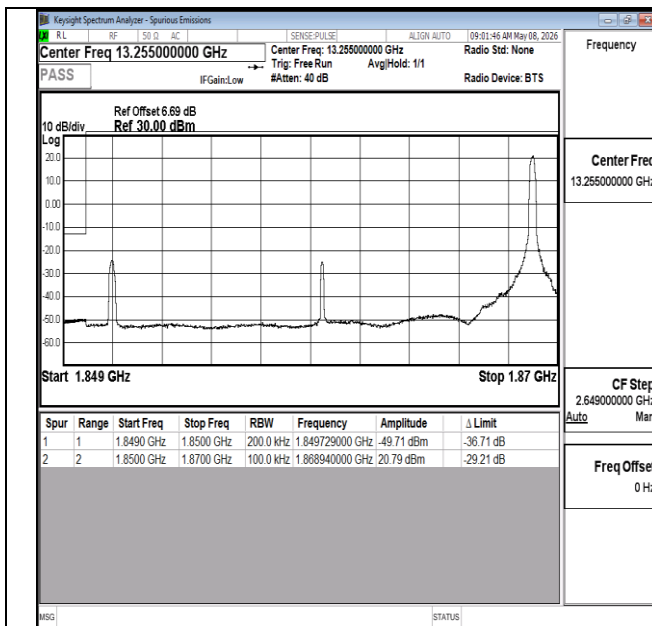
Band2-20MHz-QPSK-18700-1RB#99-PASS
