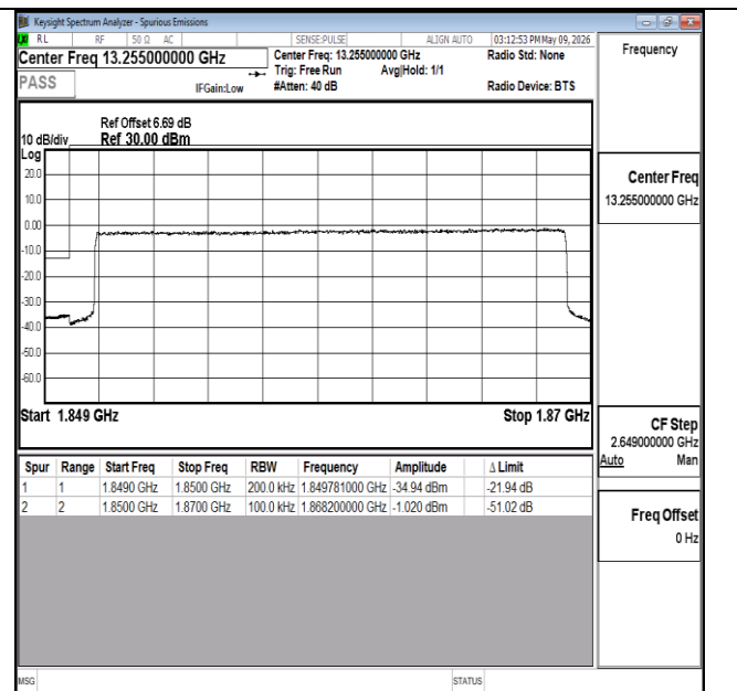
Band2-20MHz-QPSK-18700-100RB#0-PASS
