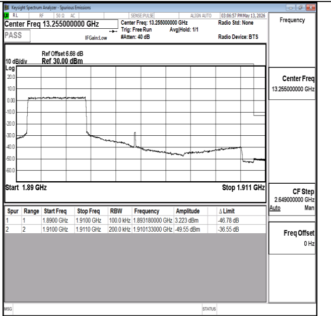
Band2-20MHz-16QAM-19100-27RB#0-PASS
