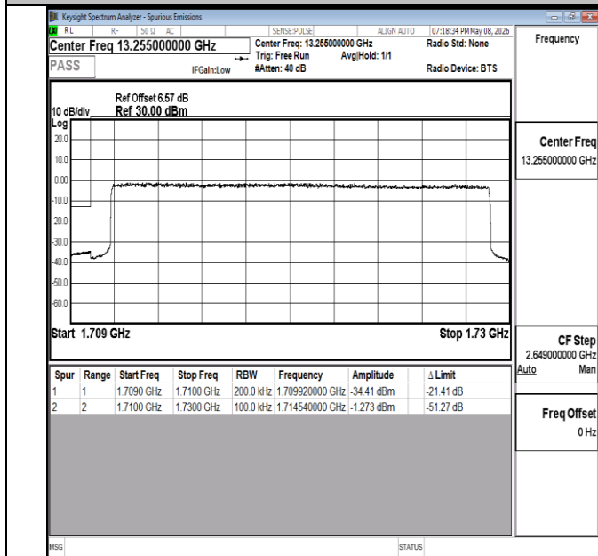
Band4-20MHz-QPSK-20050-100RB#0-PASS
