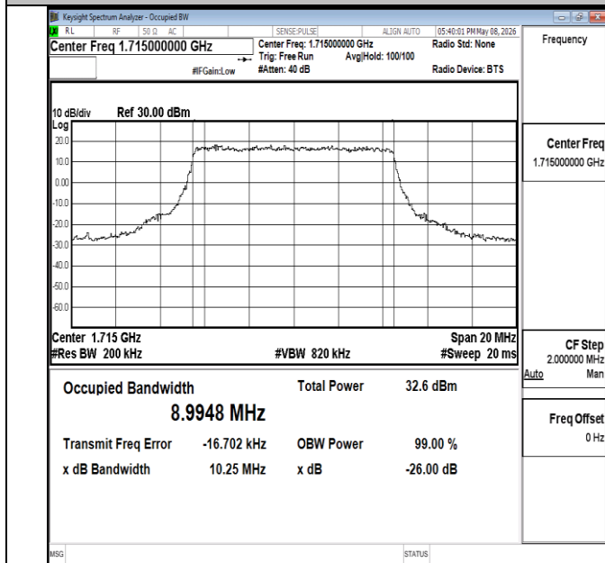
Band4-10MHz-QPSK-20000-50RB#0-PASS
