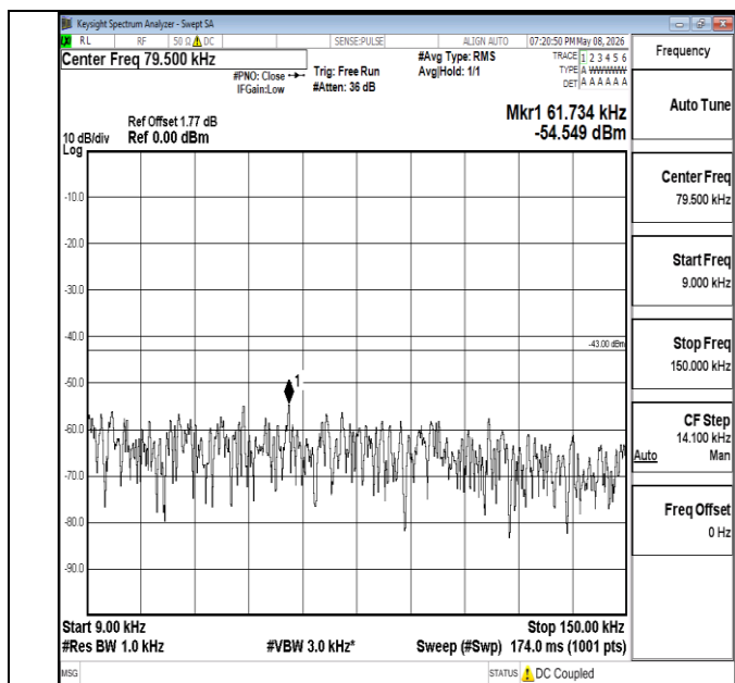
Band4-20MHz-QPSK-20175-1RB#0-0.009~0.15-PASS
