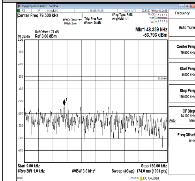
Band5-3MHz-QPSK-20635-1RB#0-0.009~0.15-PASS
