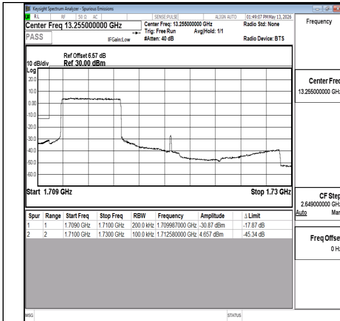
Band66-20MHz-QPSK-132072-27RB#0-PASS
