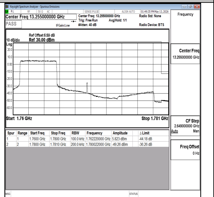
Band66-20MHz-QPSK-132572-27RB#0-PASS
