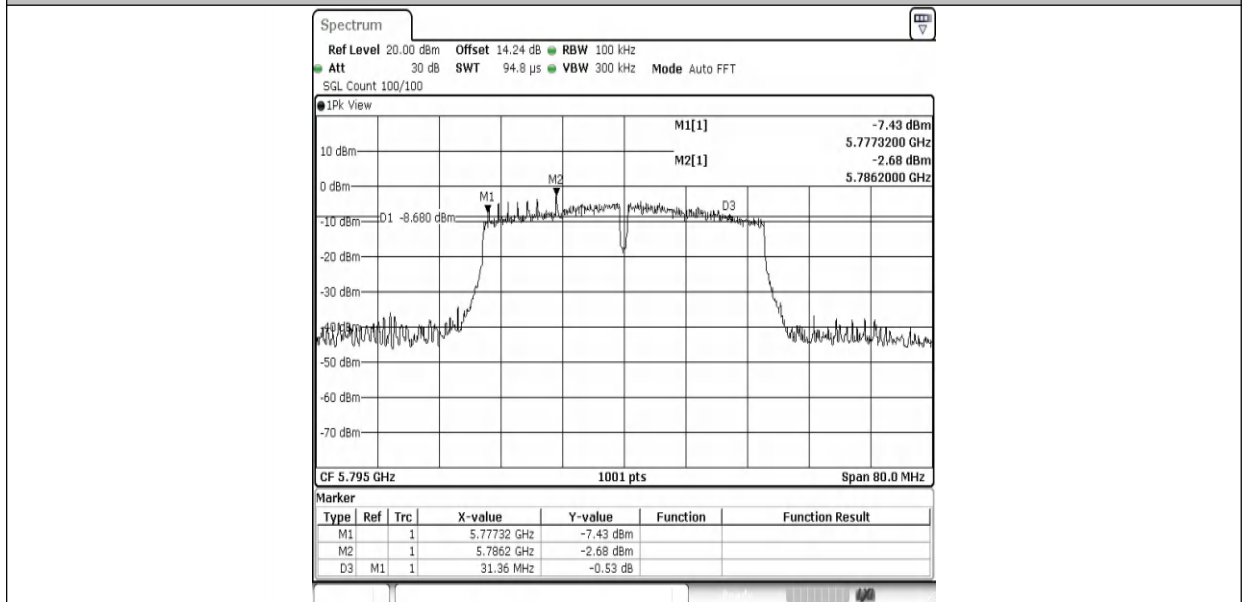
11N40ISO-Ant1-5795-PASS
