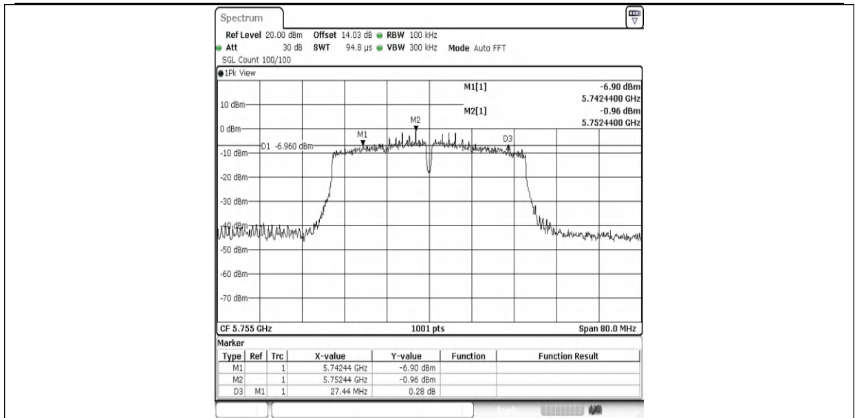
11N40ISO-Ant1-5755-PASS
