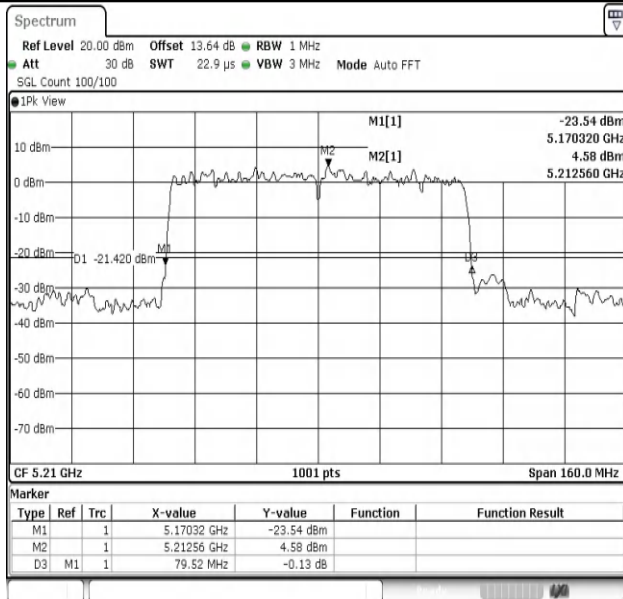
11AC80SISO-Ant1-5210
