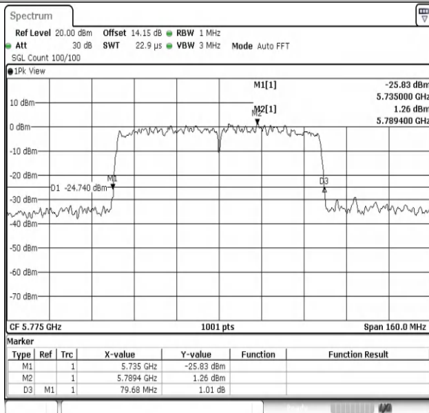
11AC80SISO-Ant1-5775
