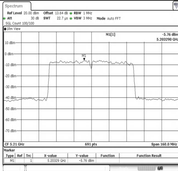
11AC80SISO-Ant1-5210-PASS
