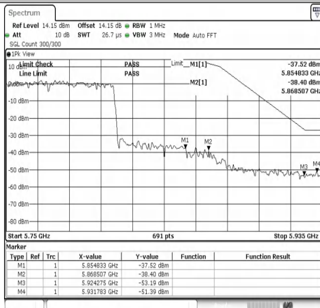
11AC80SISO-Ant1-5775-PASS
