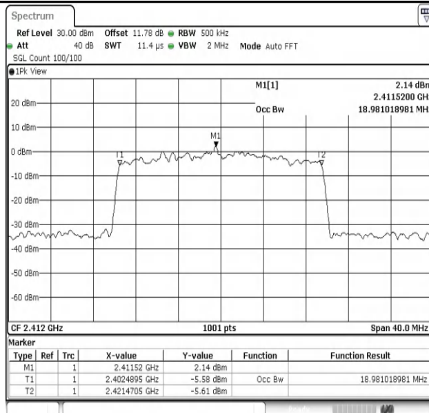
11AX20MIMO-Ant1-2412
