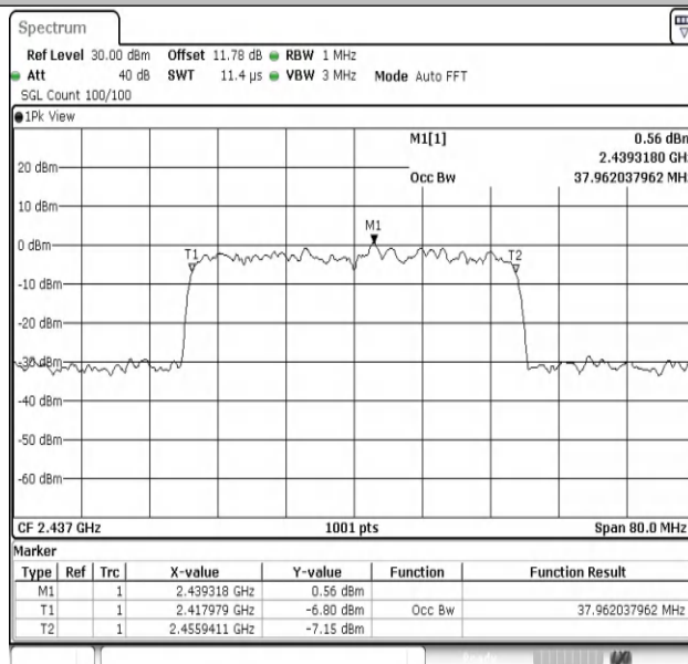
11AX40MIMO-Ant2-2437
