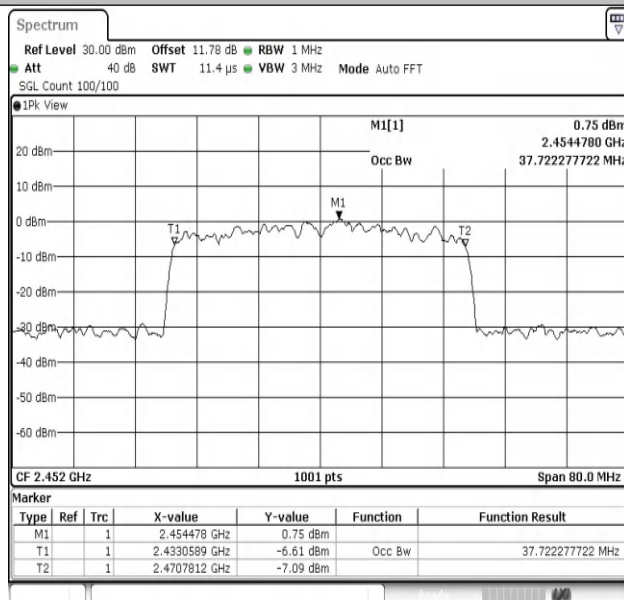
11AX40MIMO-Ant2-2452
