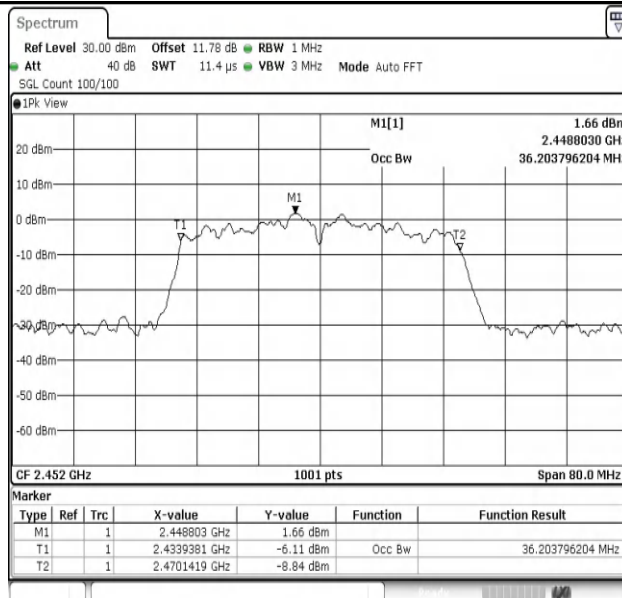
11N40MIMO-Ant1-2452
