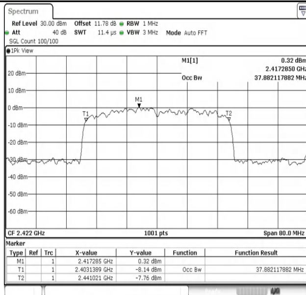
11AX40MIMO-Ant1-2422
