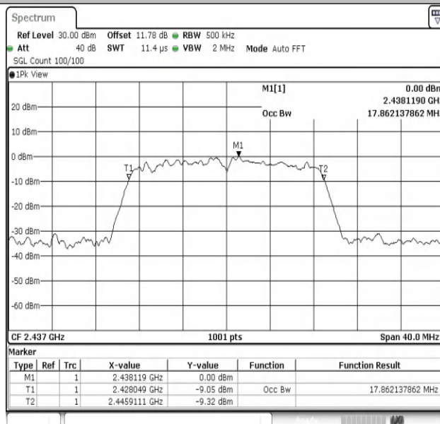
11N20MIMO-Ant2-2437
