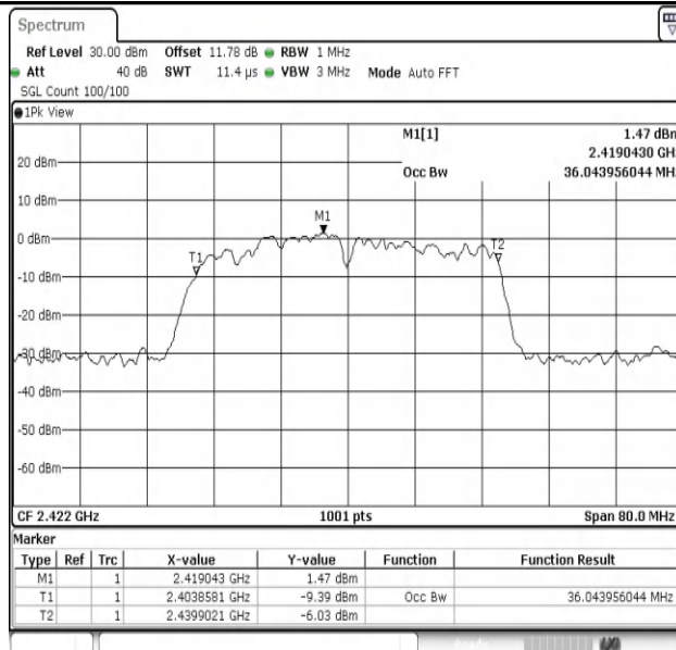
11N40MIMO-Ant1-2422
