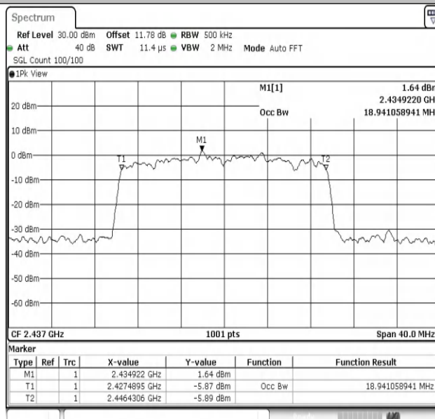
11AX20MIMO-Ant2-2437
