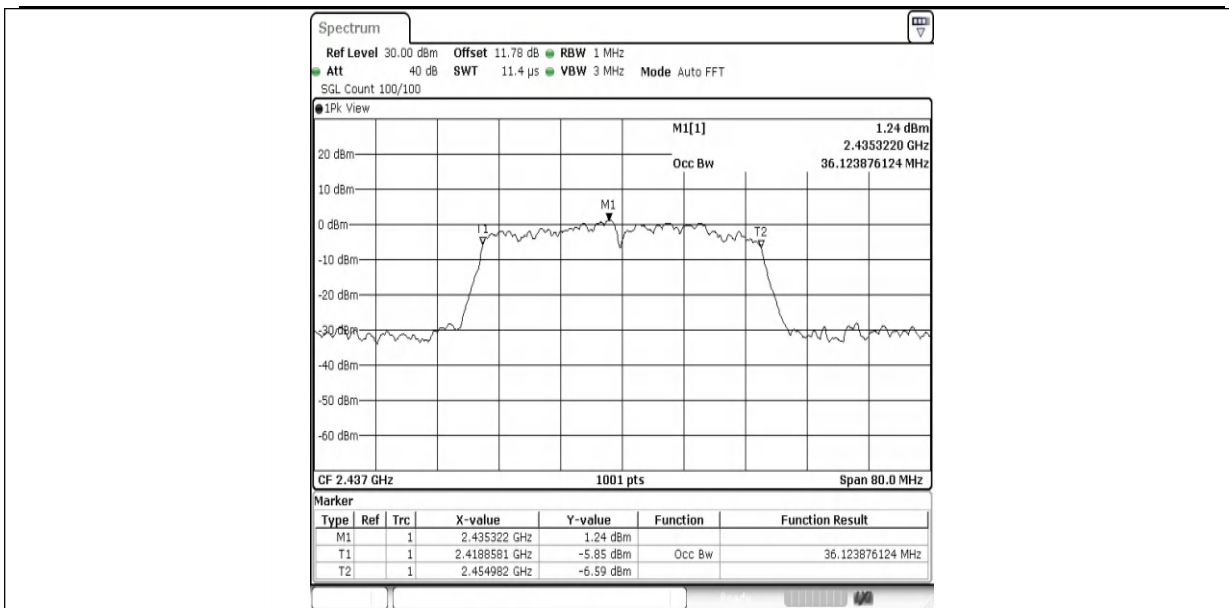
11N40MIMO-Ant1-2437
