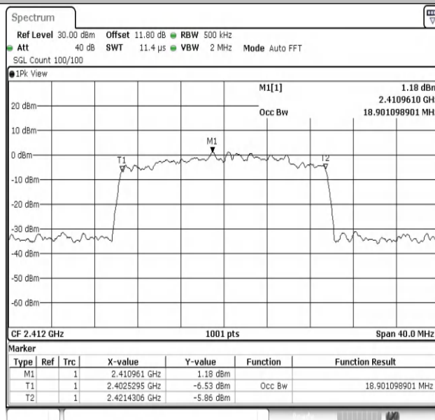
11AX20MIMO-Ant2-2412
