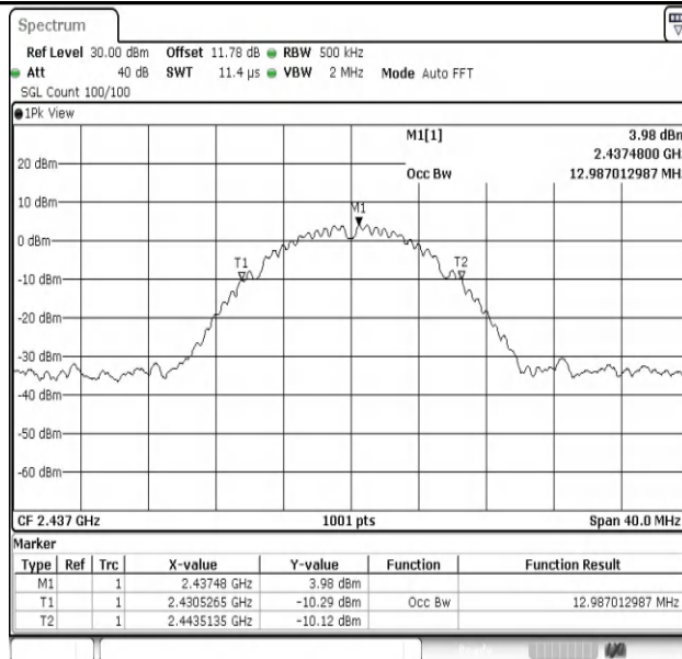
11B-Ant1-2437
