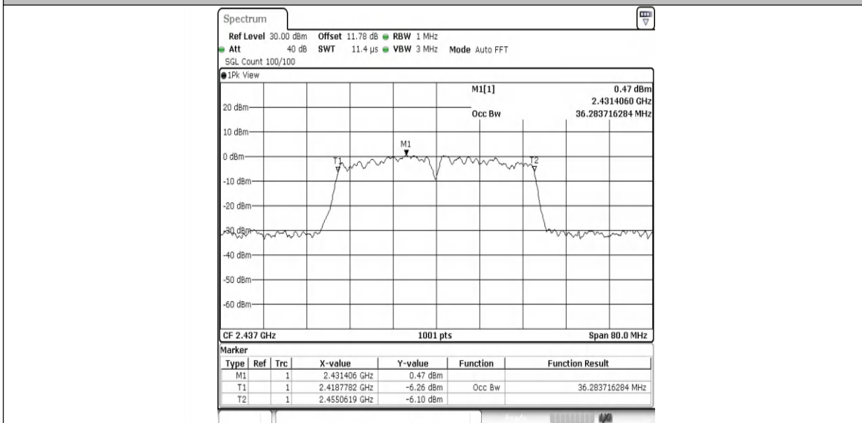
11N40MIMO-Ant2-2437
