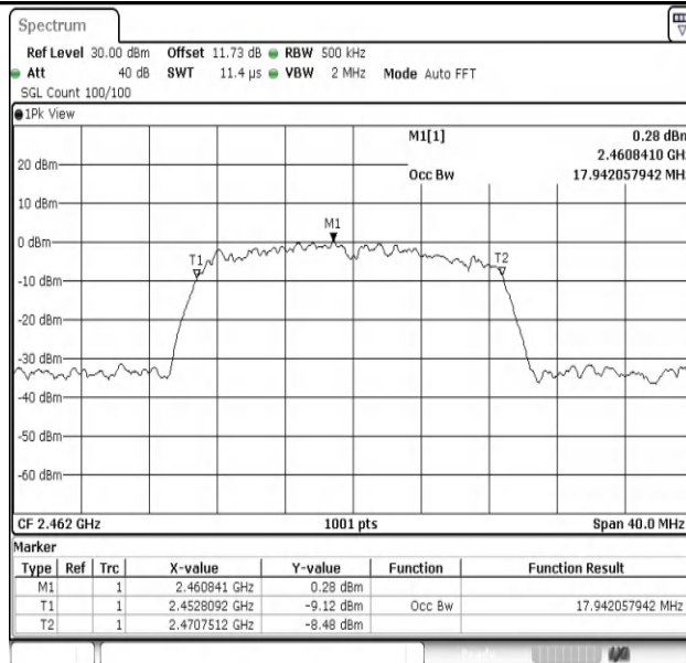
11N20MIMO-Ant1-2462
