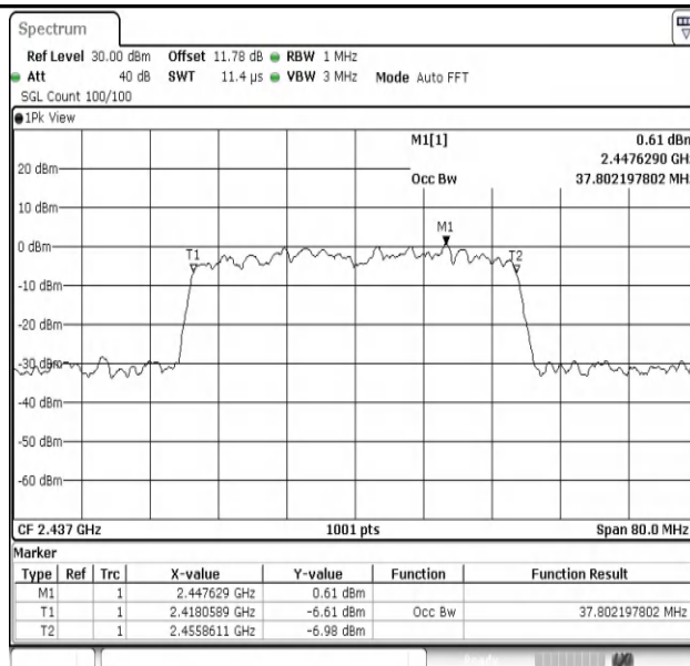
11AX40MIMO-Ant1-2437
