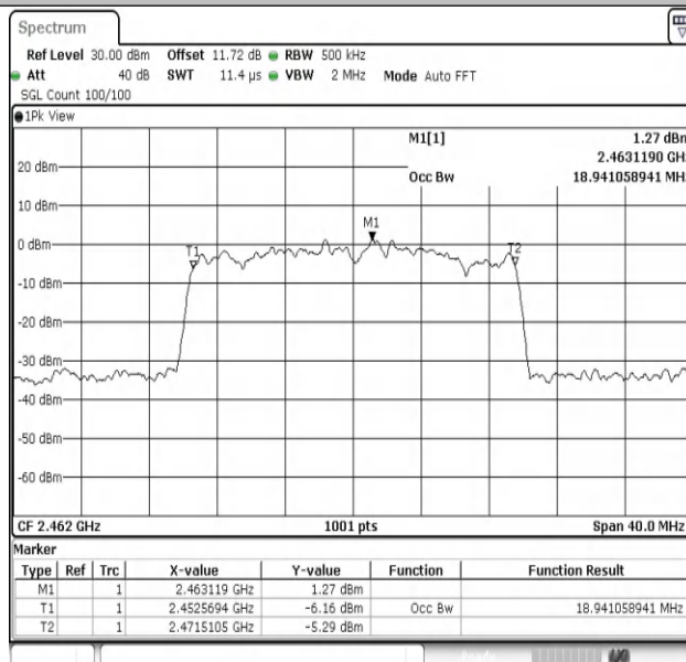
11AX20MIMO-Ant2-2462
