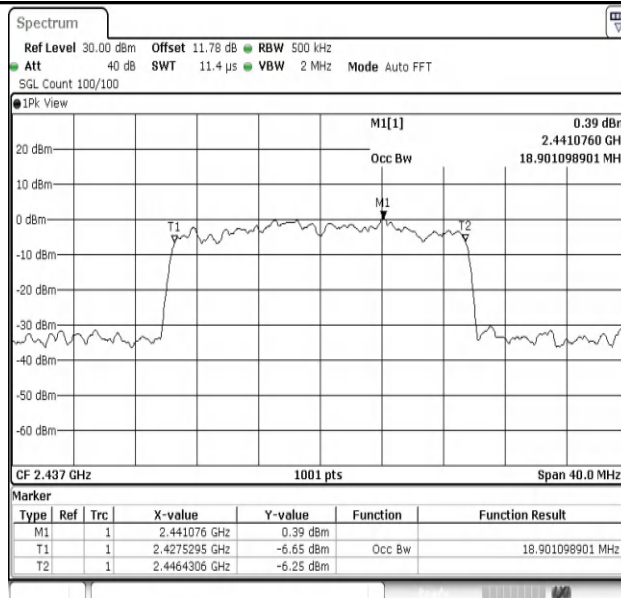
11AX20MIMO-Ant1-2437
