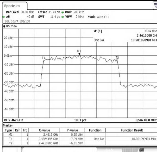
11AX20MIMO-Ant1-2462
