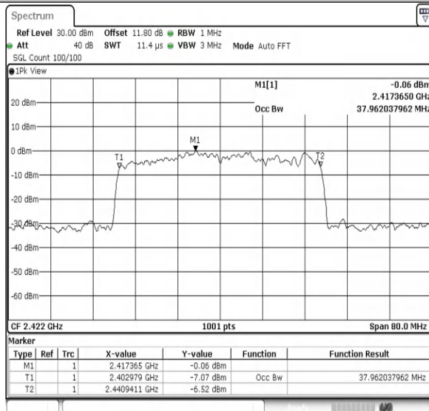
11AX40MIMO-Ant2-2422
