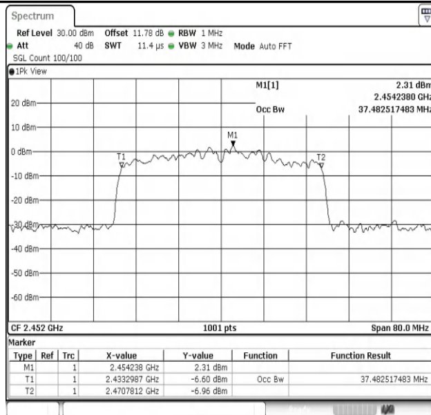
11AX40MIMO-Ant1-2452
