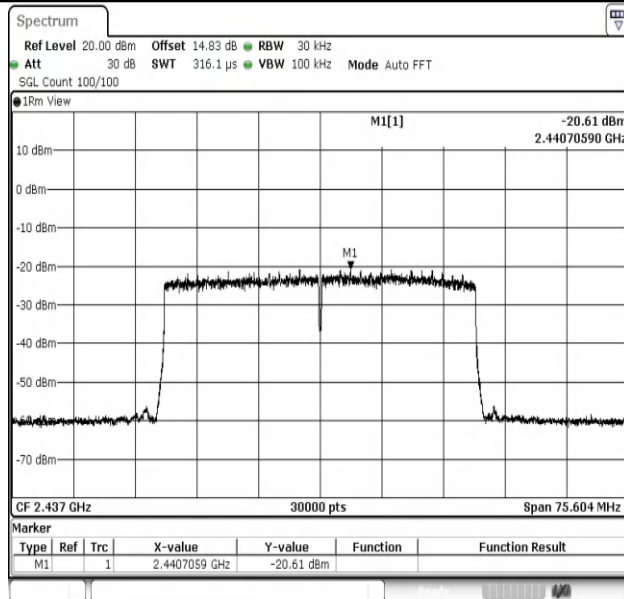
11AX40MIMO-Ant1-2437-PASS
