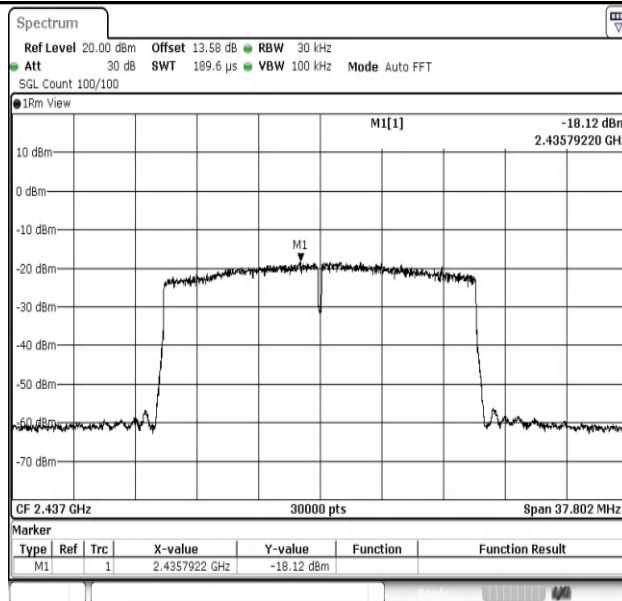
11AX20MIMO-Ant1-2437-PASS
