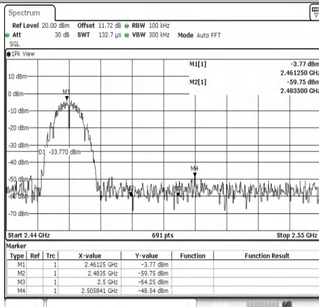
11B-Ant2-2462-PASS
