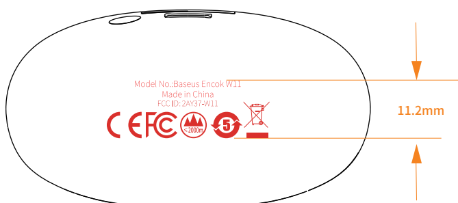
底视图
