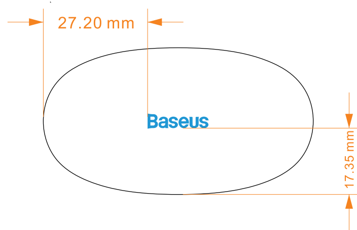
顶视图
