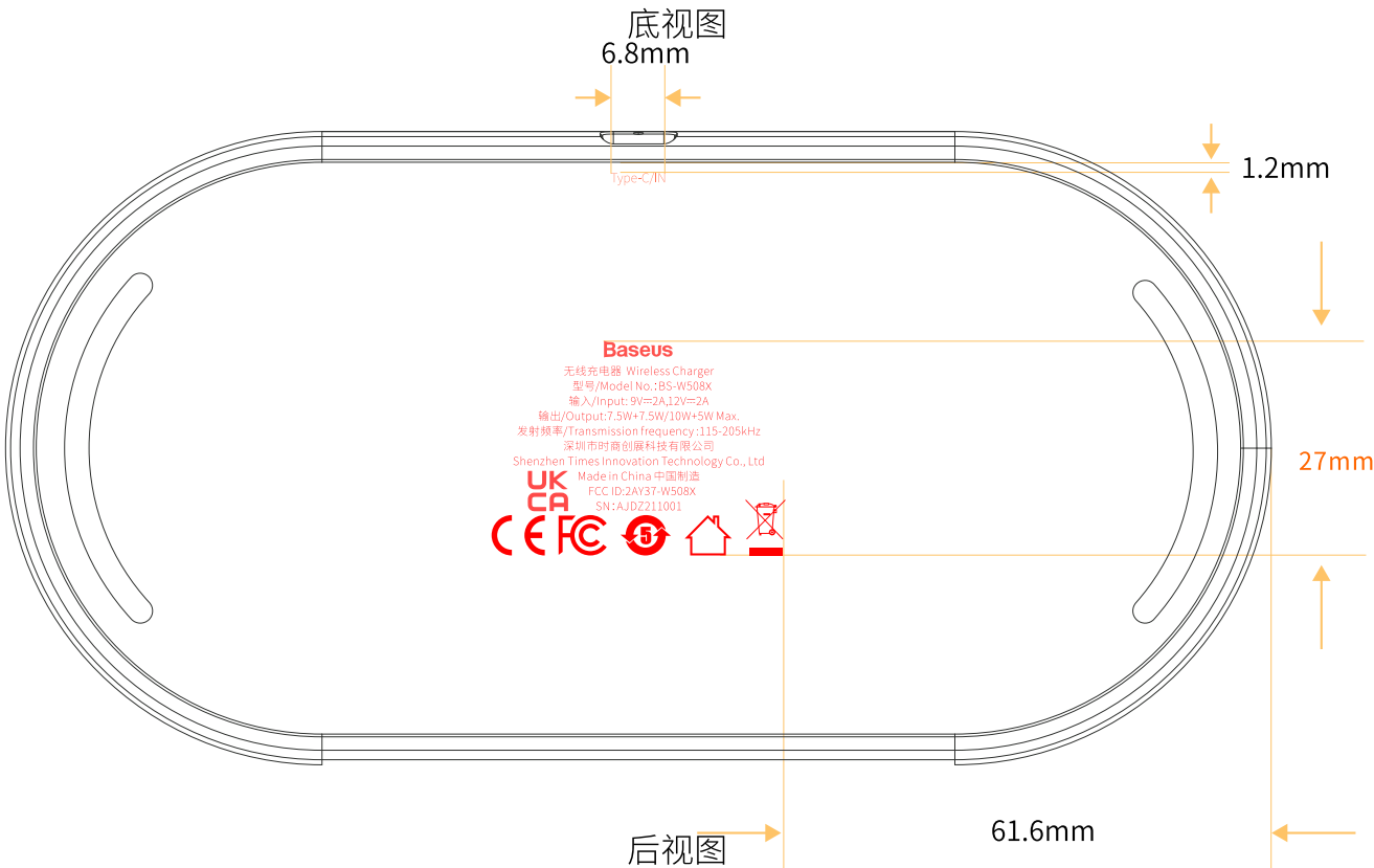
后视图
