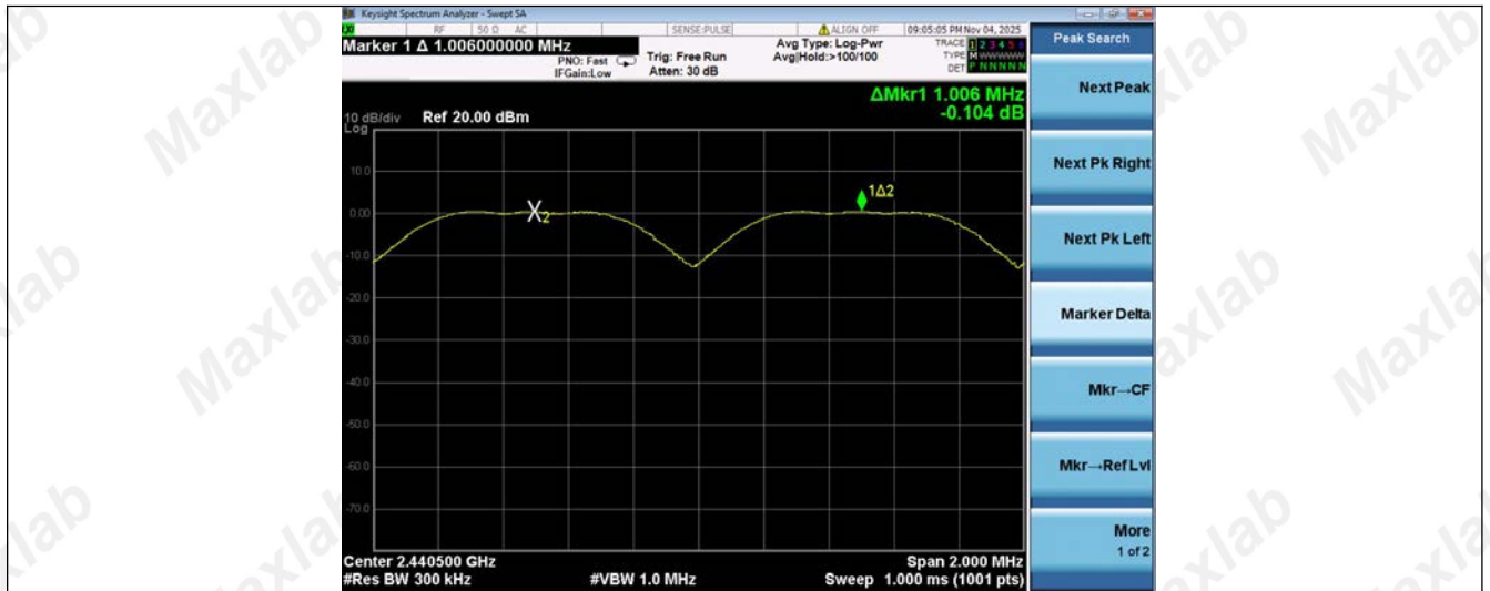
GFSK
