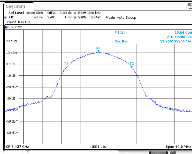
11B_Ant1_2437
