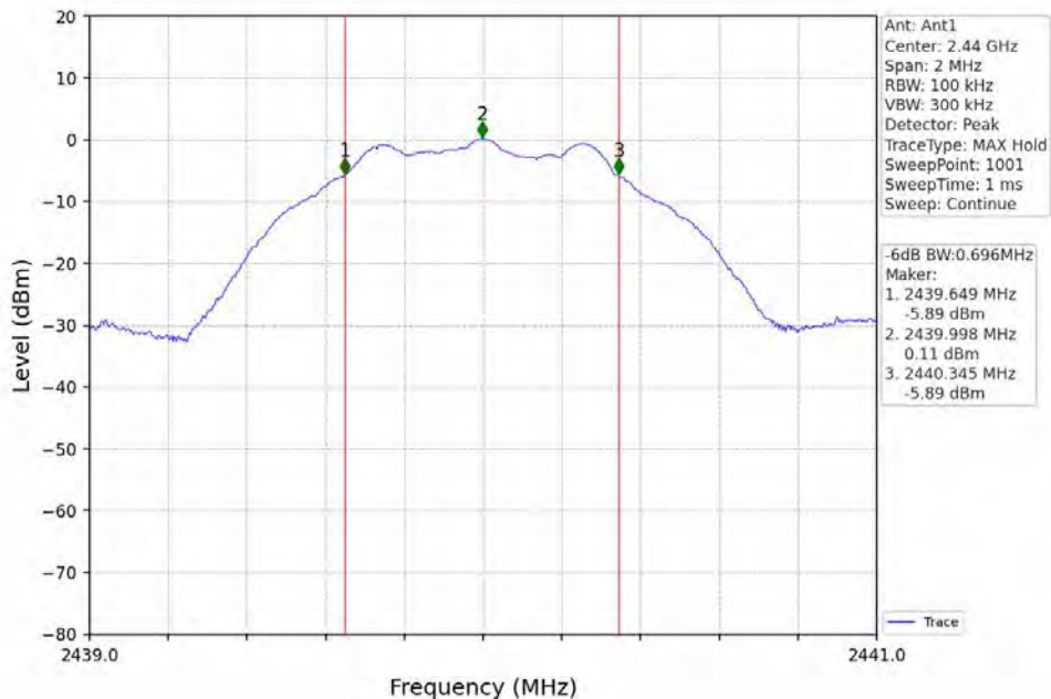
1M_MCH_2440MHz_DataRate=_Ant1_NTNV
