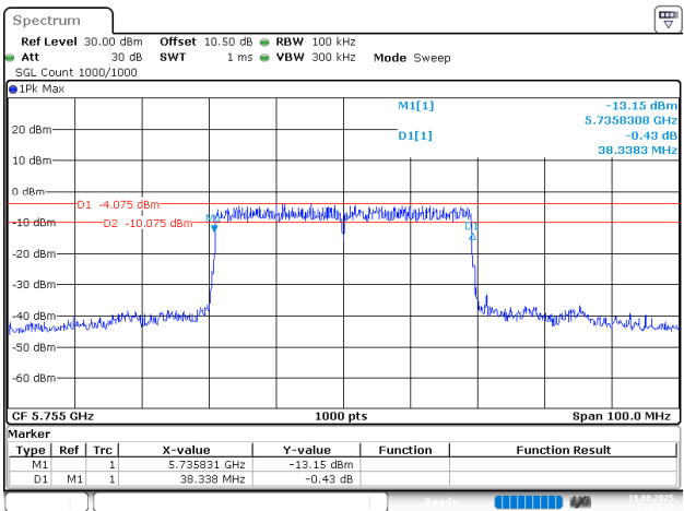
802.11ax40_5755MHz_Chain 0
