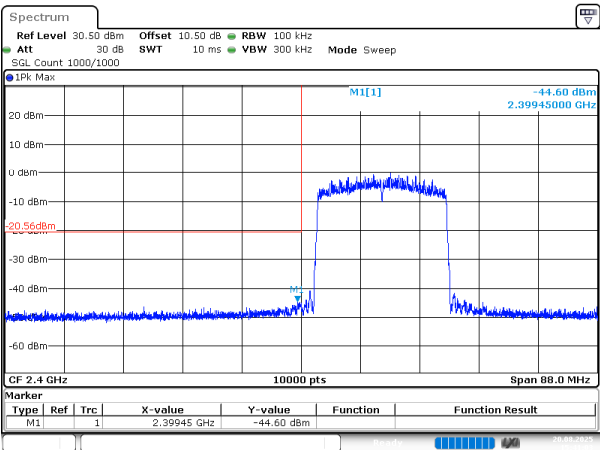
802.11ax20_2412MHz_Chain 1
