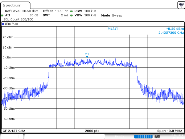
802.11ax20_2437MHz_Chain 1
