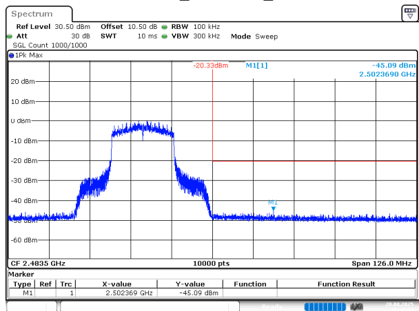
802.11ax20_2462MHz_Chain 1
