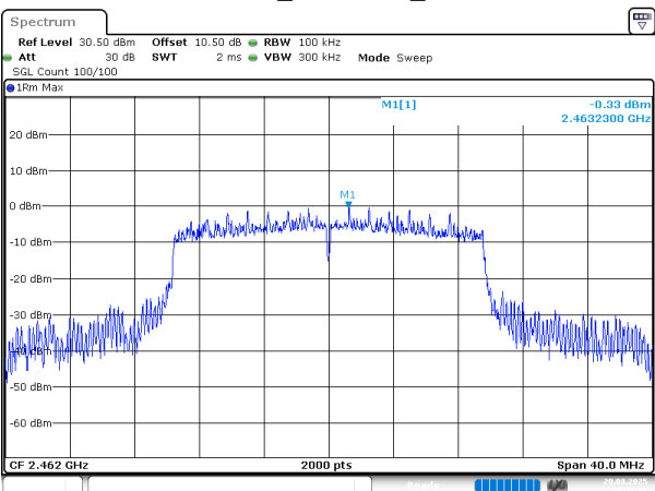
802.11ax20_2462MHz_Chain 1
