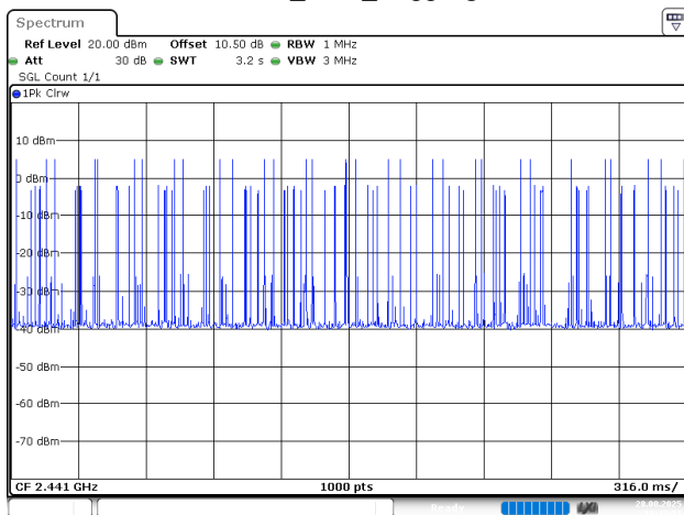
3EDR_DH1_Hopping
