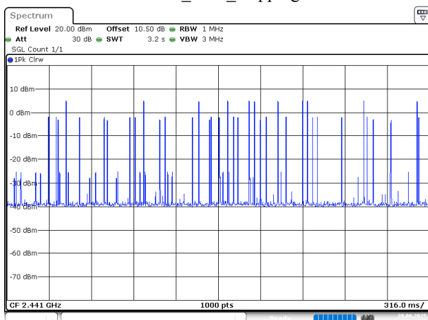
3EDR_DH5_Hopping
