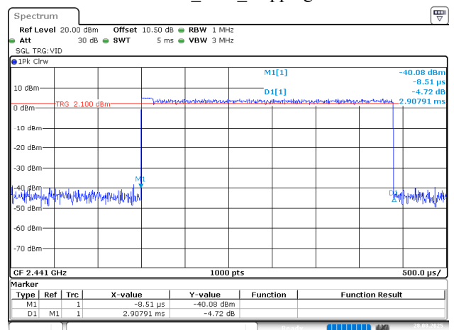
3EDR_DH5_Hopping
