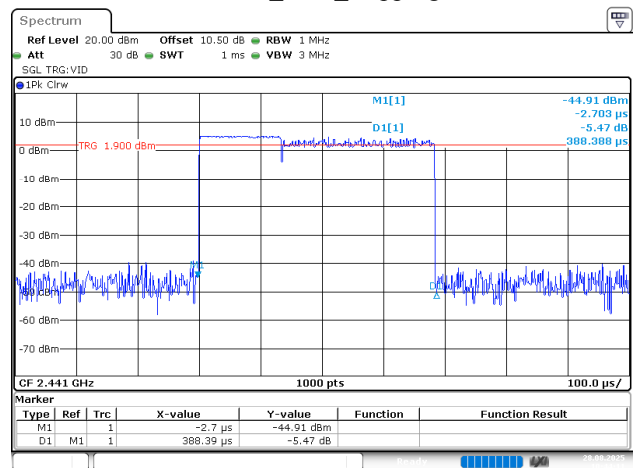
3EDR_DH1_Hopping
